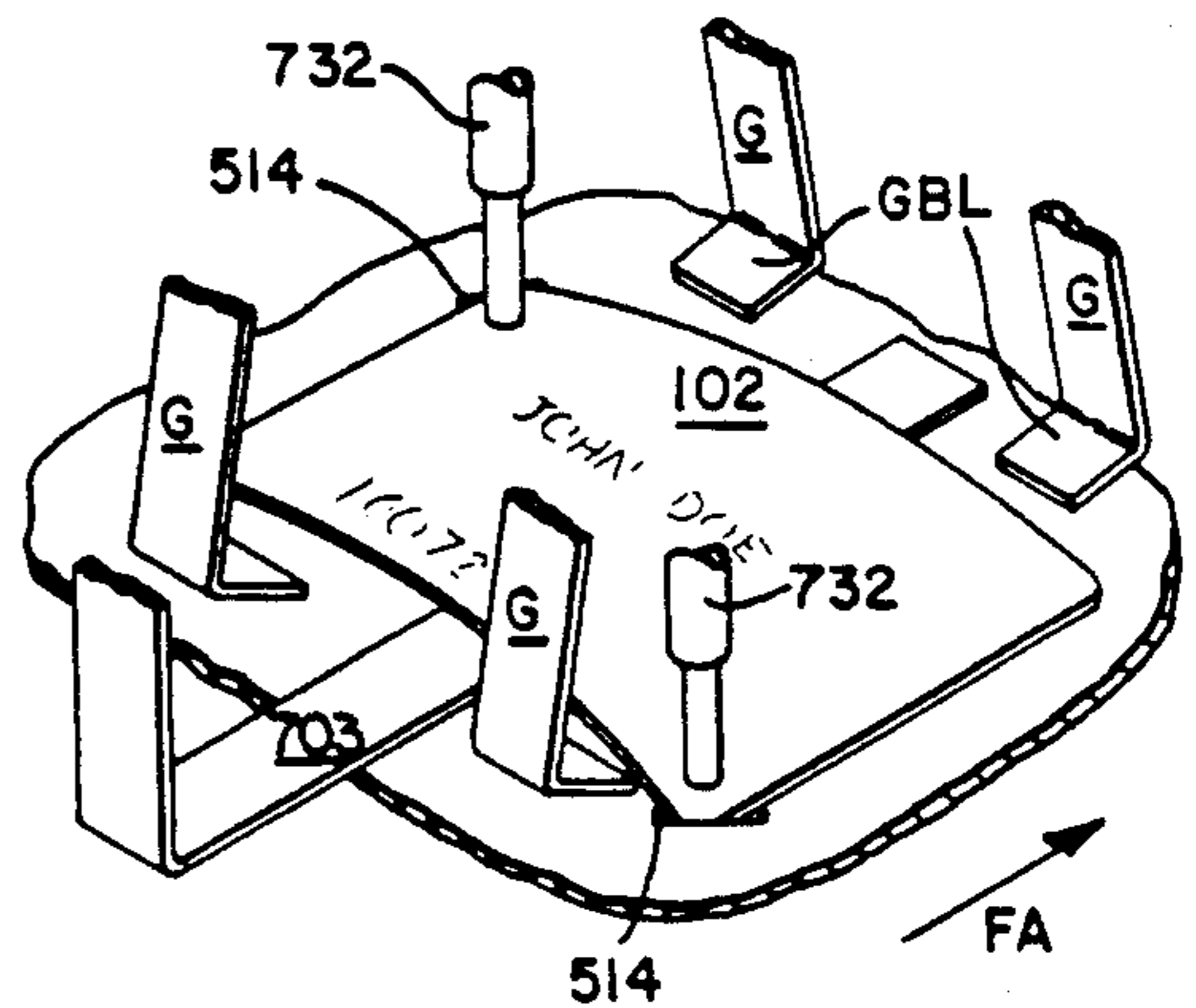
FIG. 17B.
