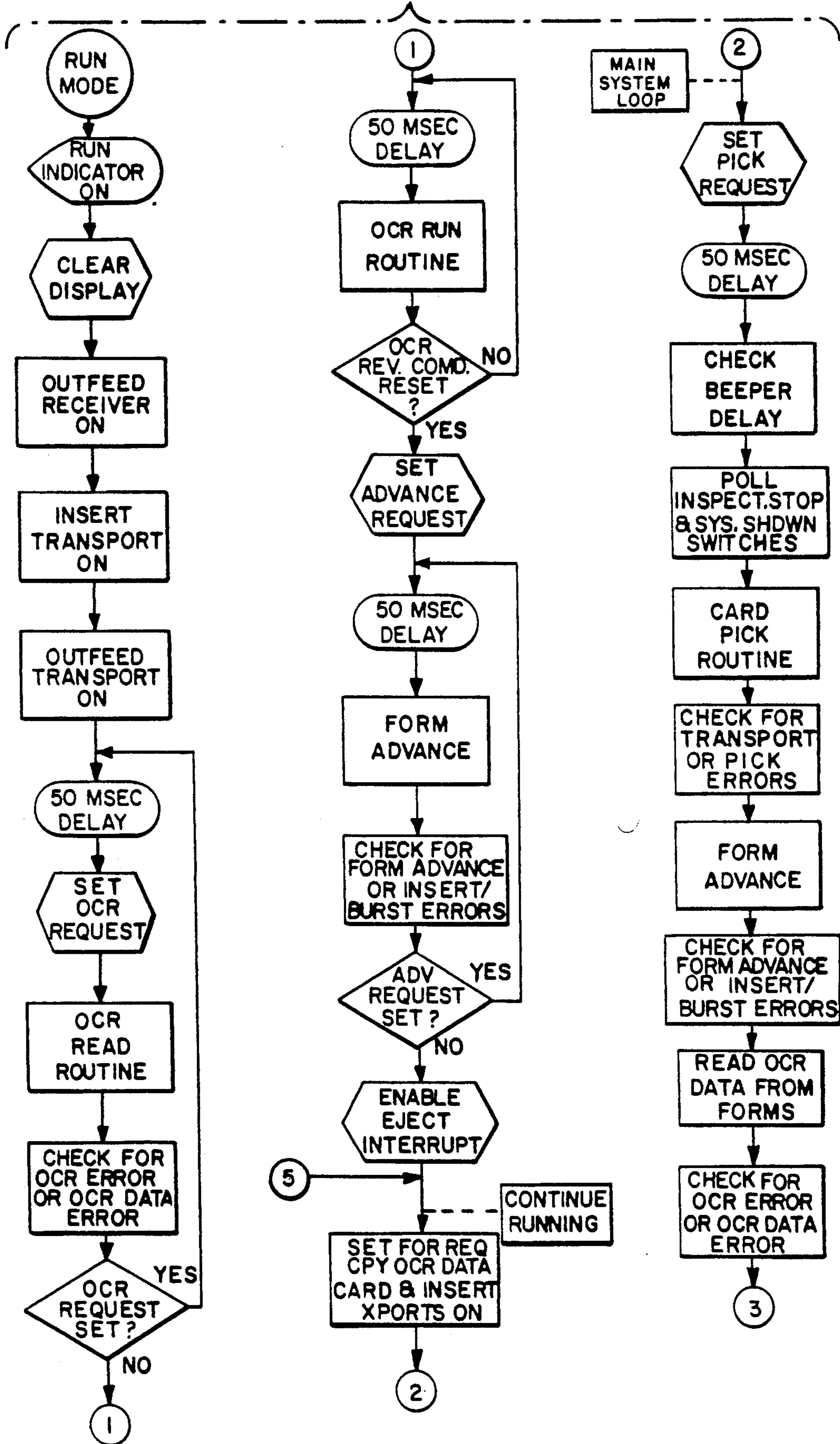
FIG. 60A.
