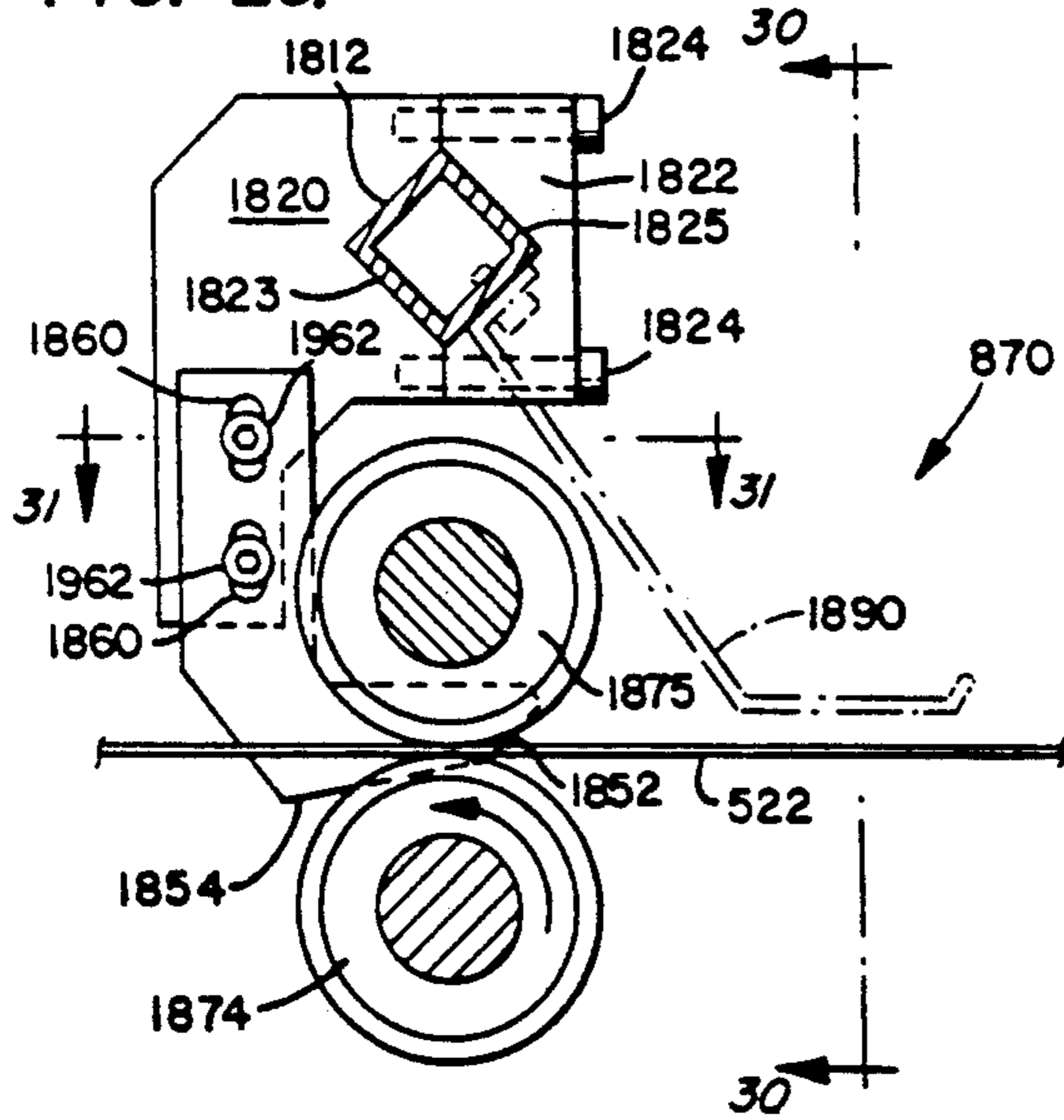
FIG. 29.
