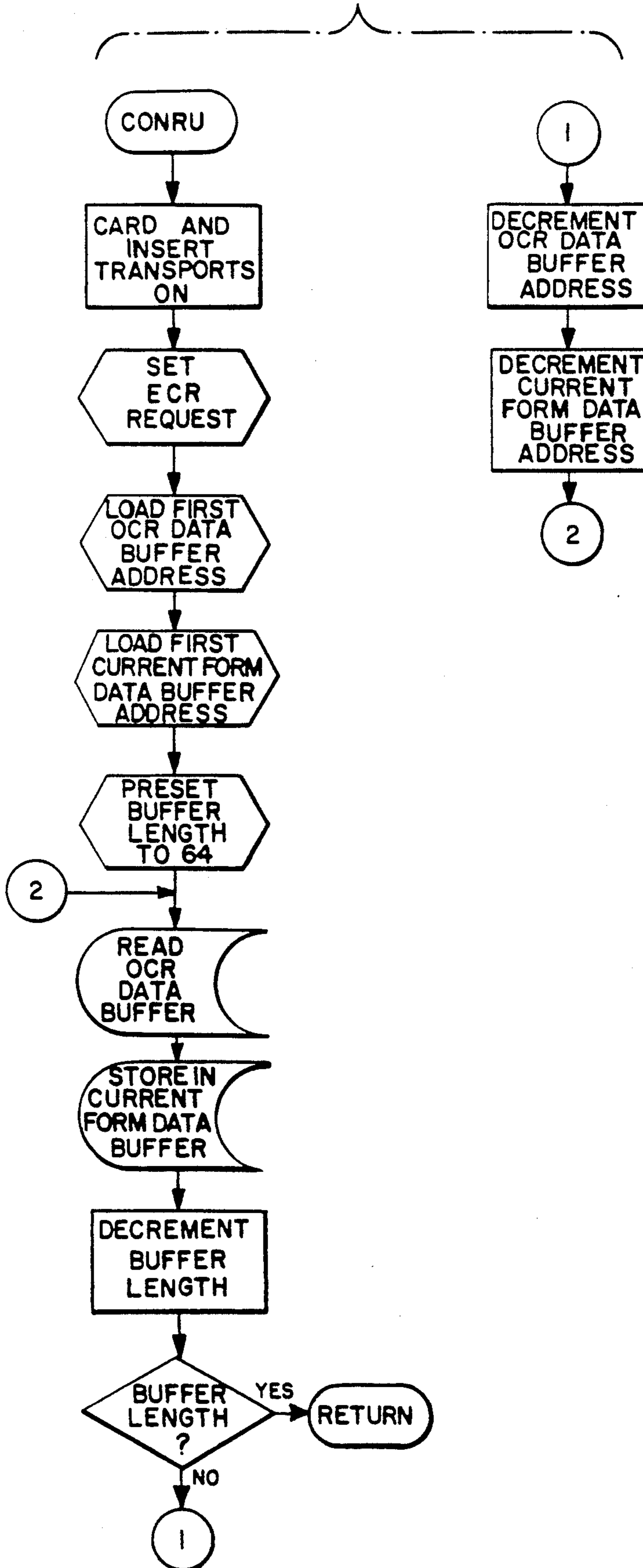
FIG. 60C.
