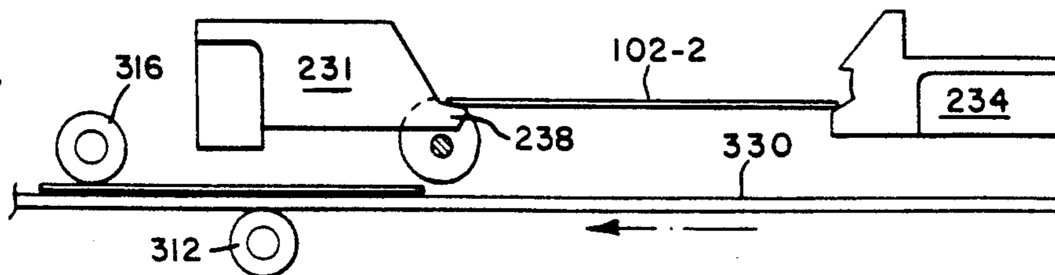
FIG. 5D.
