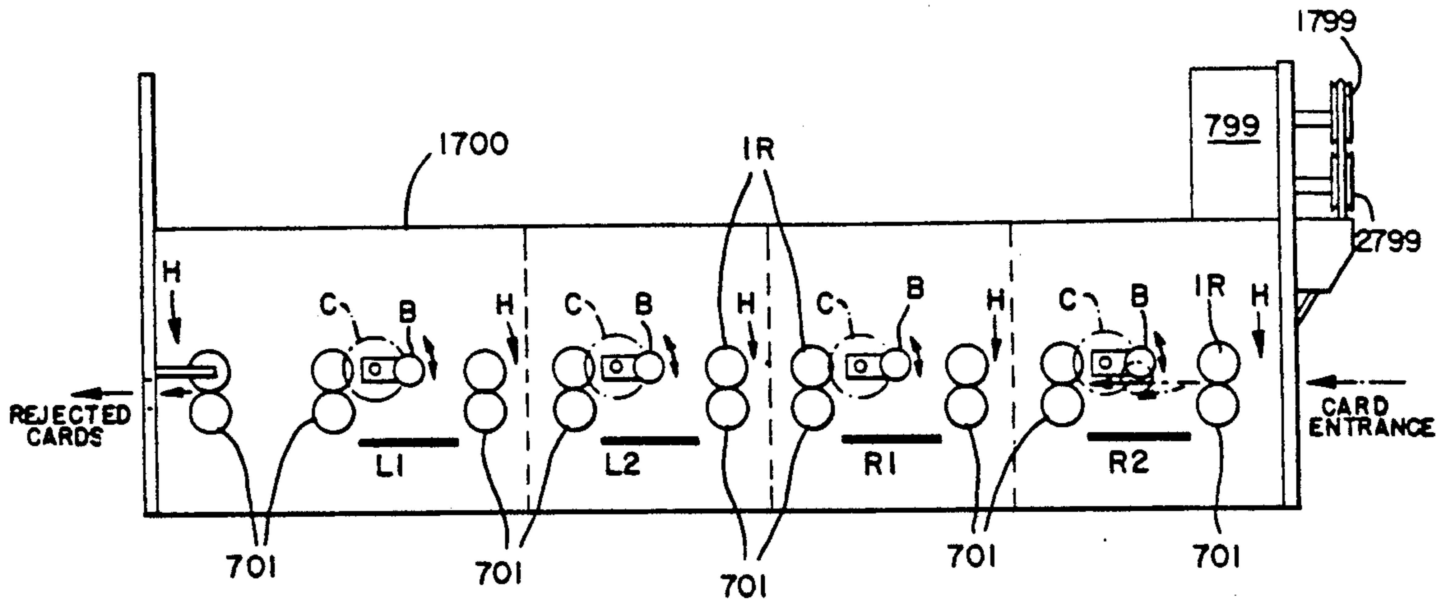
FIG. 15.
