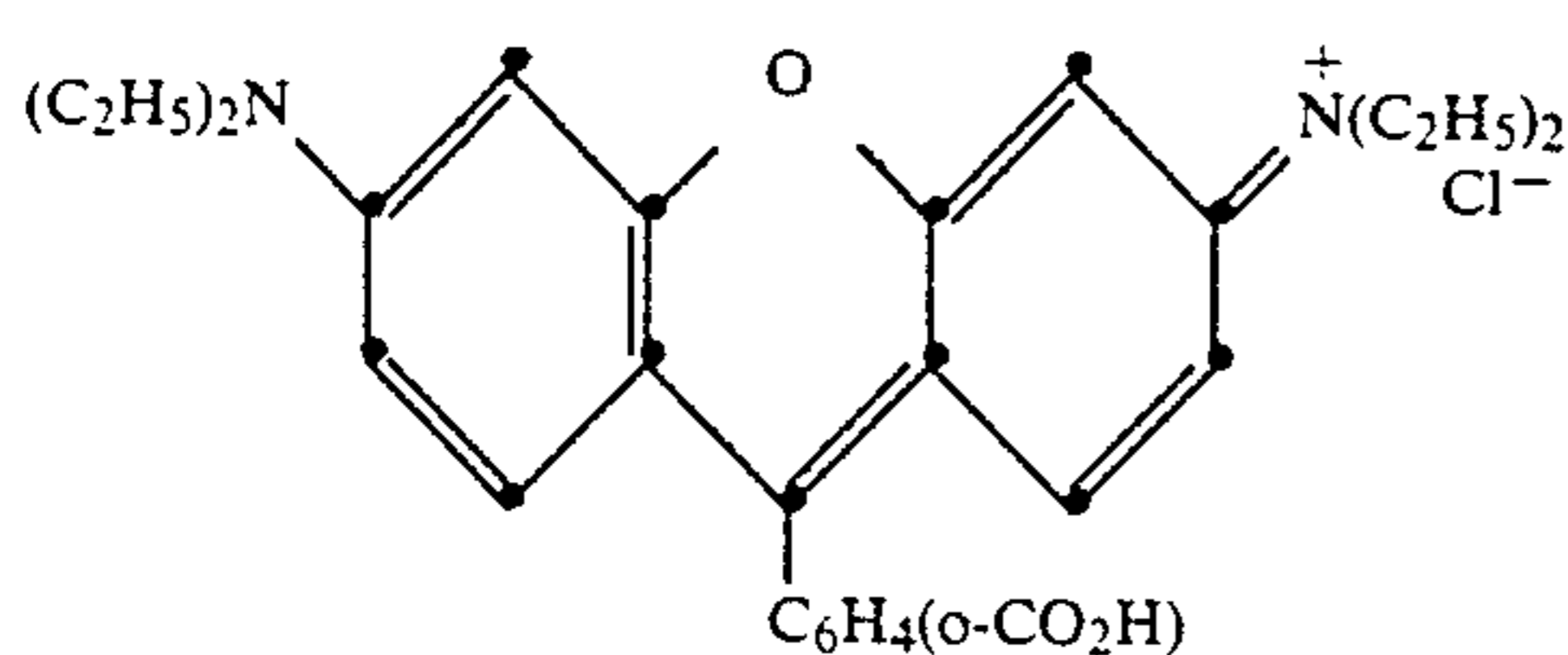
Rhodamine B
