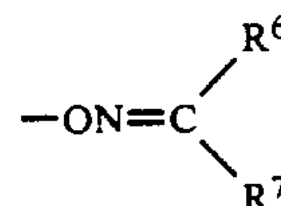
Oxime
