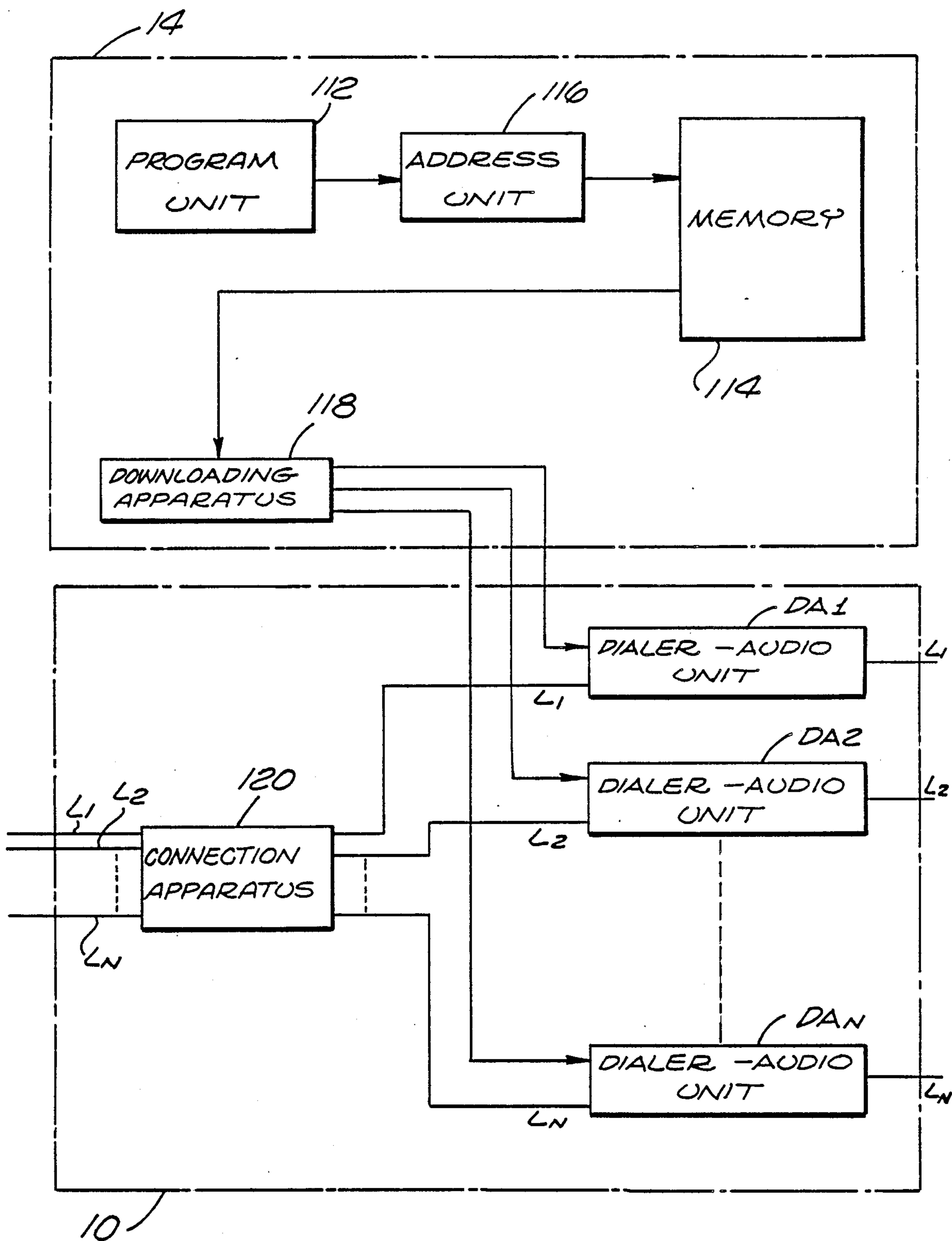
FIG. 4
