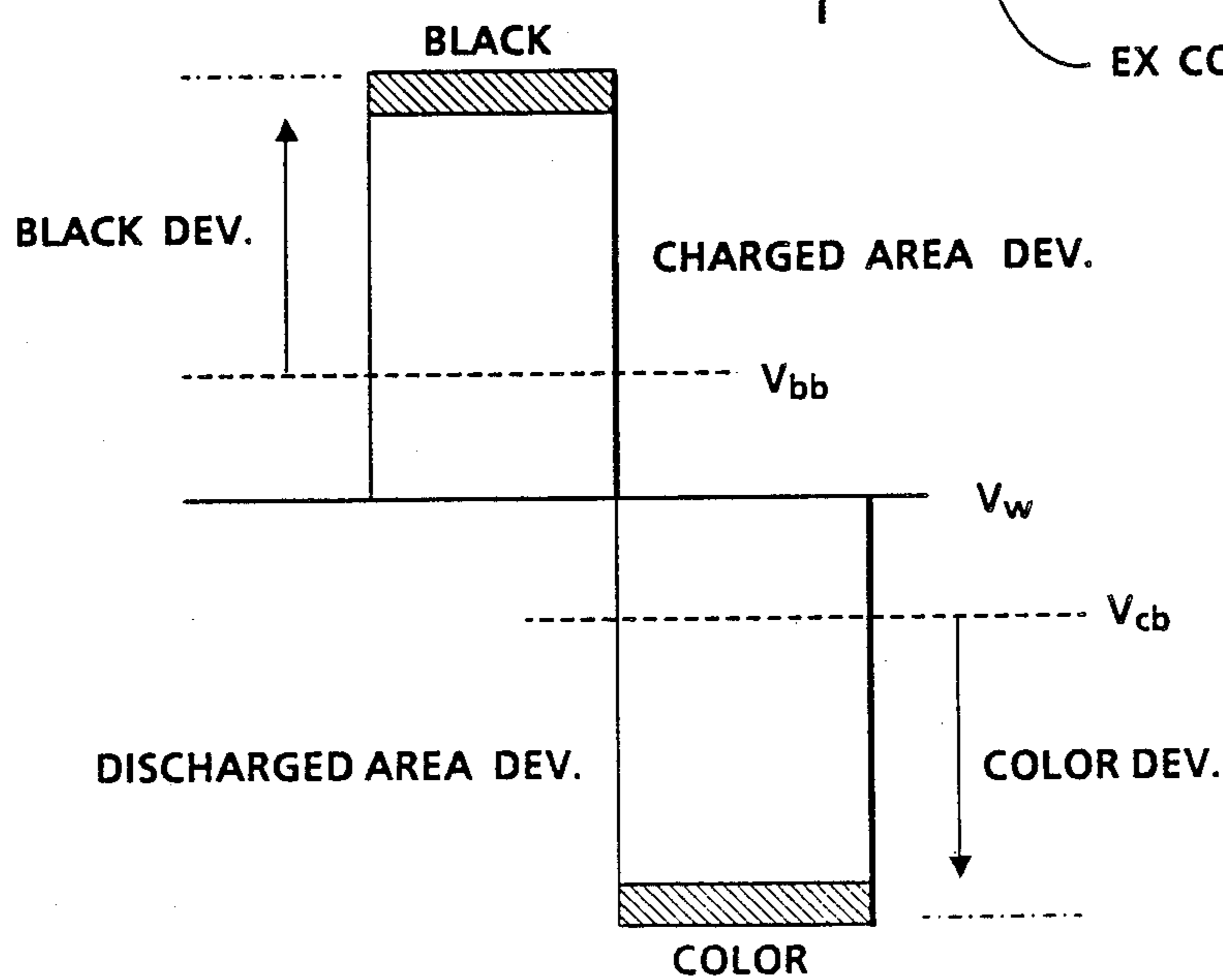
FIG. 1b
