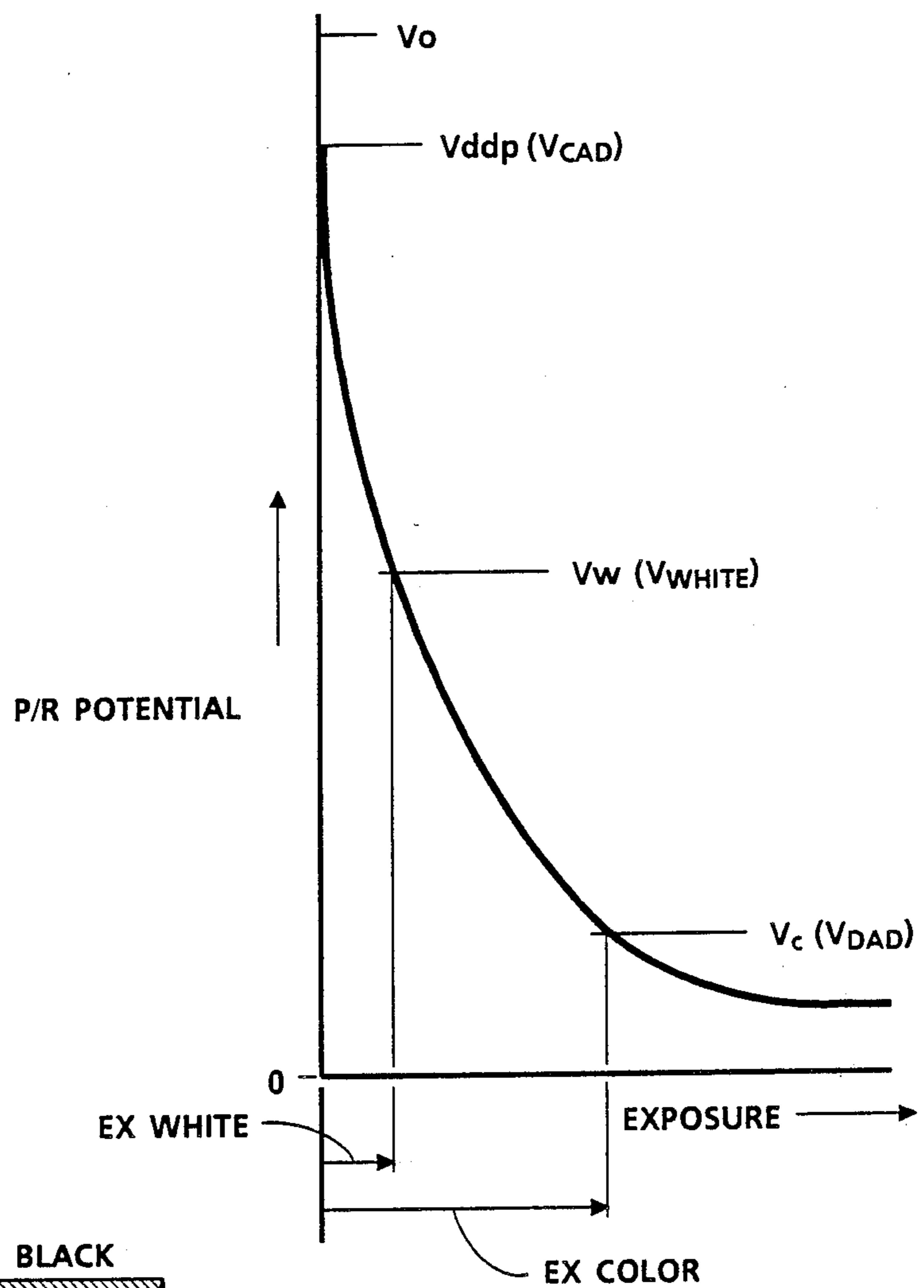
FIG. 1a
