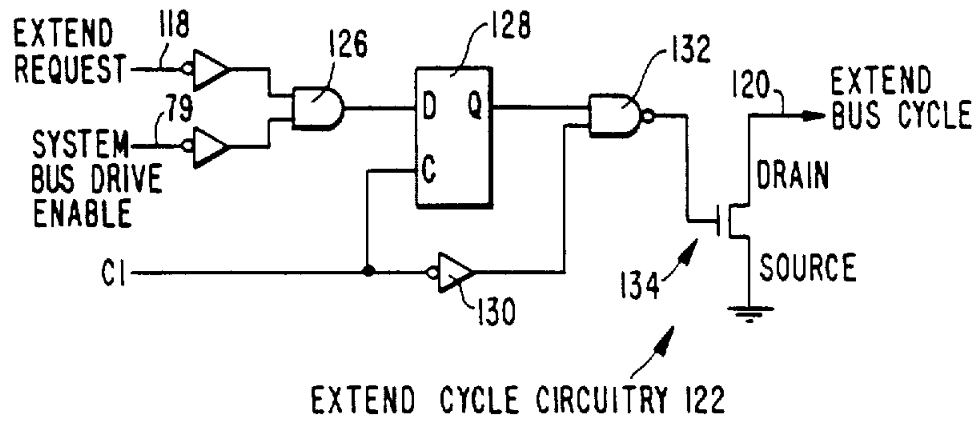
FIG. 7.
