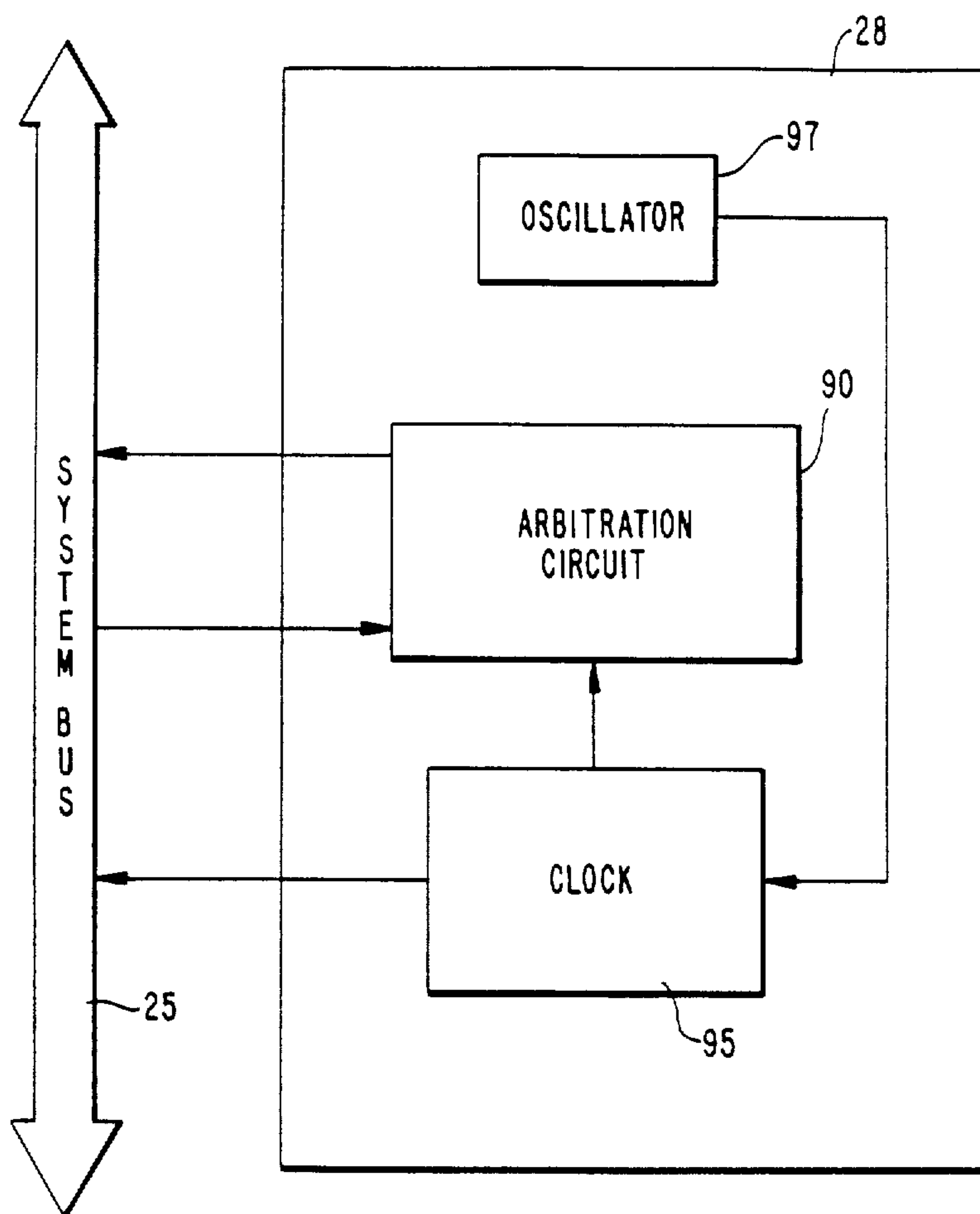
FIG. 5
