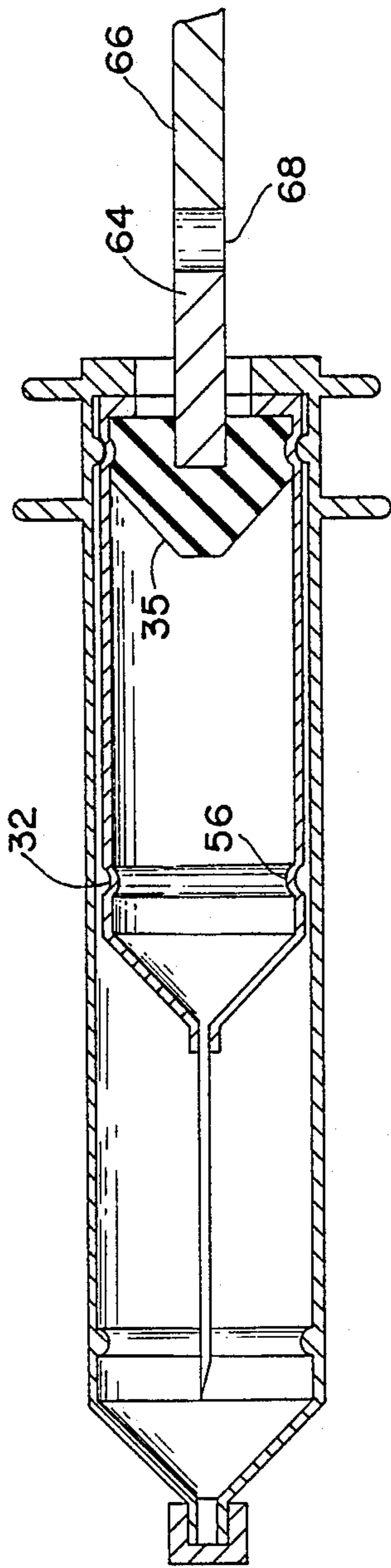
FIG. 8
