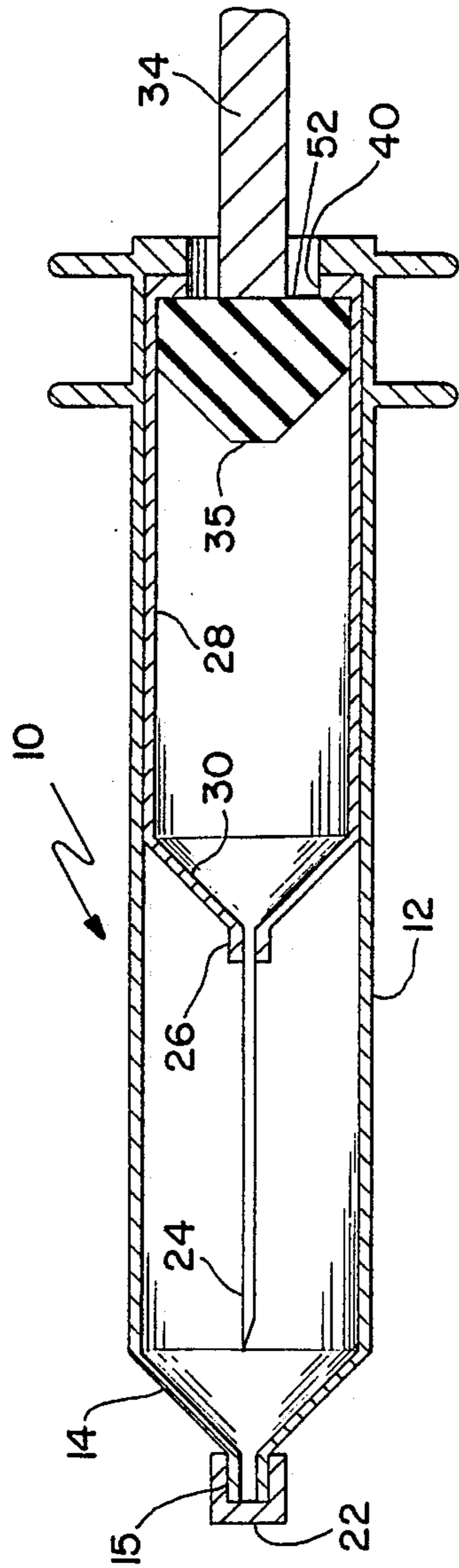
FIG. 1
