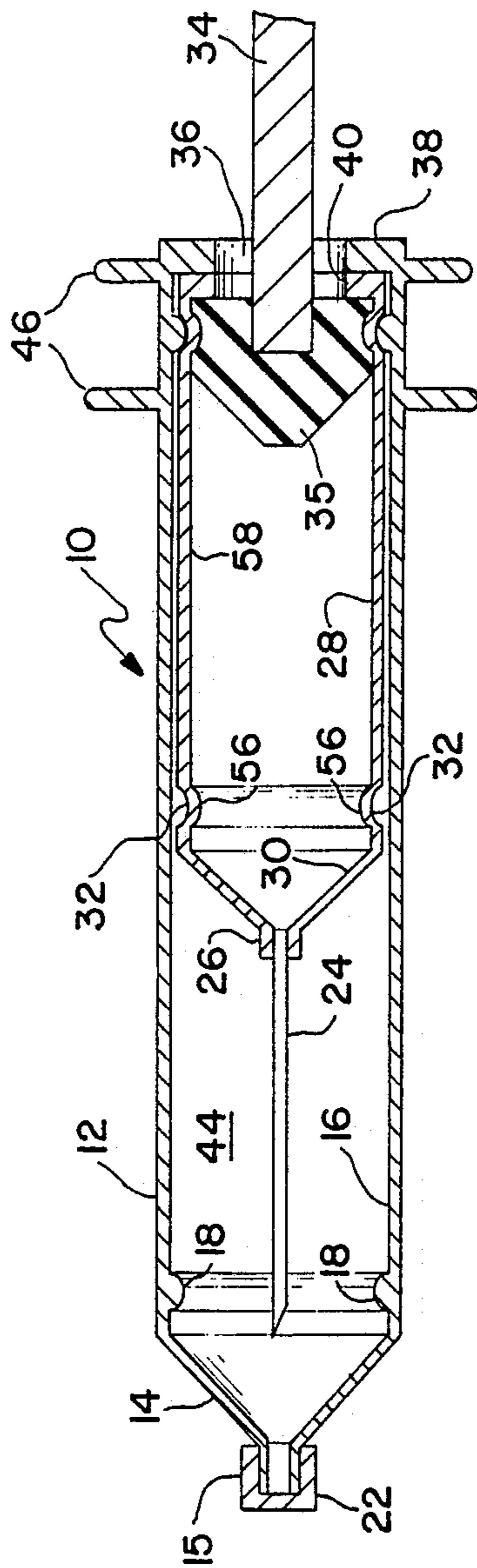
FIG. 5
