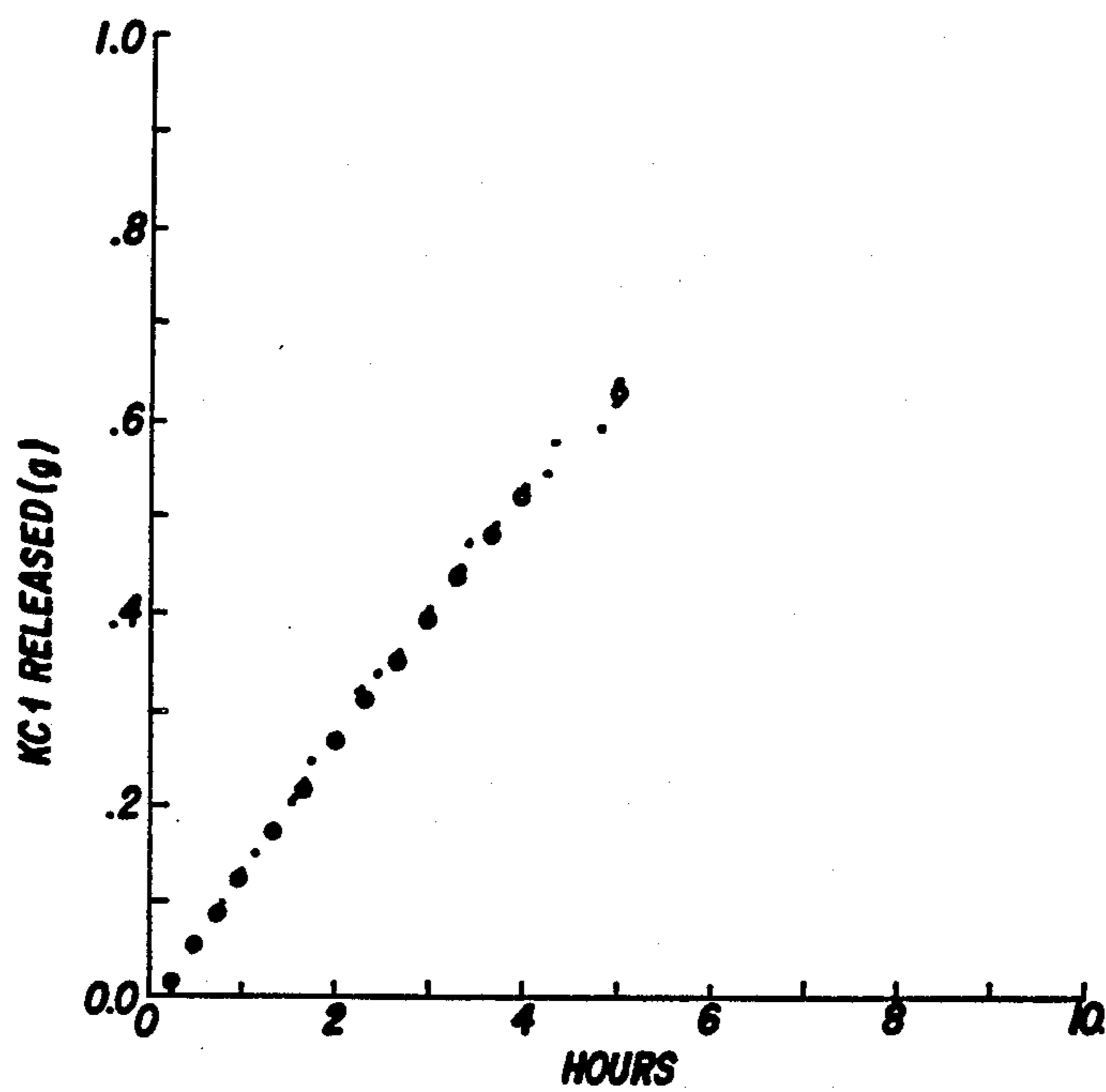
FIG. 3C NMP-50
