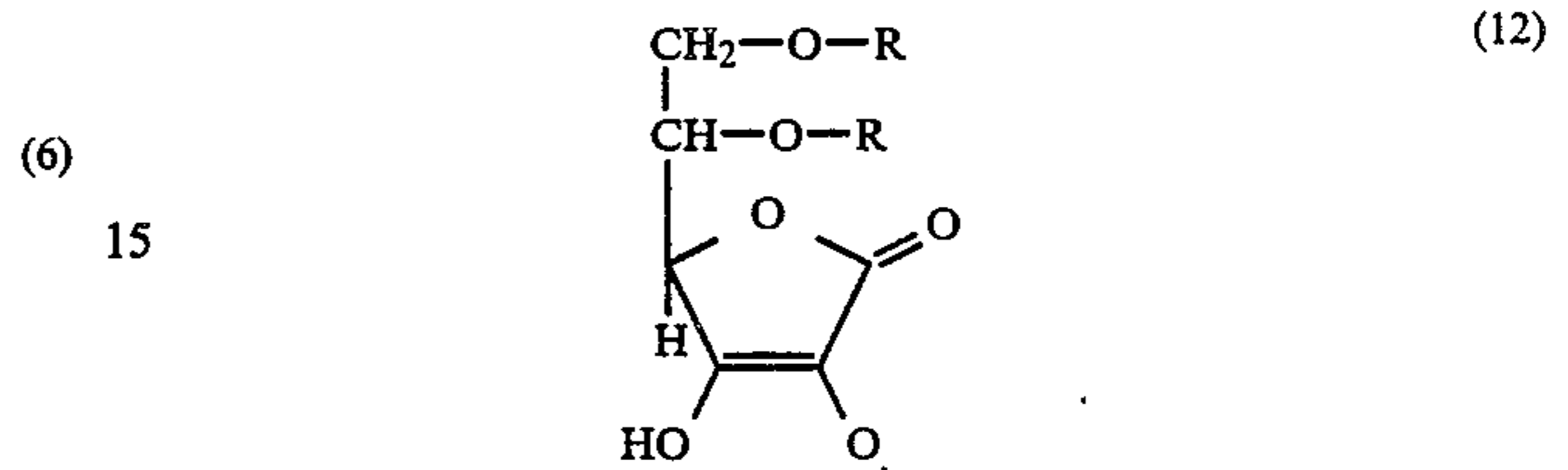
2,5,6 tri-ester
