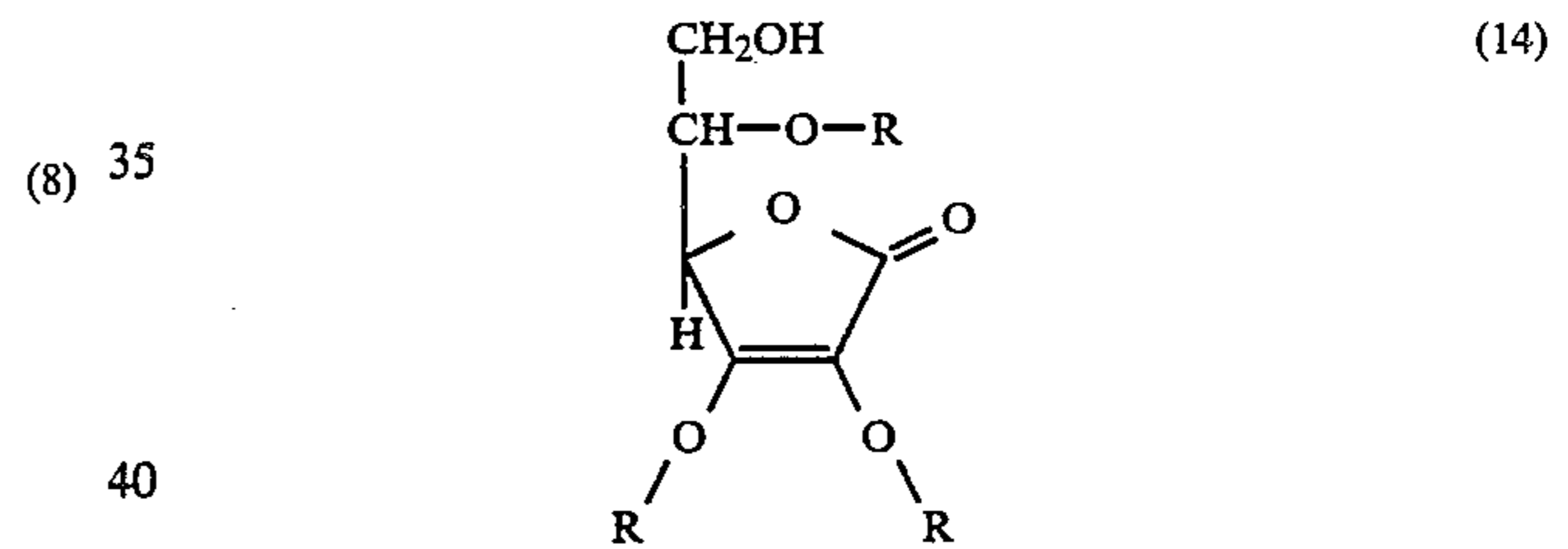
2,3,5 tri-ester
