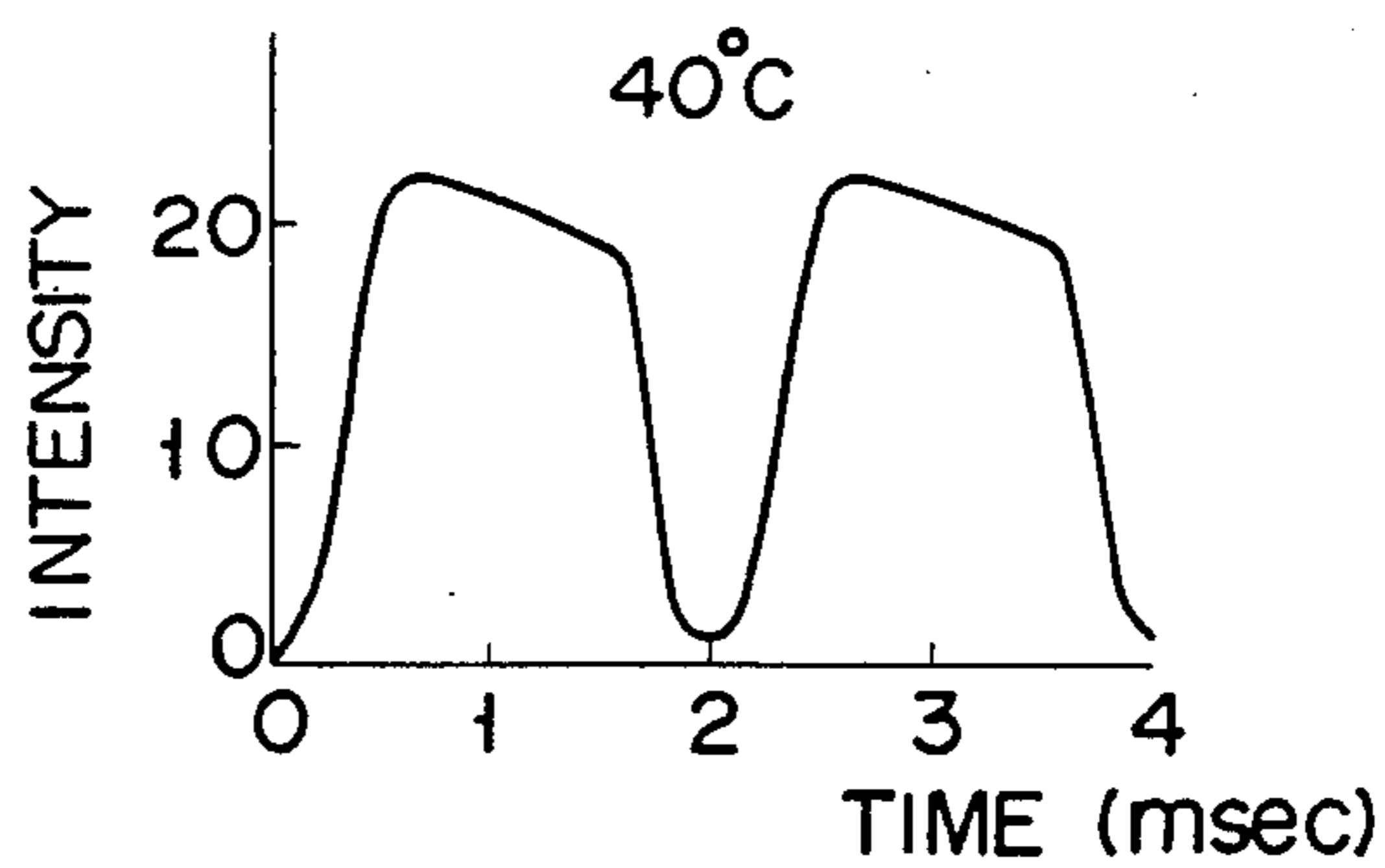
FIG. 48D
