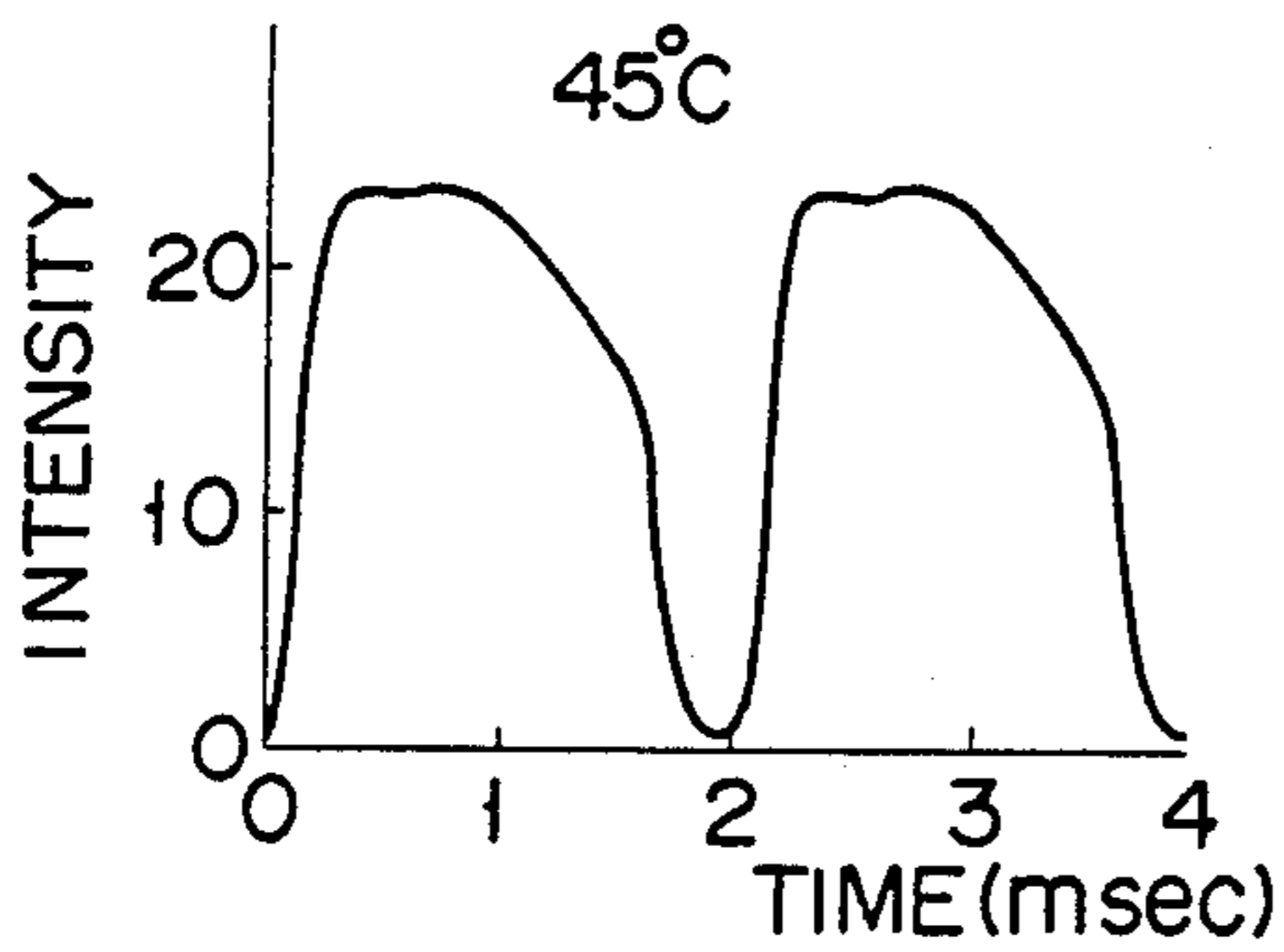
FIG. 50C
