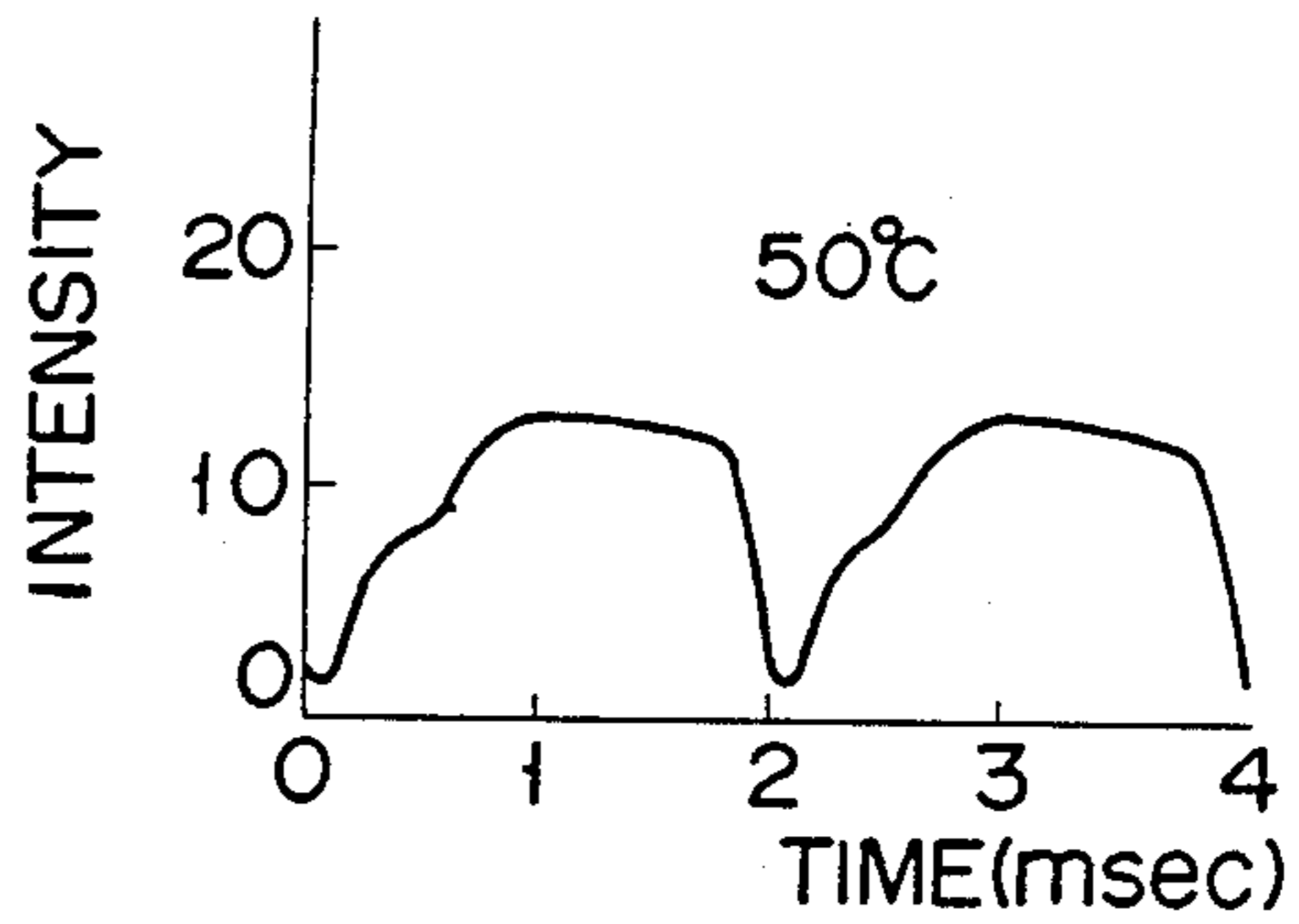
FIG. 46B
