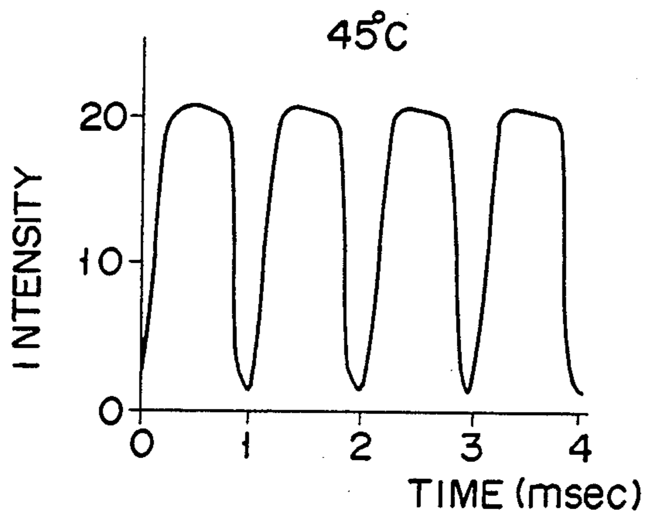
FIG. 57C
