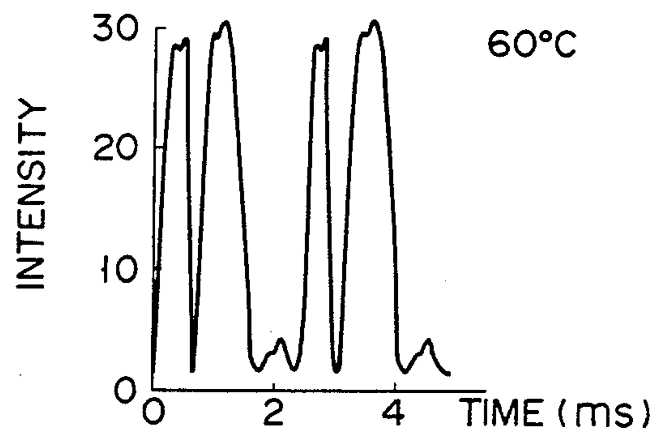
FIG. 74A
