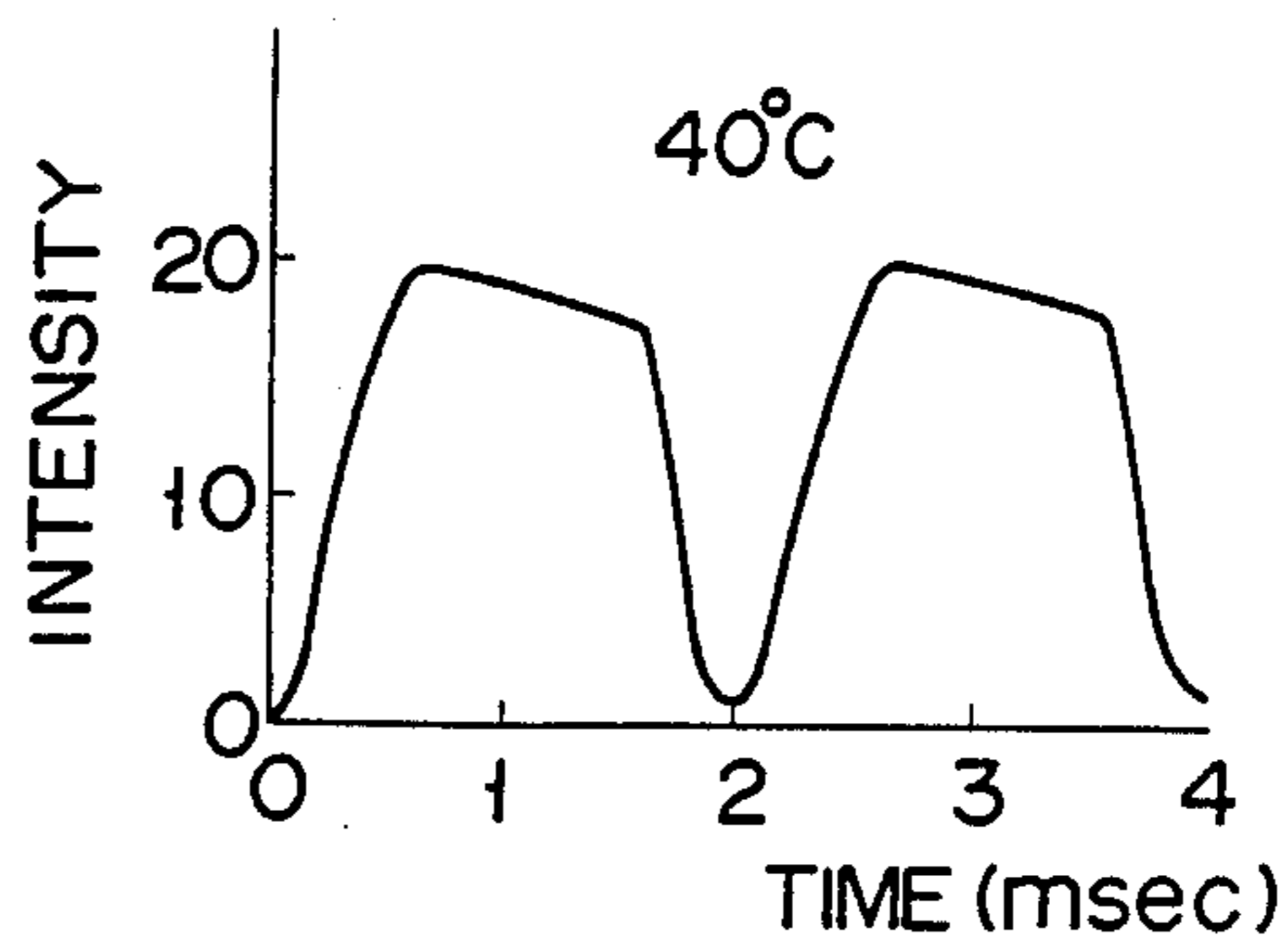
FIG. 45D
