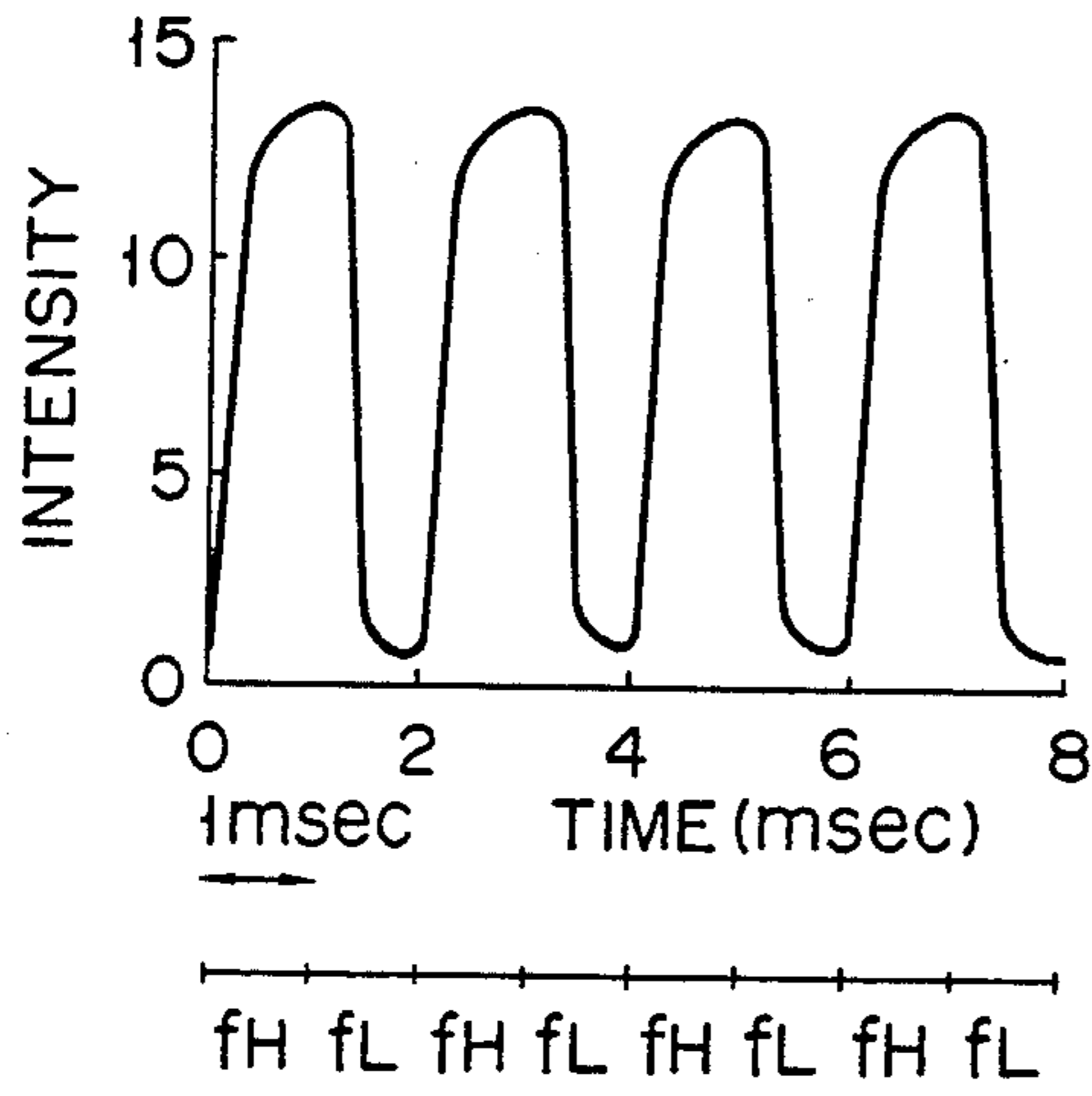
FIG. 34A
