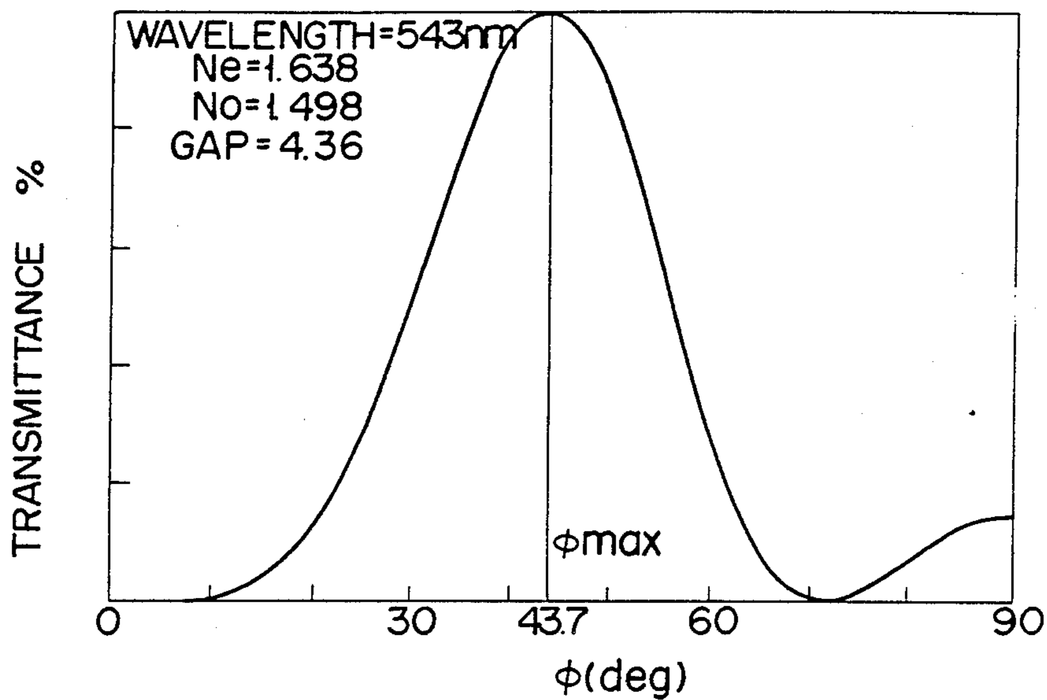
FIG. 54
