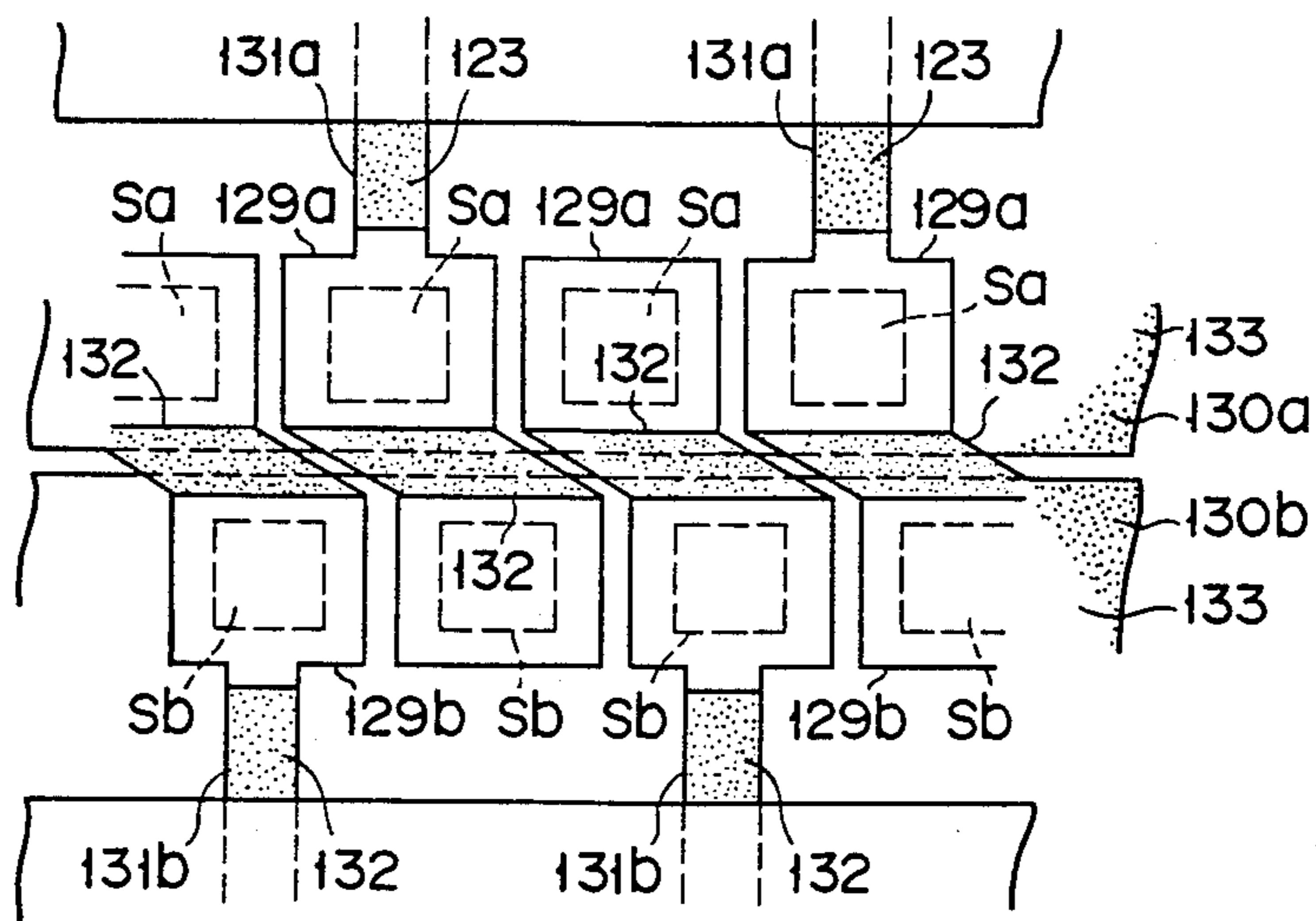
FIG. 28
