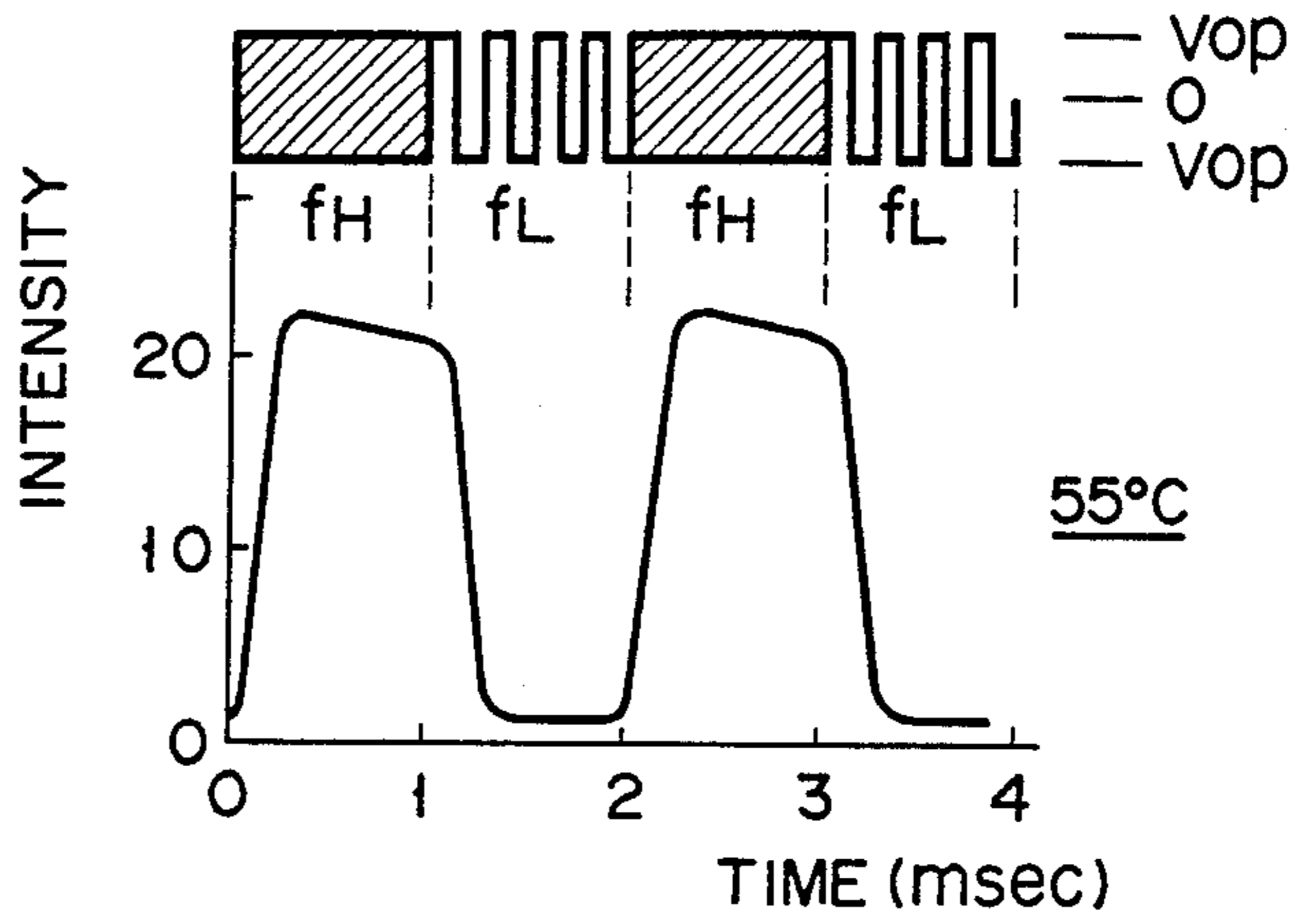
FIG. 13A
