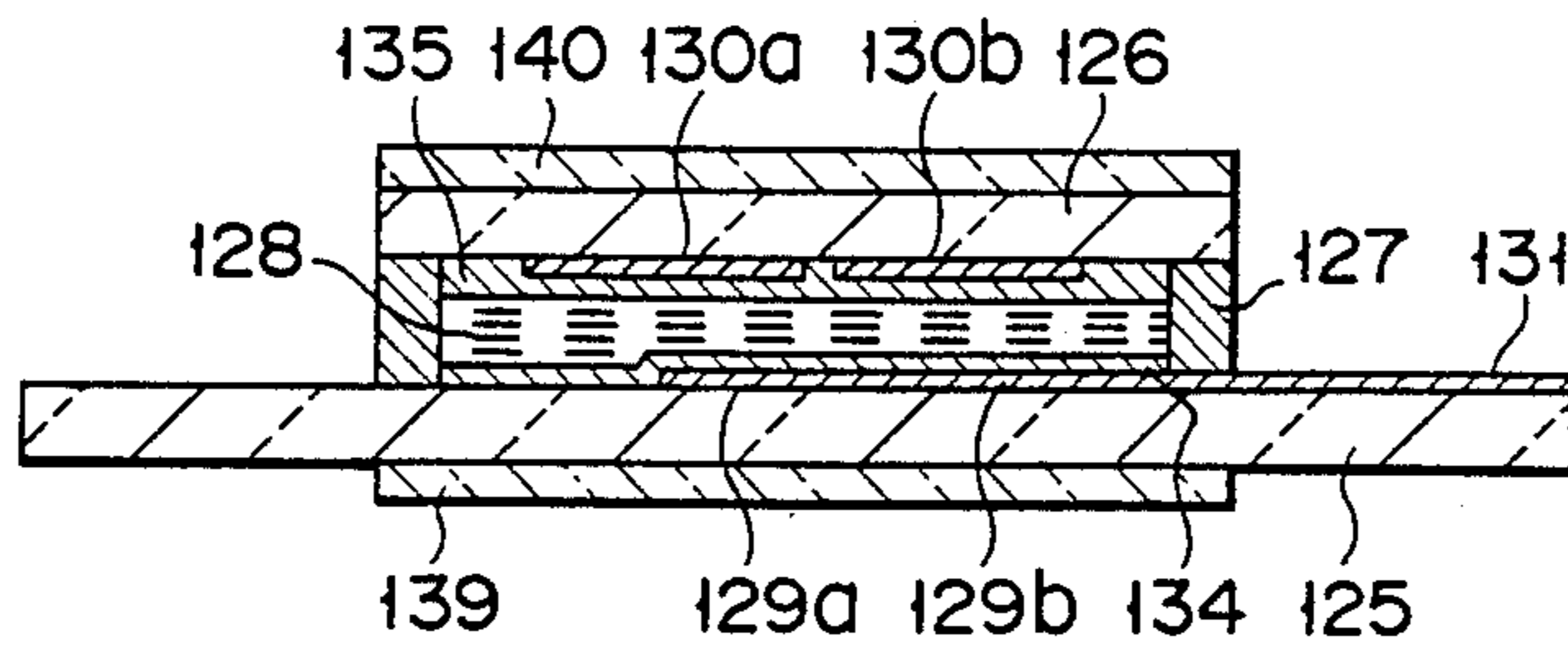
FIG. 26
