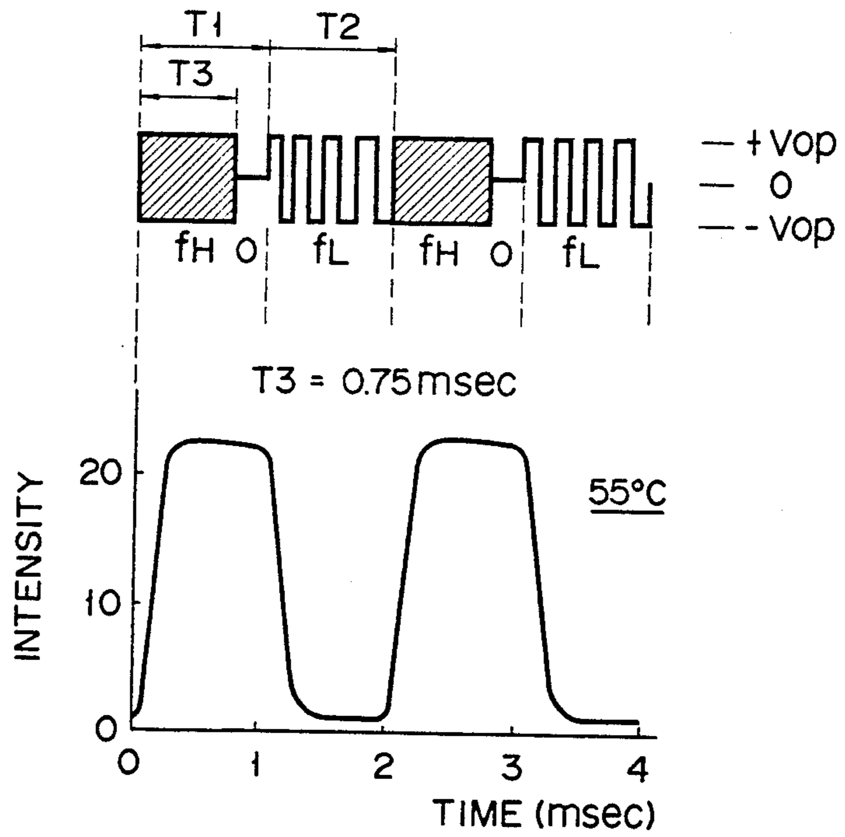
FIG. 15A
