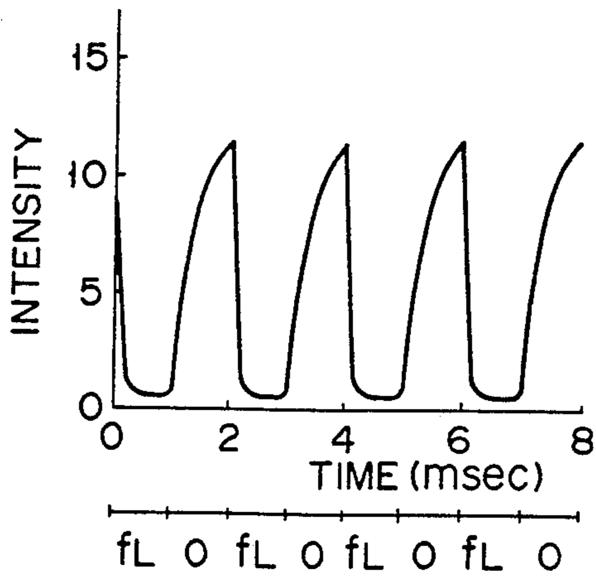
FIG. 34B
