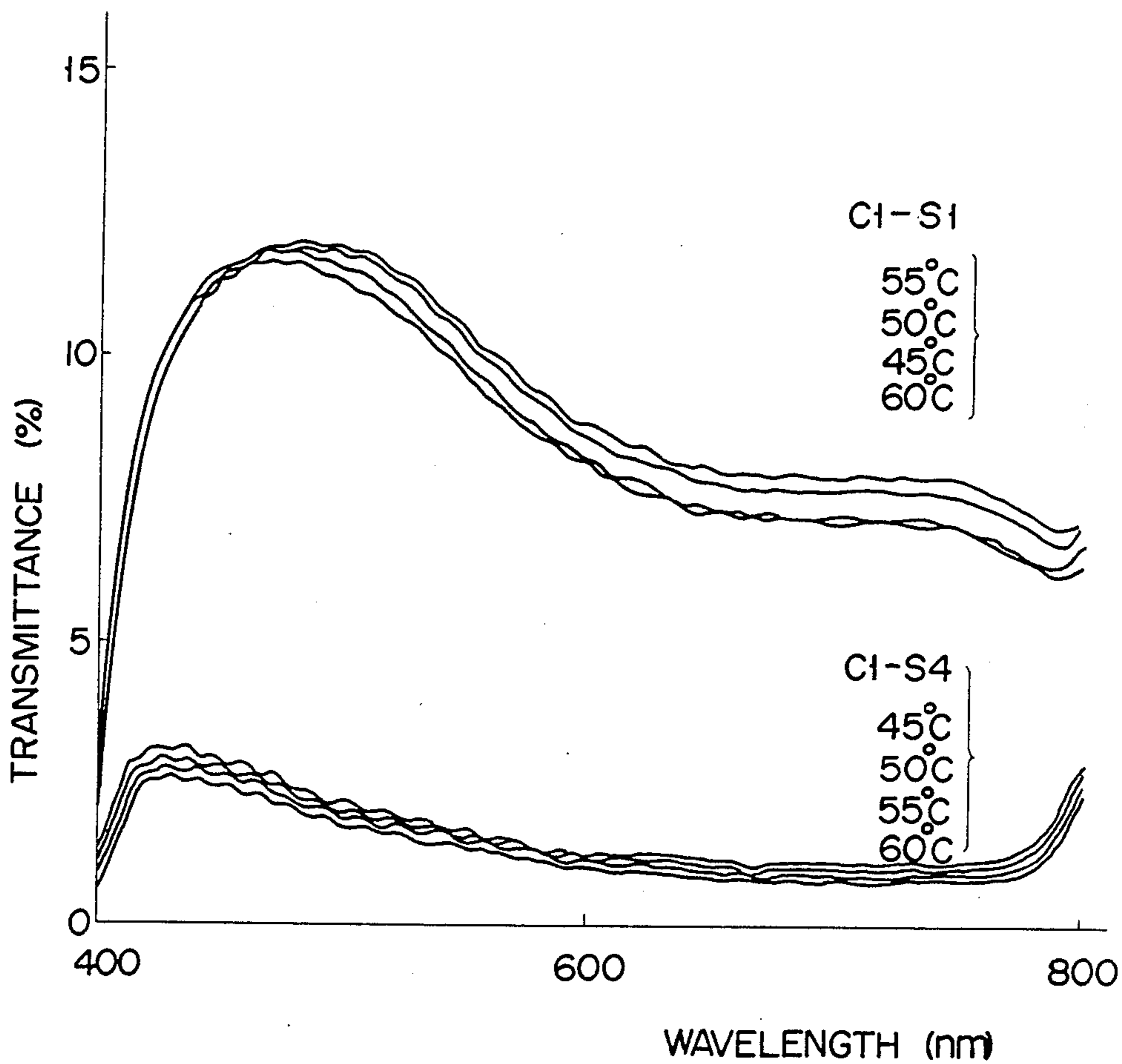
FIG. 42
