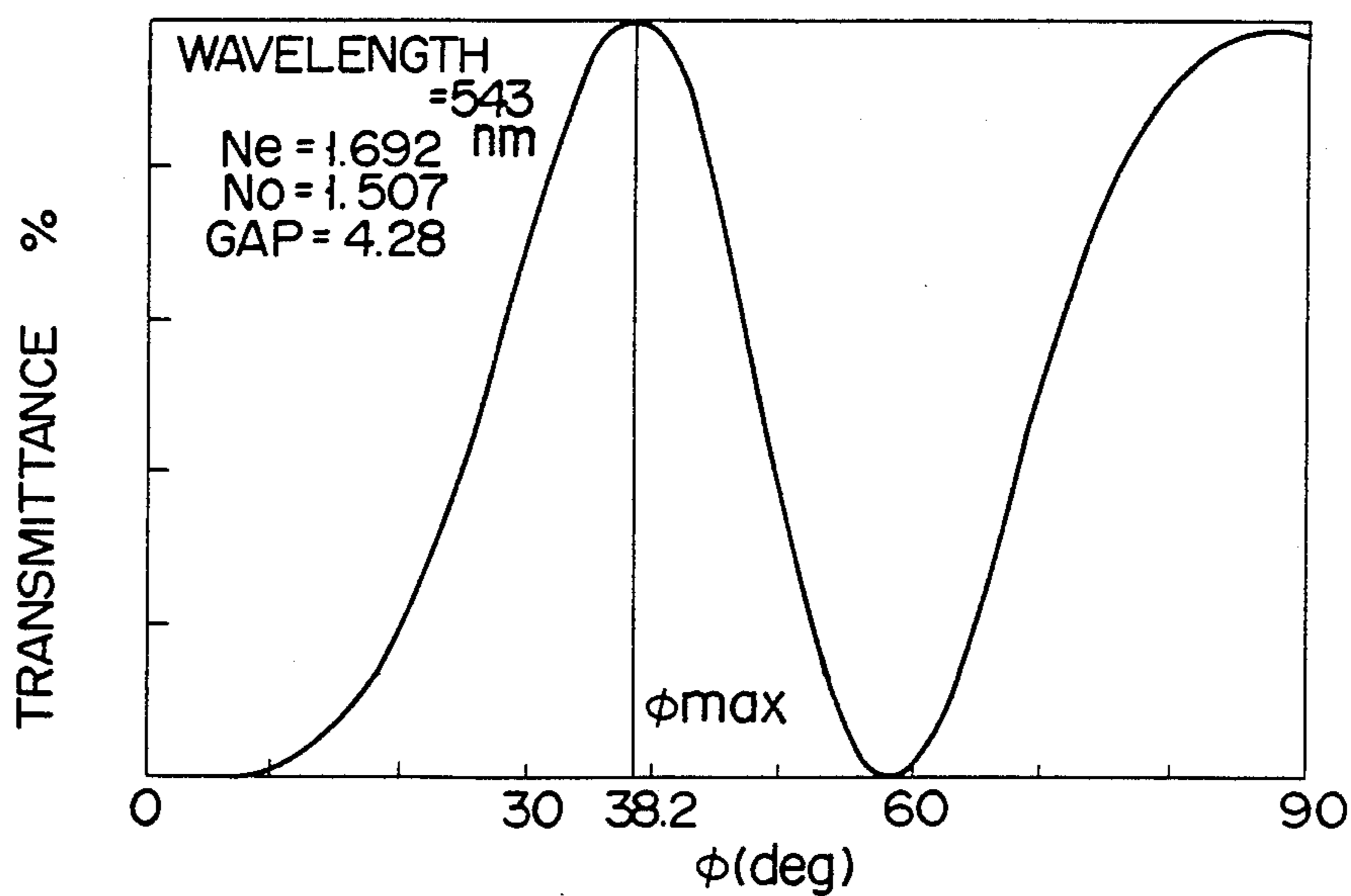
FIG. 55
