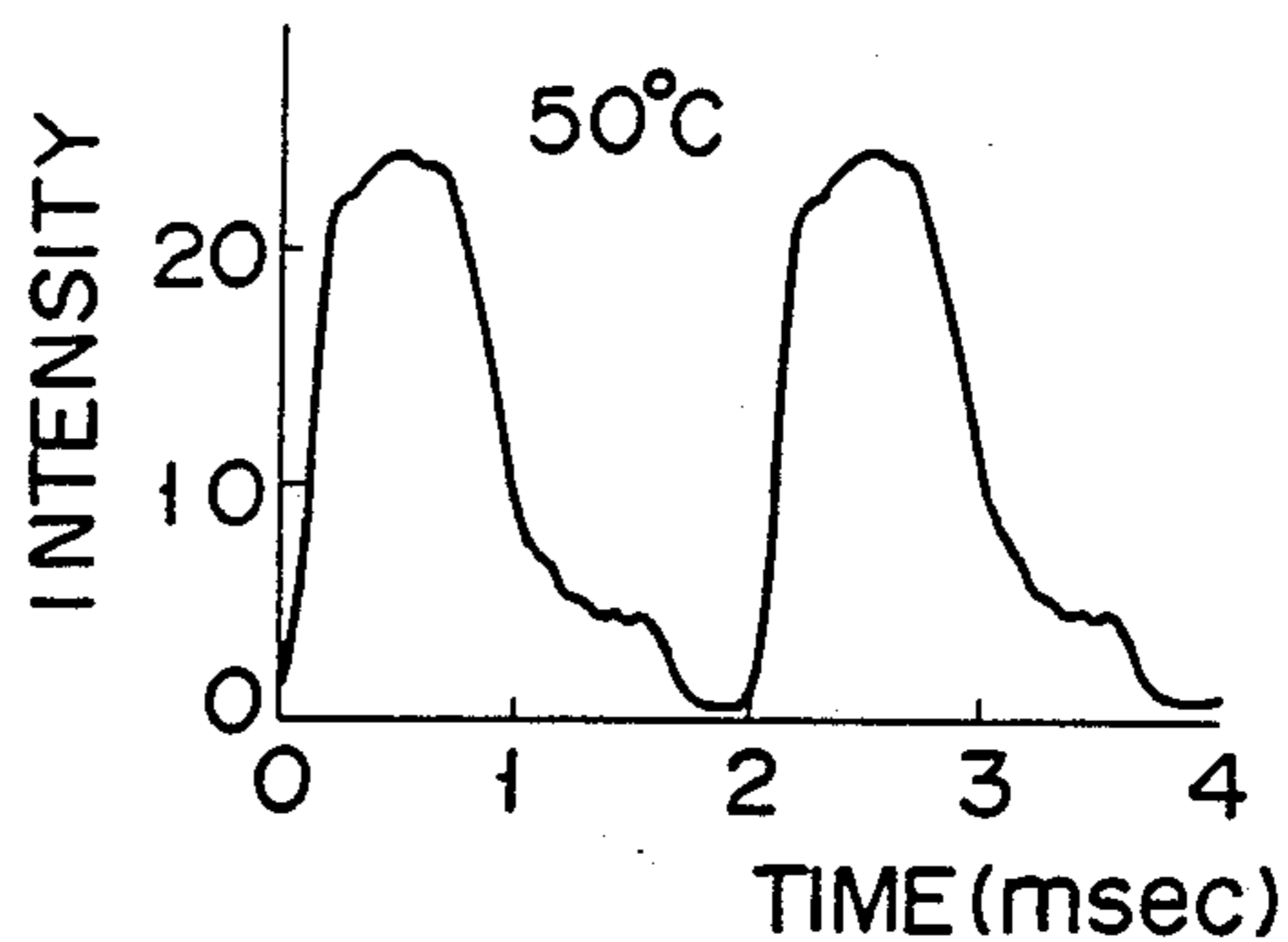
FIG. 51B
