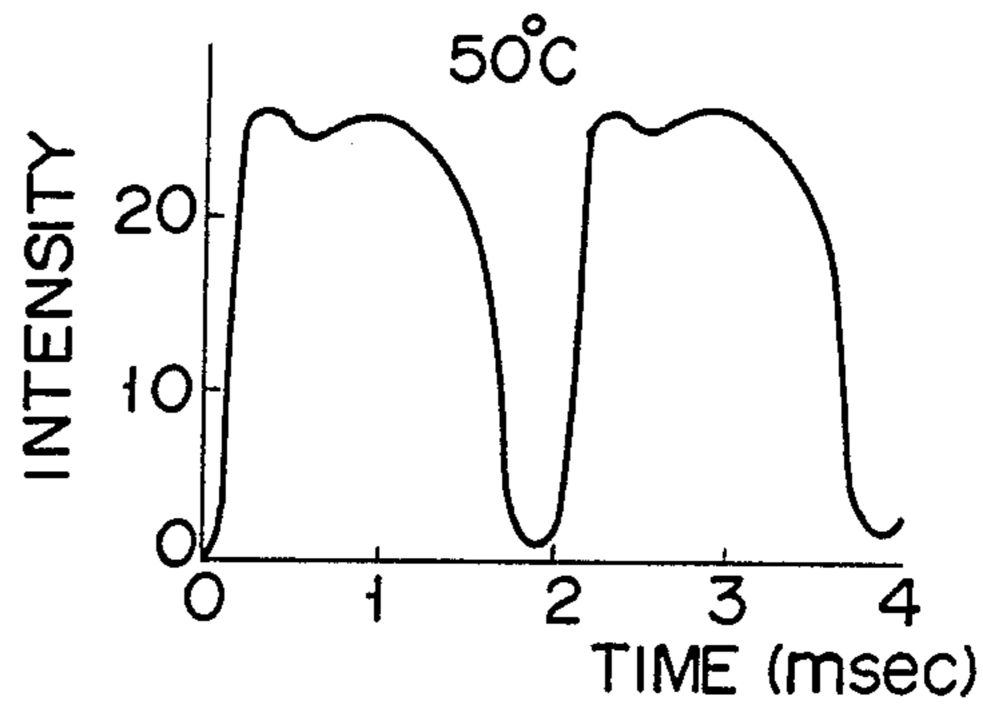
FIG. 45B
