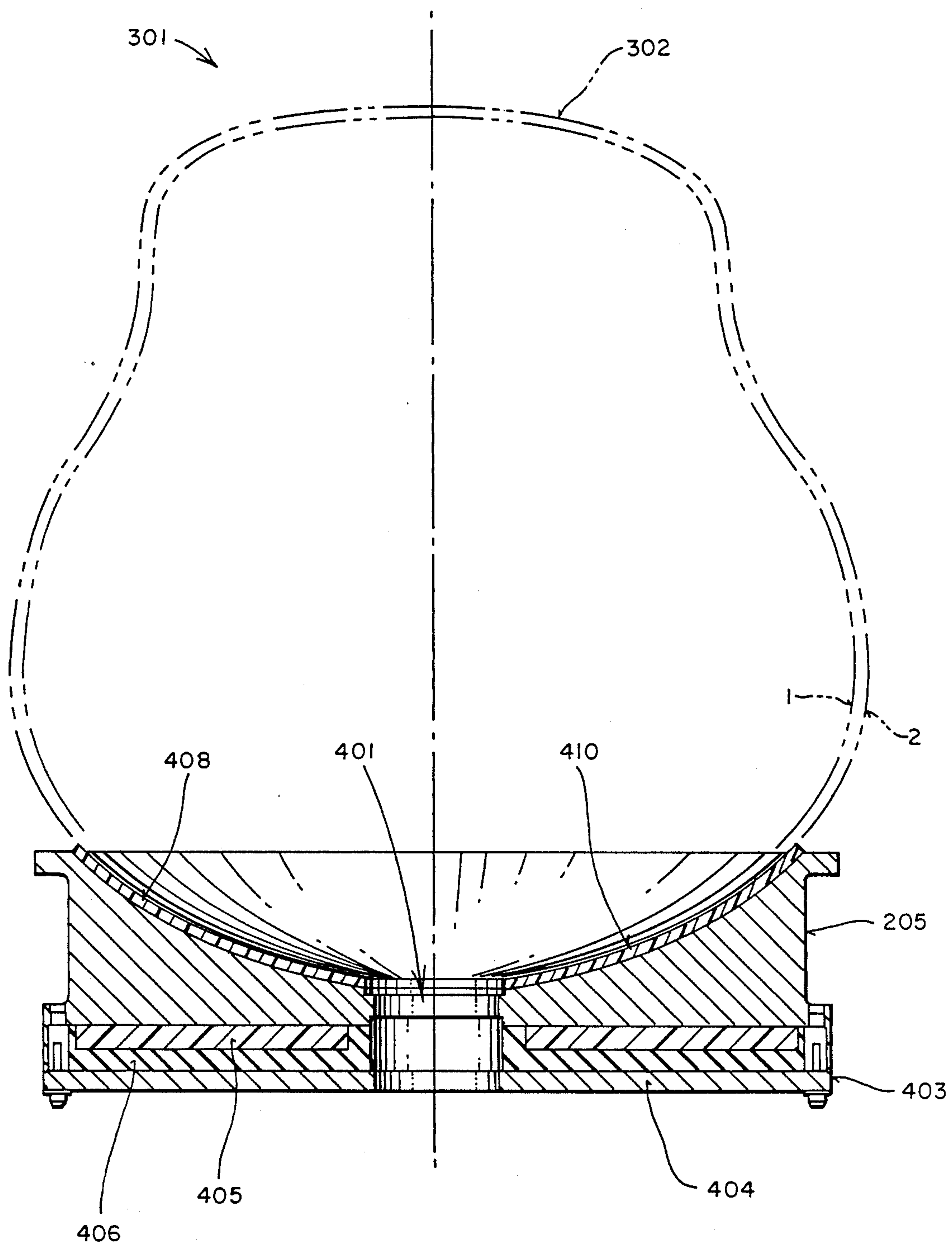
SECTION A-A
