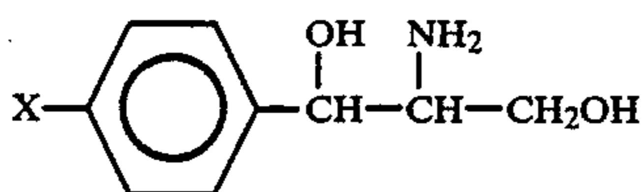
(I, threo 1S,2S)
