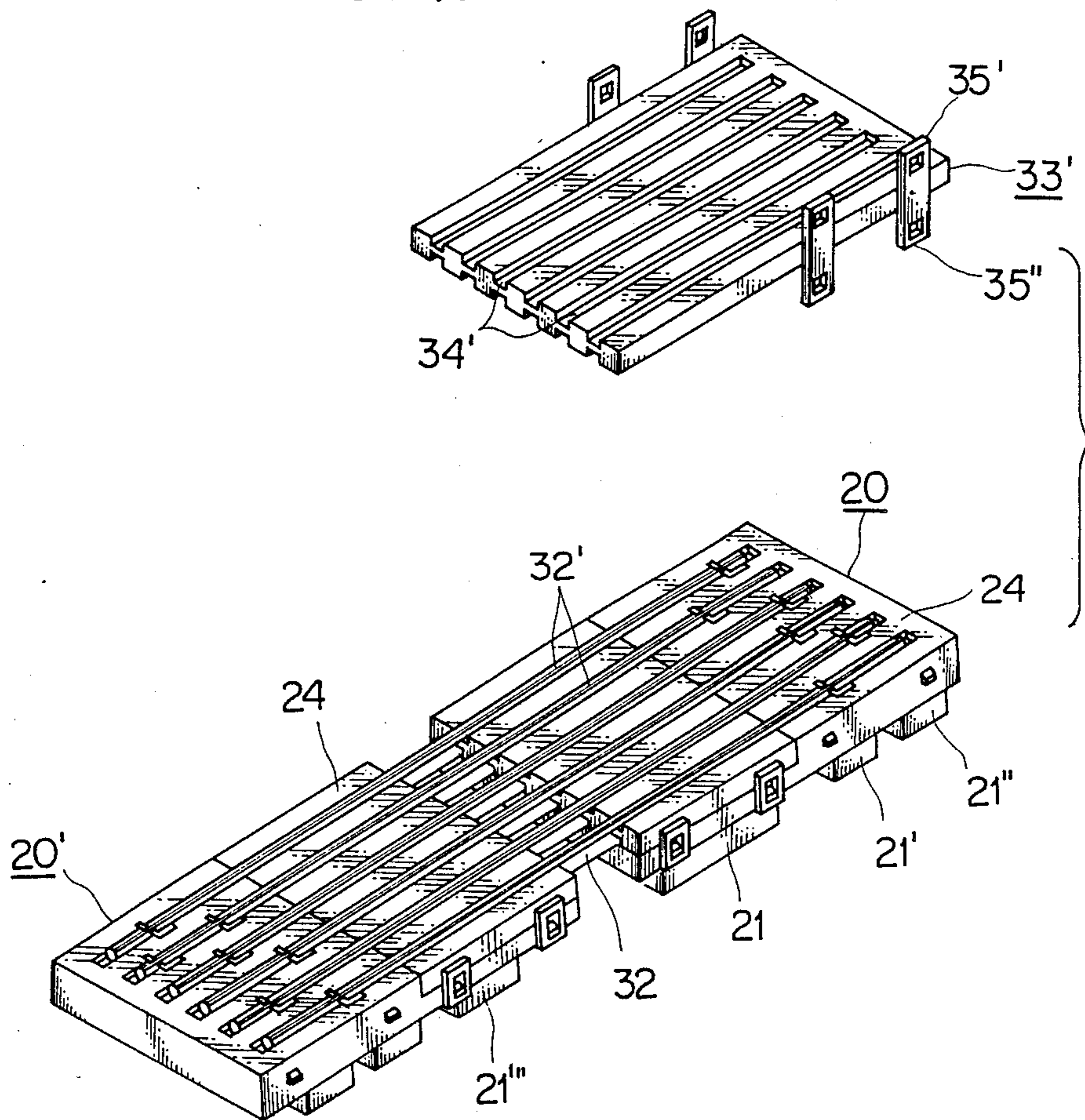
FIG. 4F
