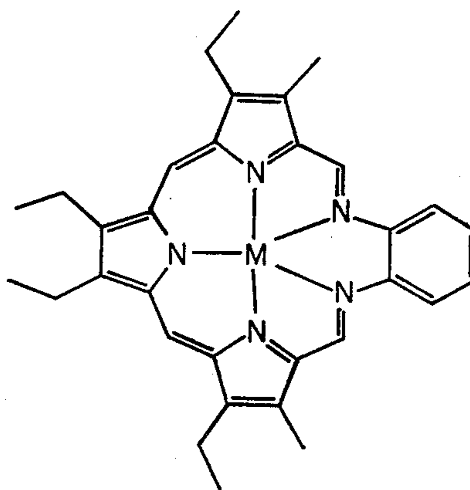
2A. M = H, n = 0 3A. M = Cd, n = 1
