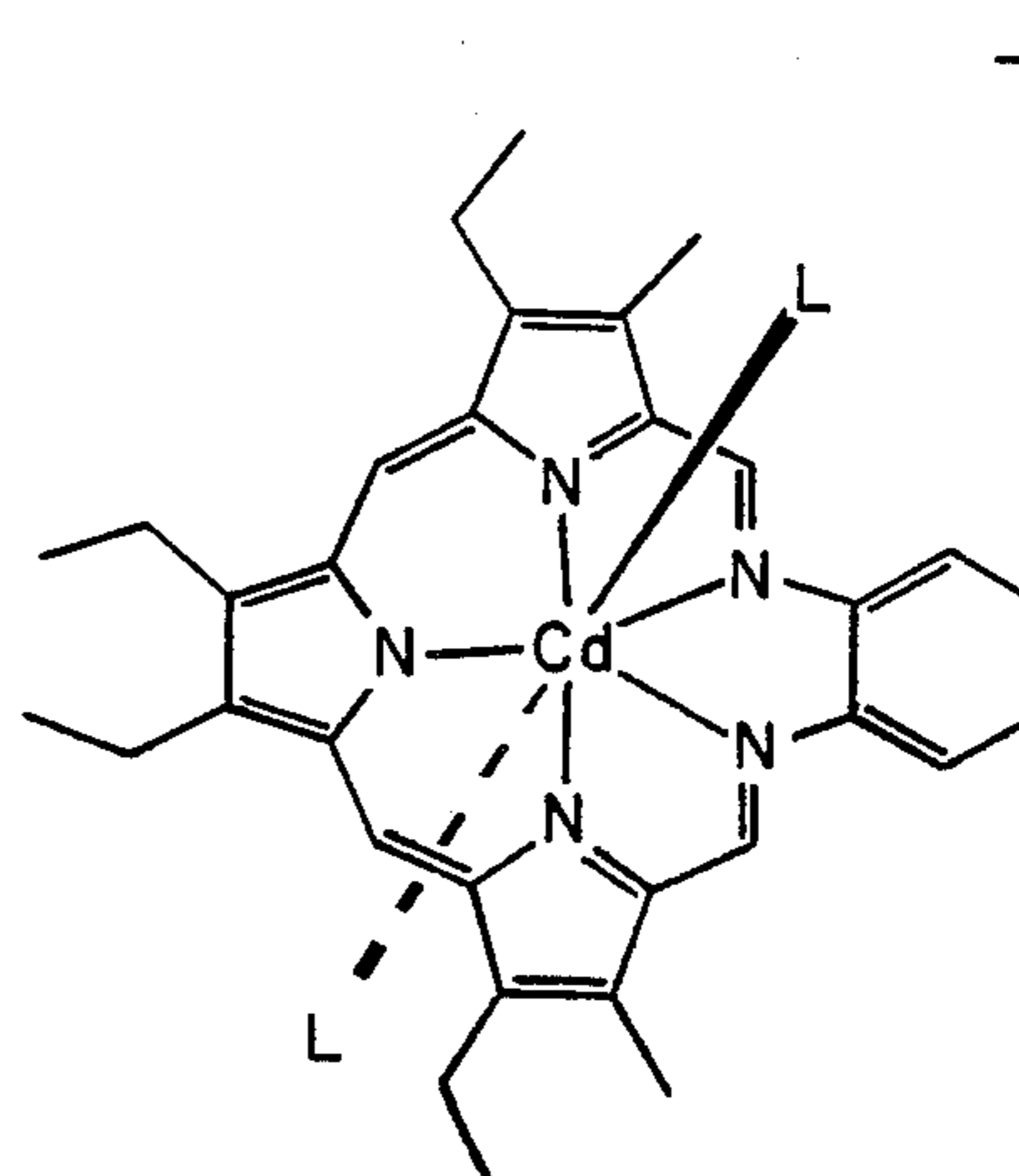
5aA. L = pyr 5bA. L = BzIm
