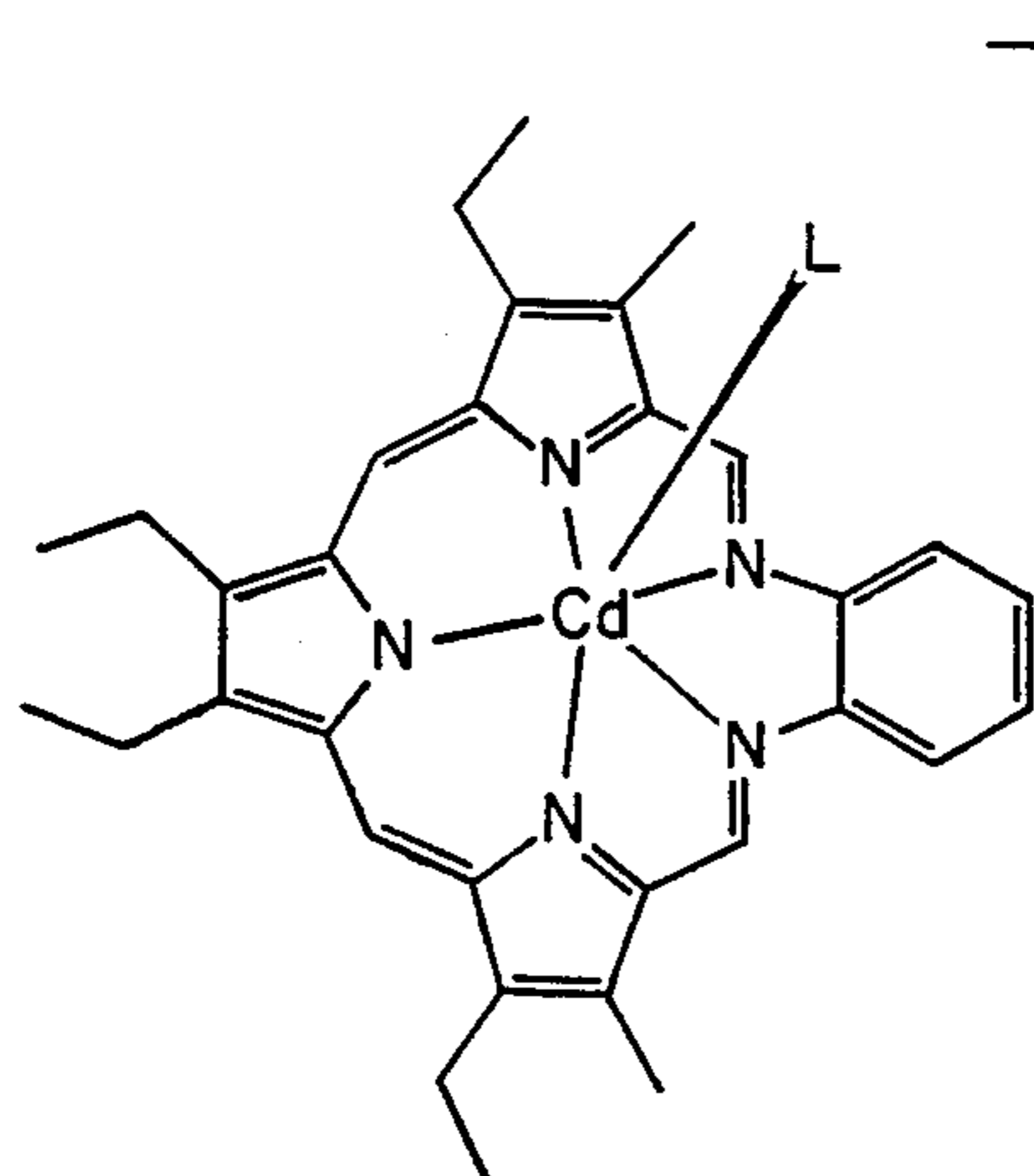
4aA. L = pyr 4bA. L = BzIm
