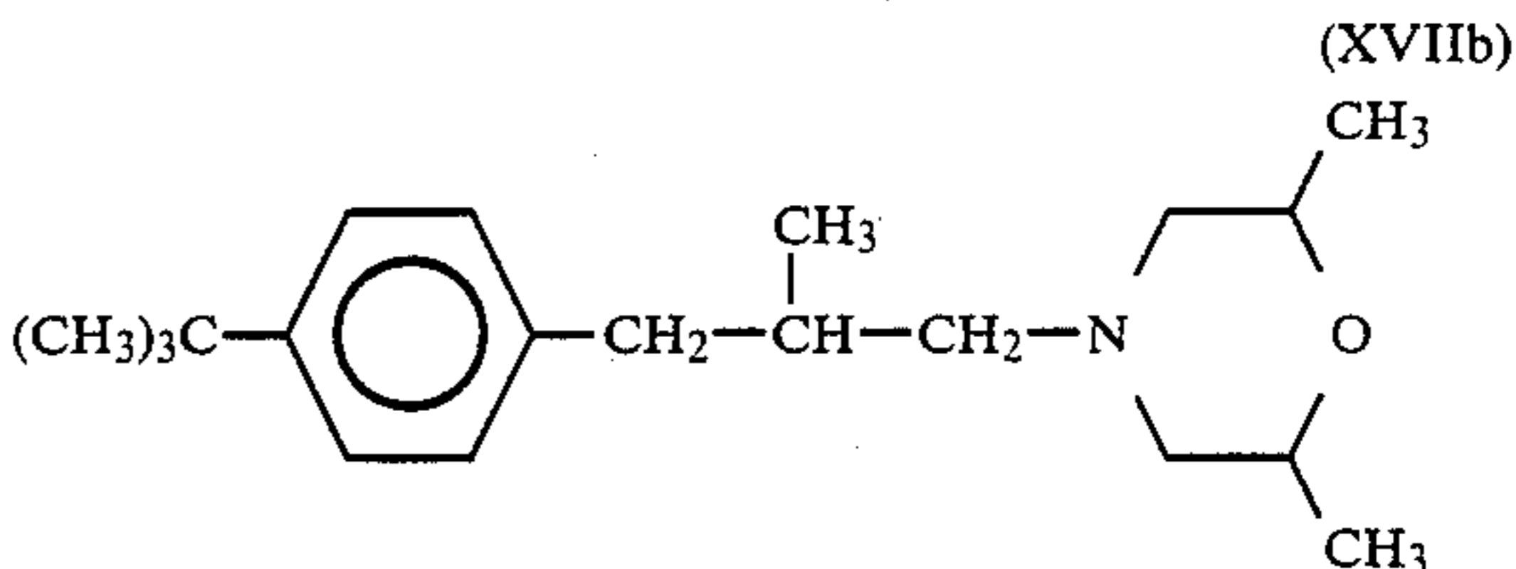
(FENPROPMORPH)
