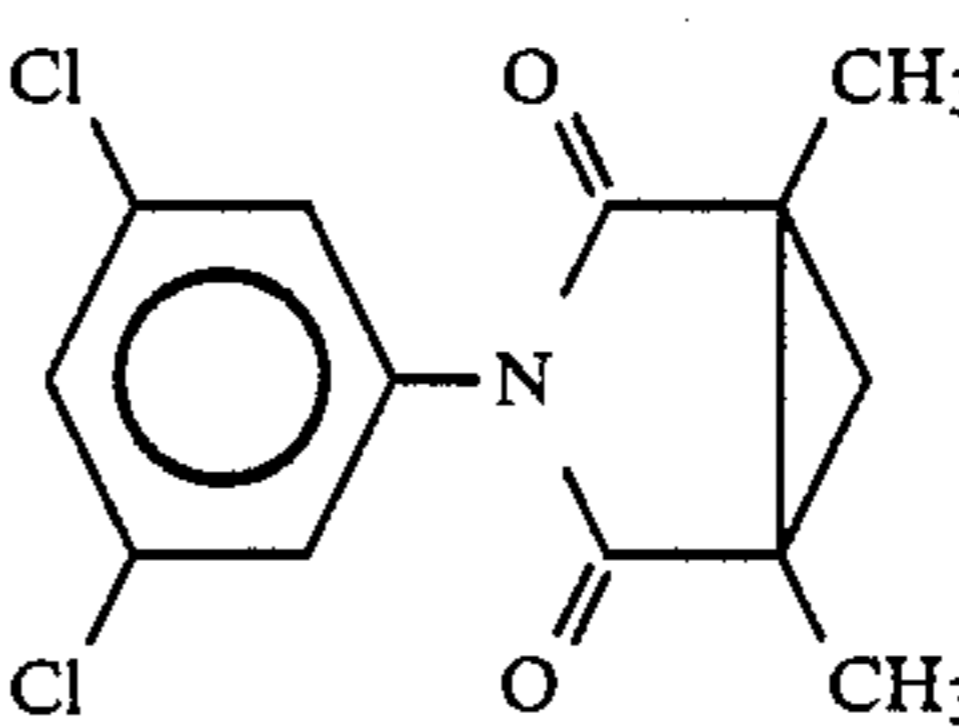
(PROCYMIDONE)
