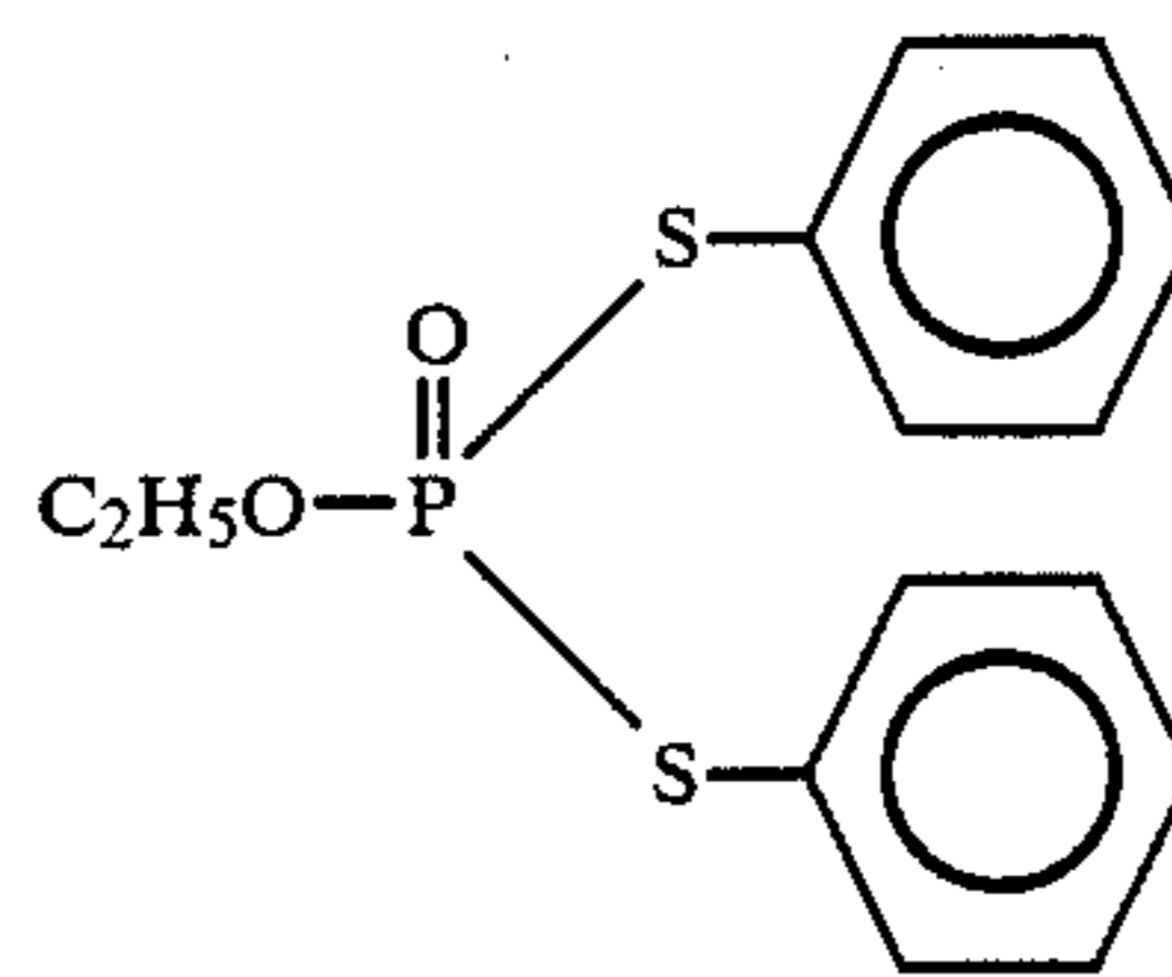
(EDIFENPHOS)
