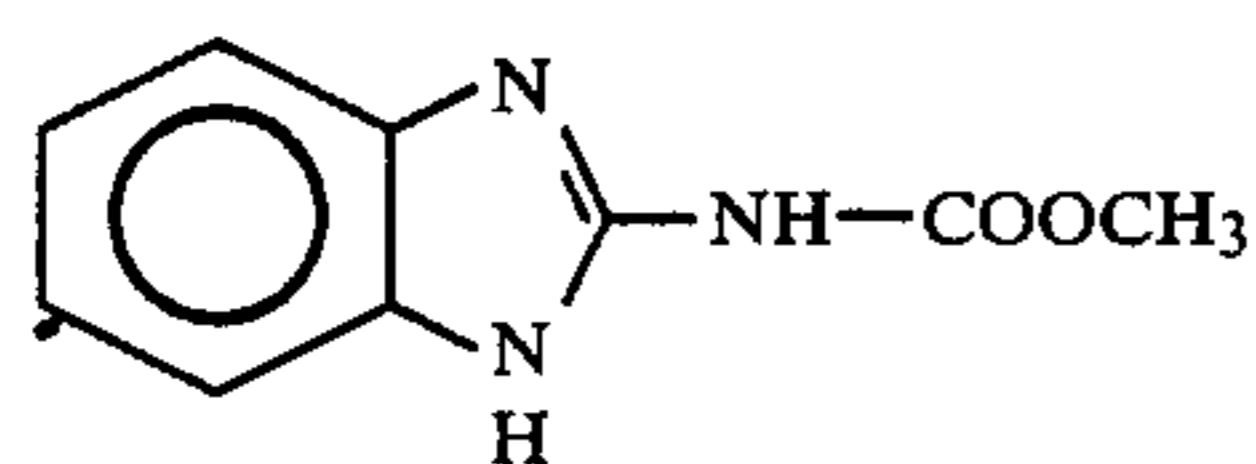
(CARBENDAZIM)
