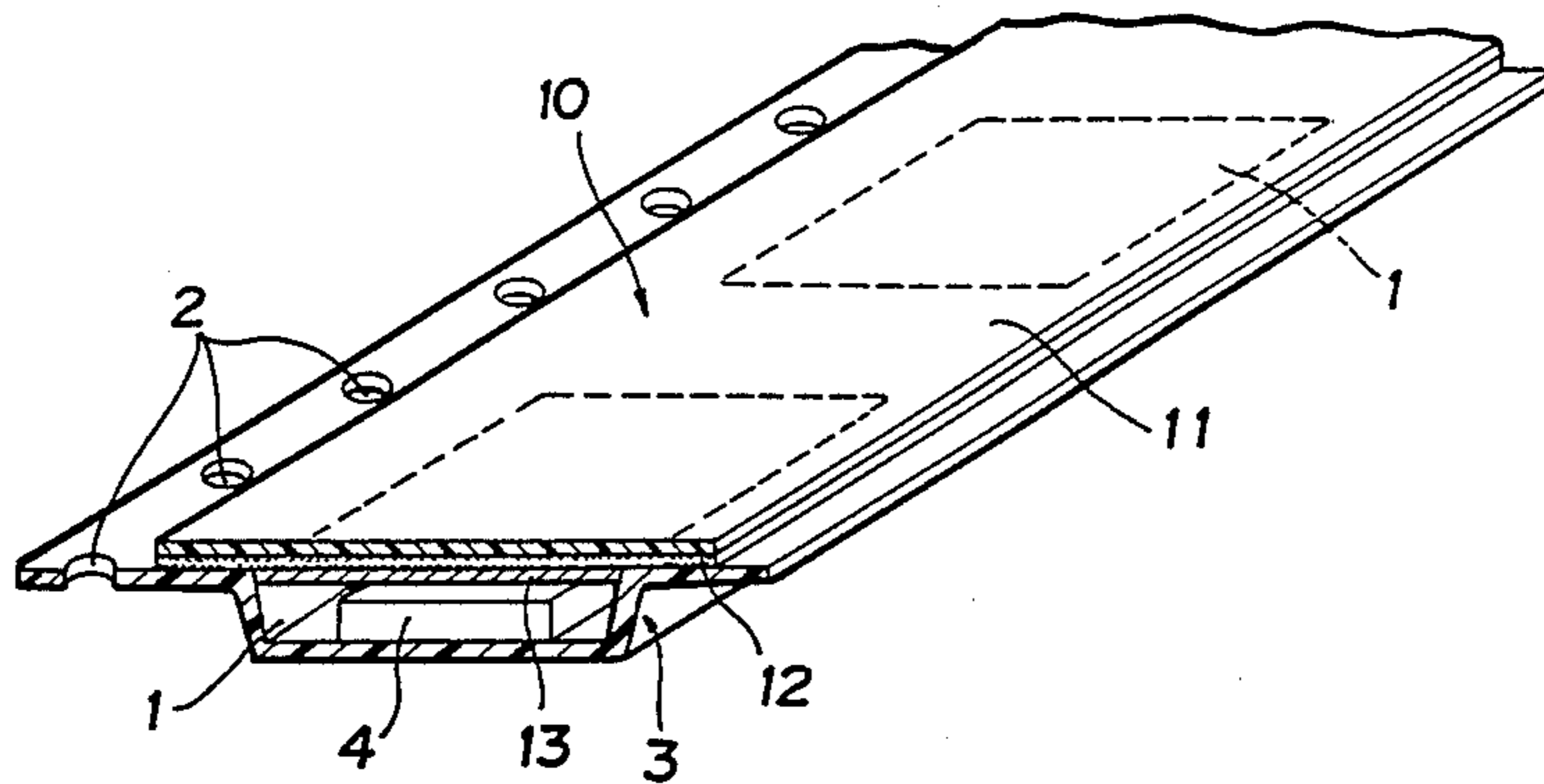
FIG. 3
