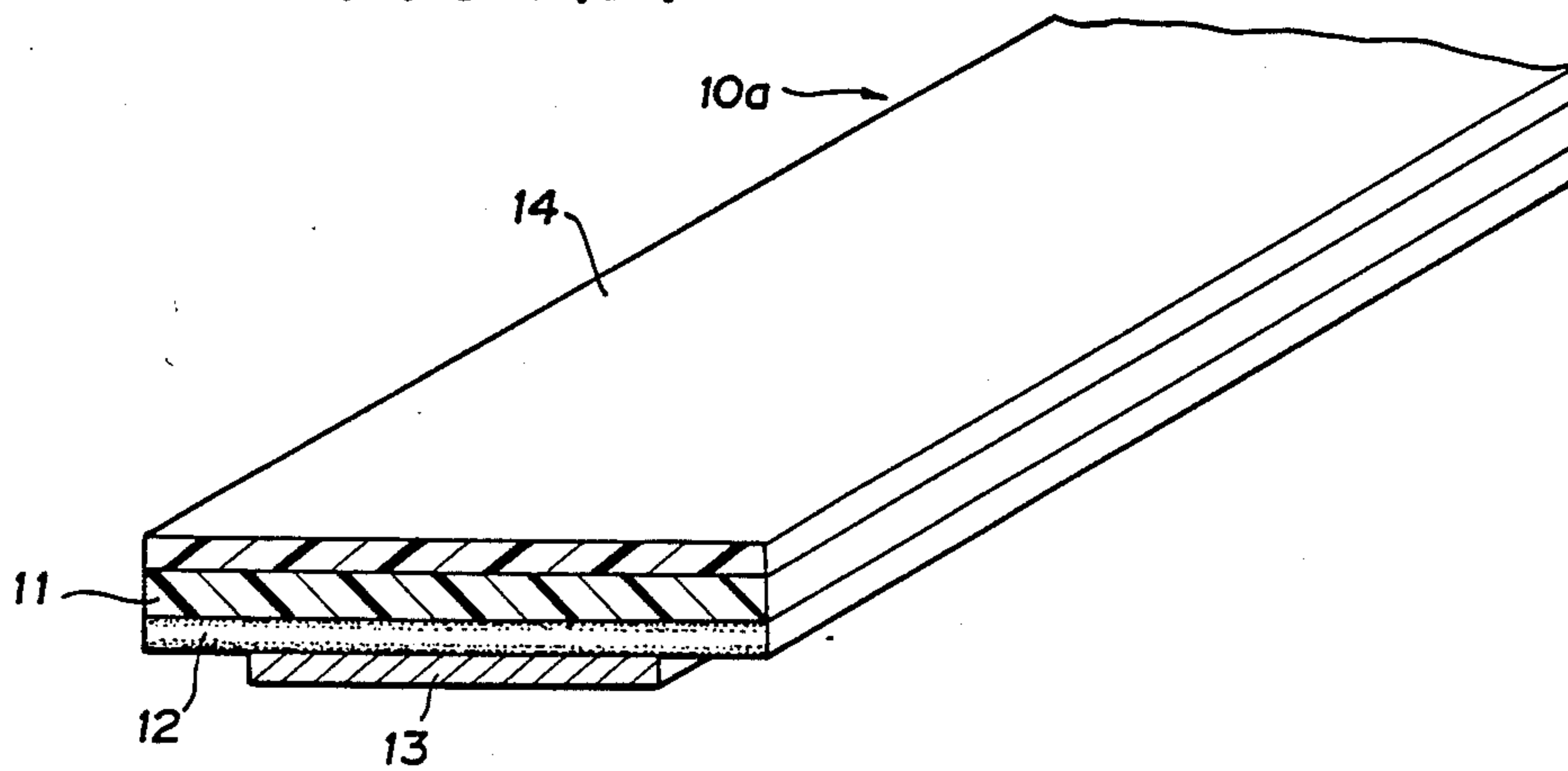
FIG. 1(B)
