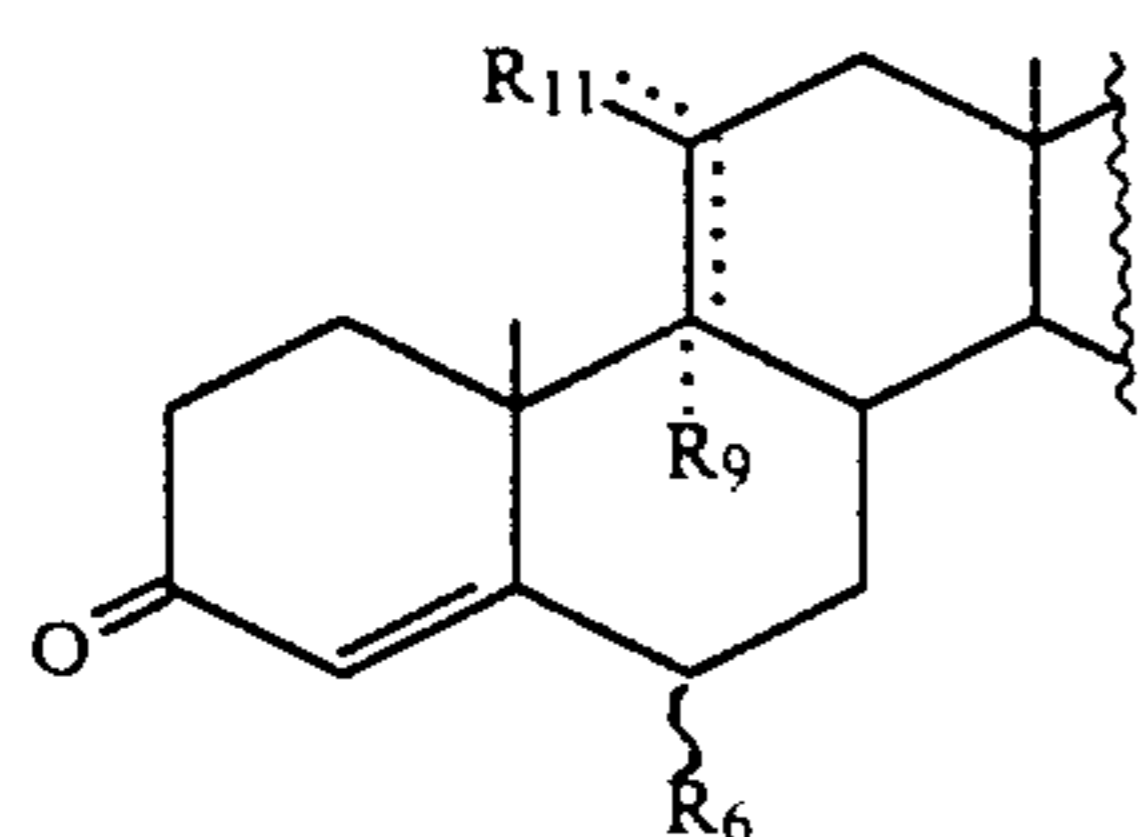
Δ 1,4 -3-keto steroids
