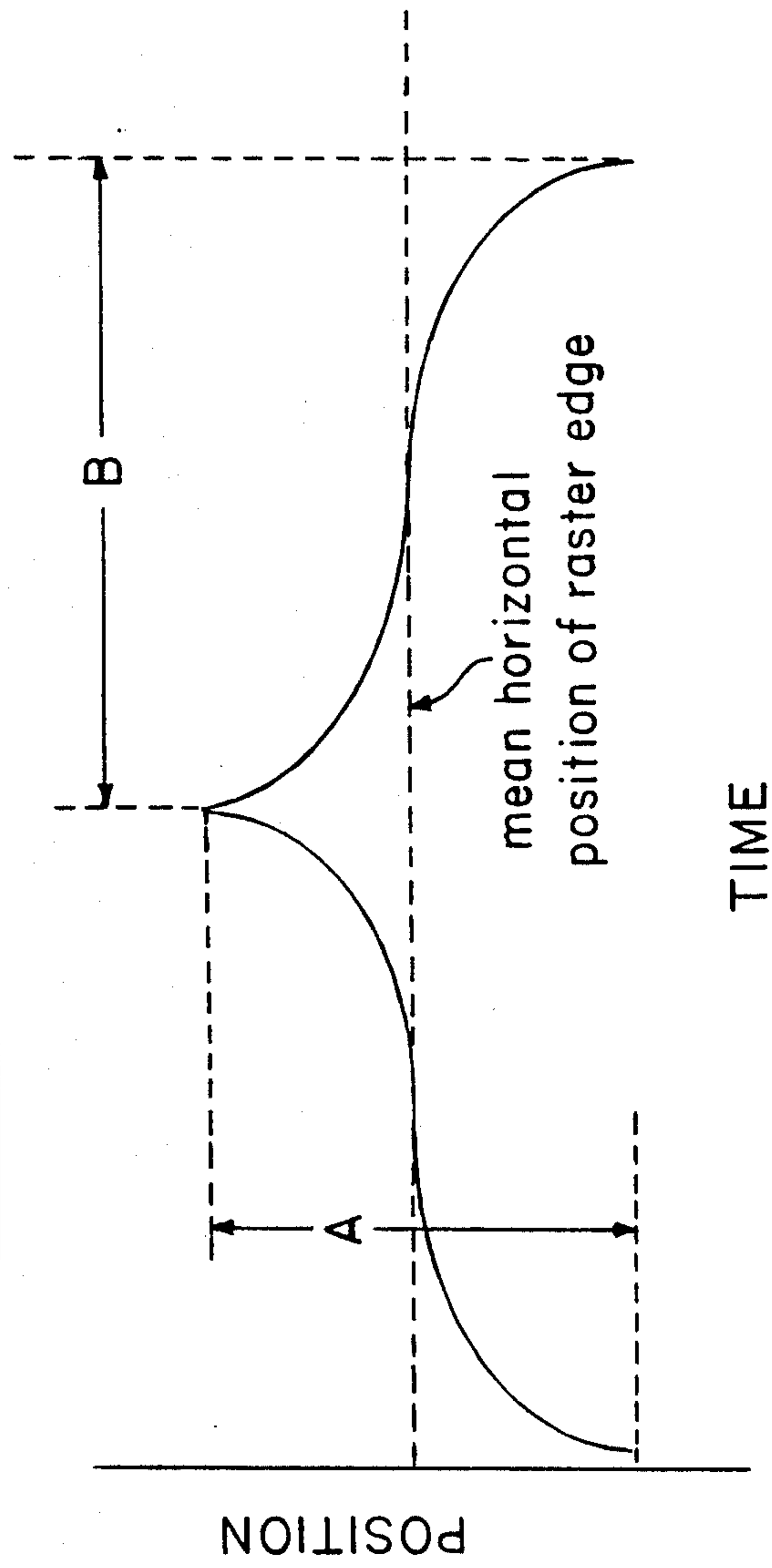
FIG. 3 Exemplary Dither Waveform
