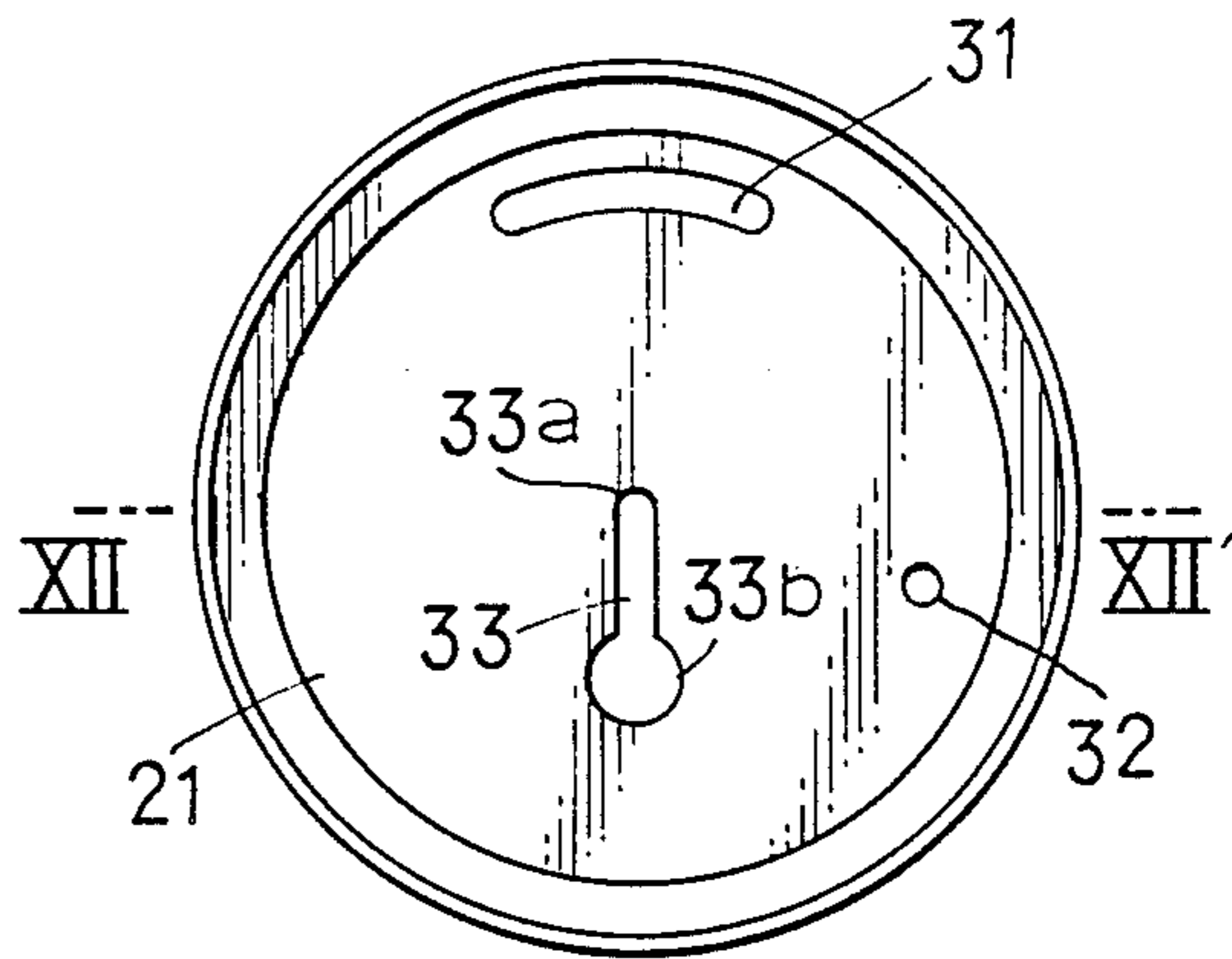
FIG. 11.
