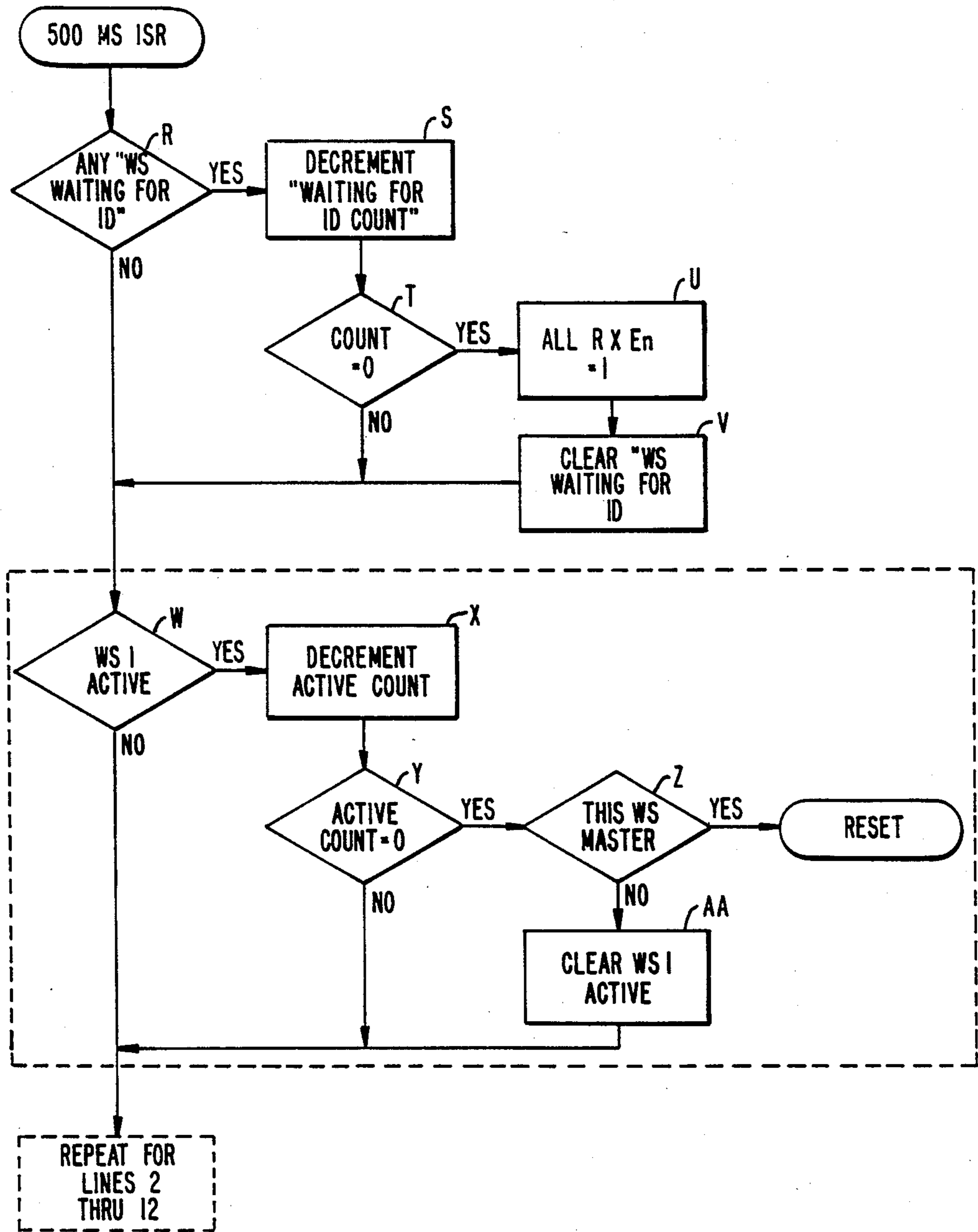
FIG. 5B.
