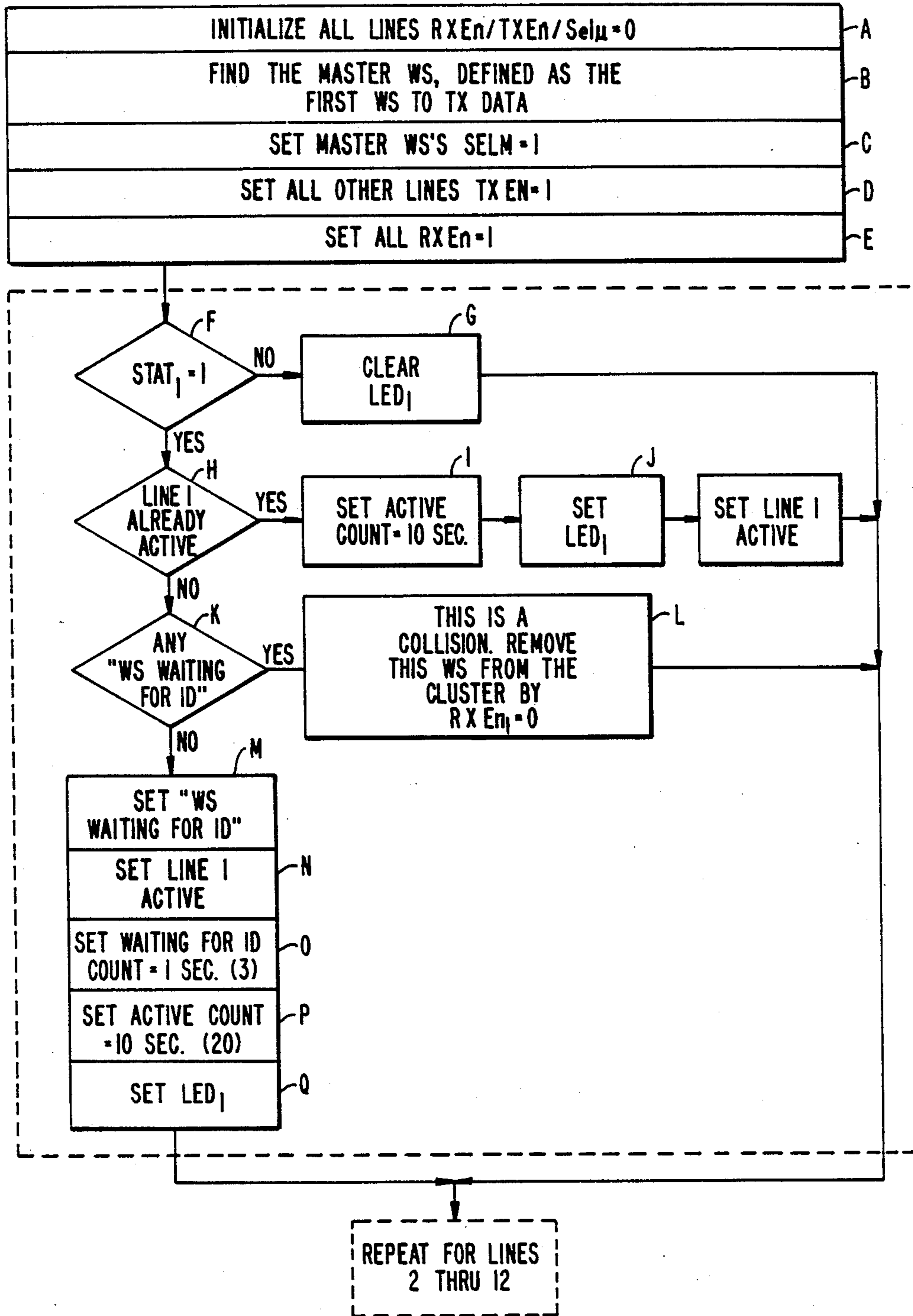
FIG. 5A.
