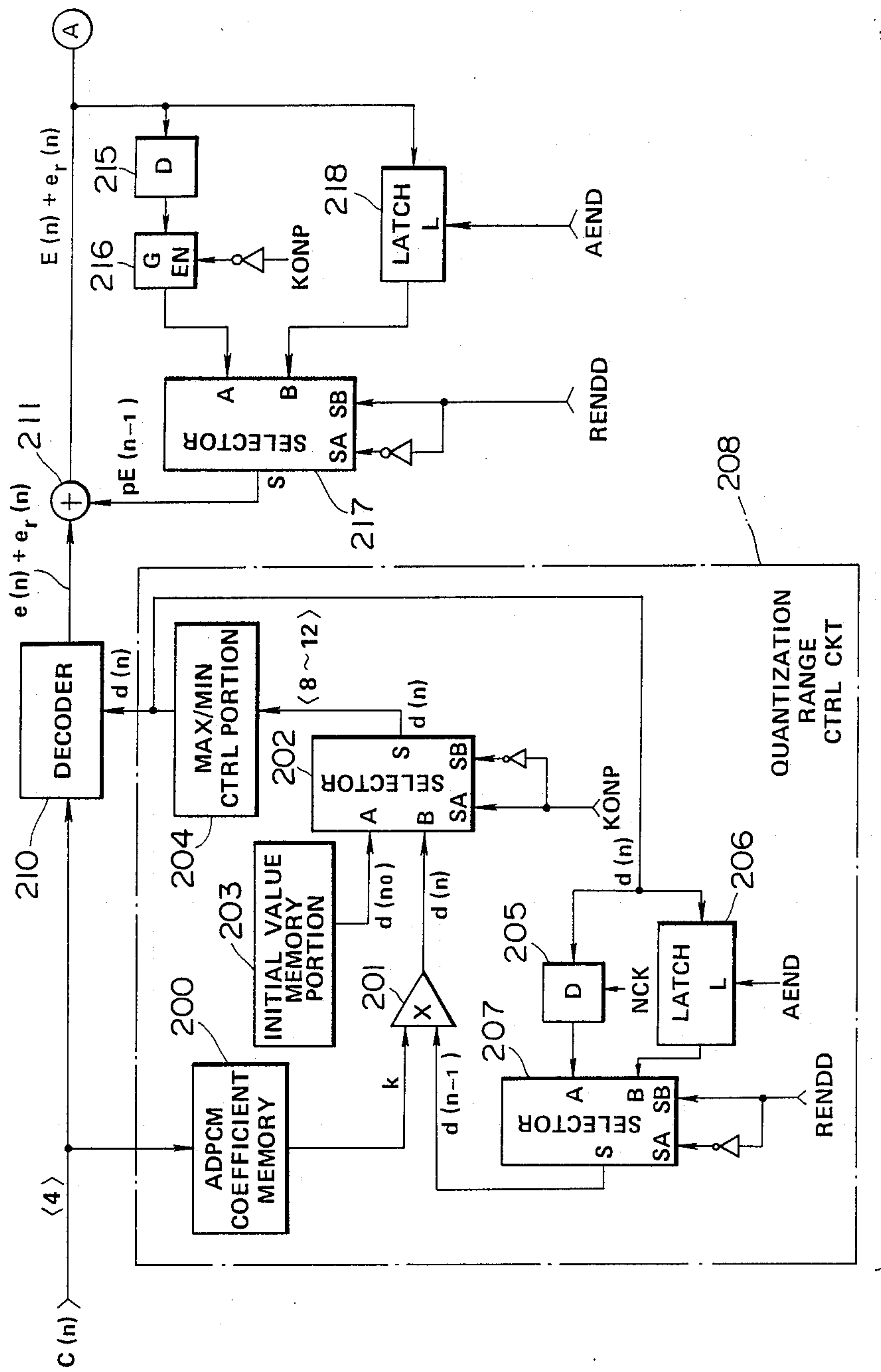
ADPCM DECODING CKT 124A
