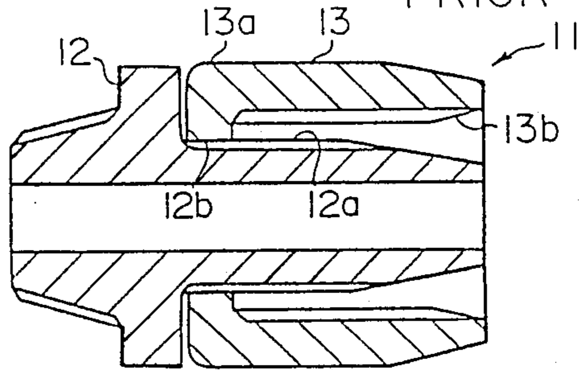
FIG. 16(a) PRIOR-ART
