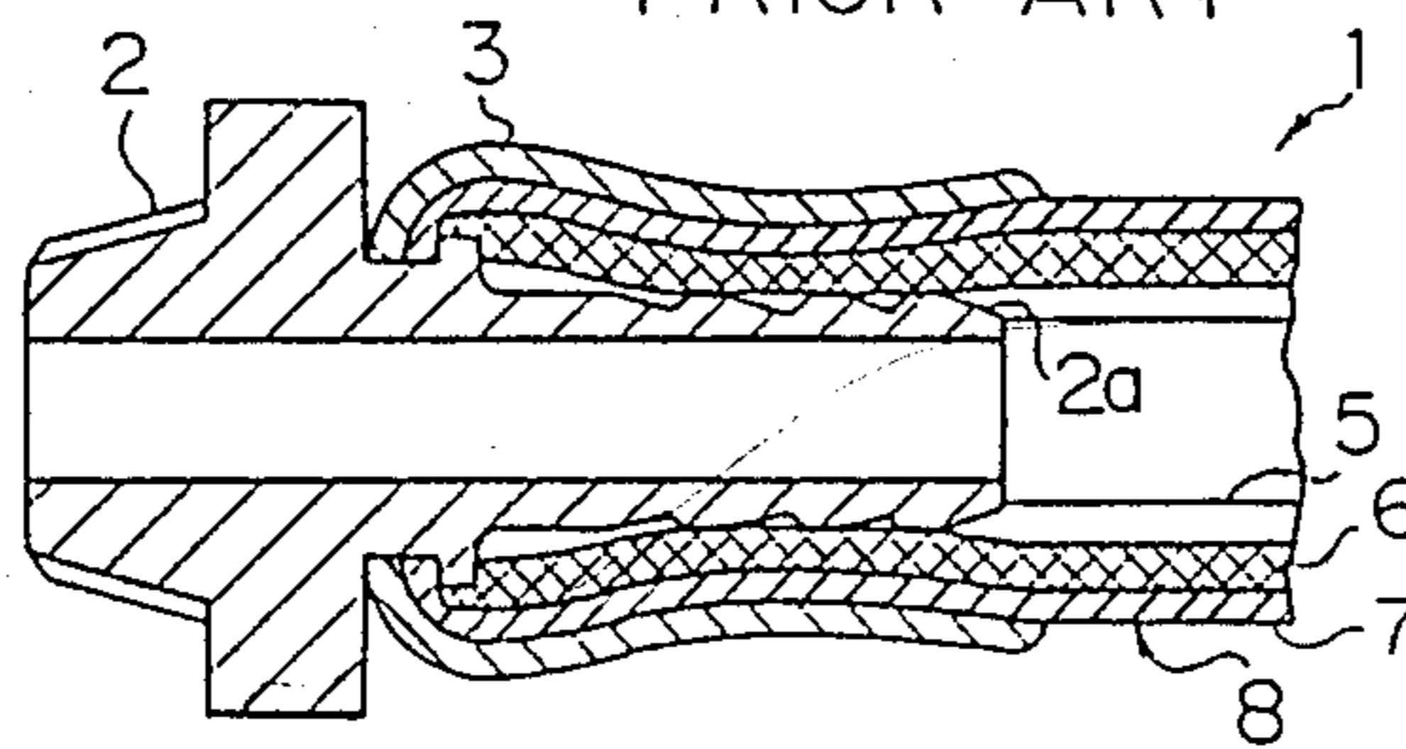
FIG. 15 PRIOR-ART
