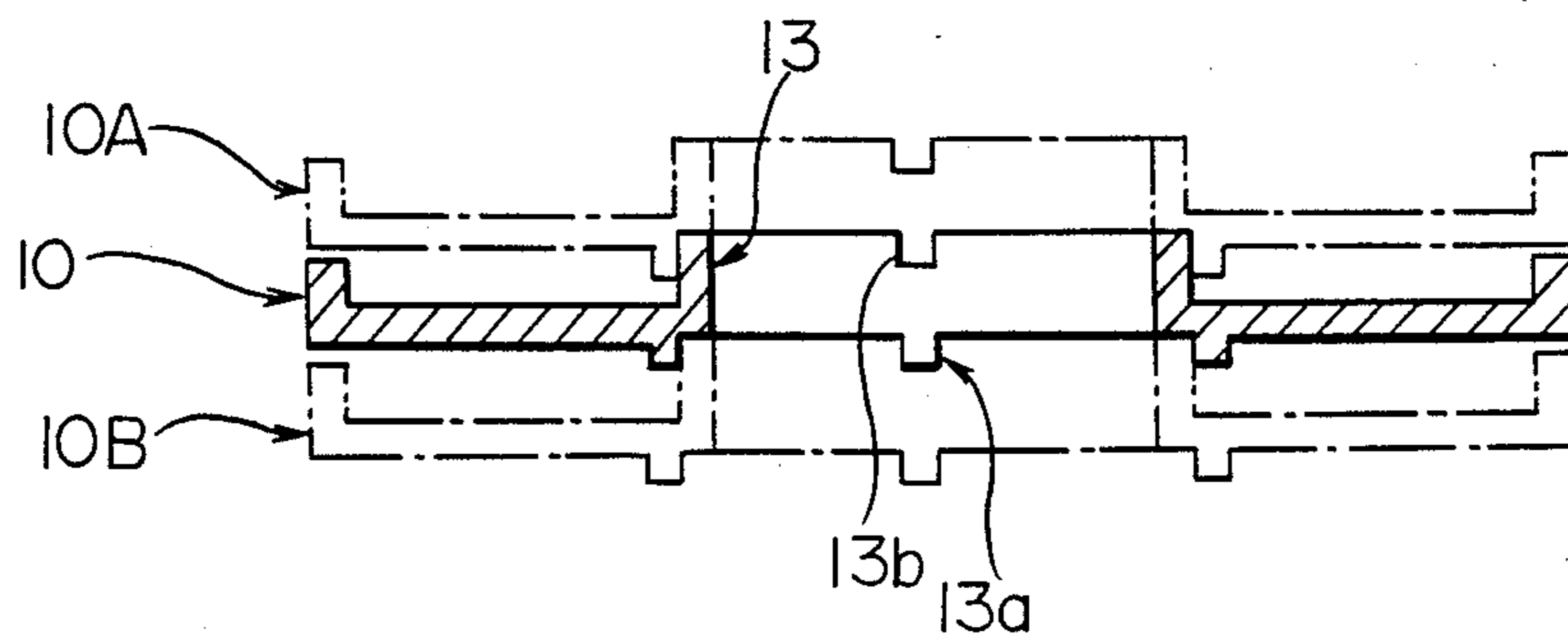
FIG. 6
