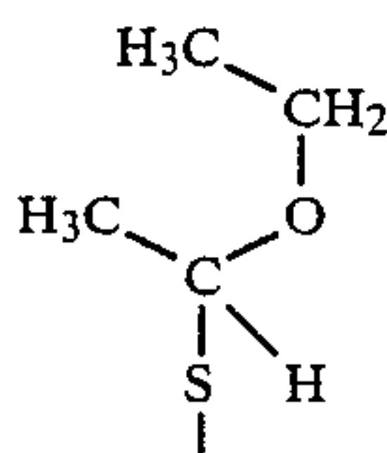
ethoxyethyl
