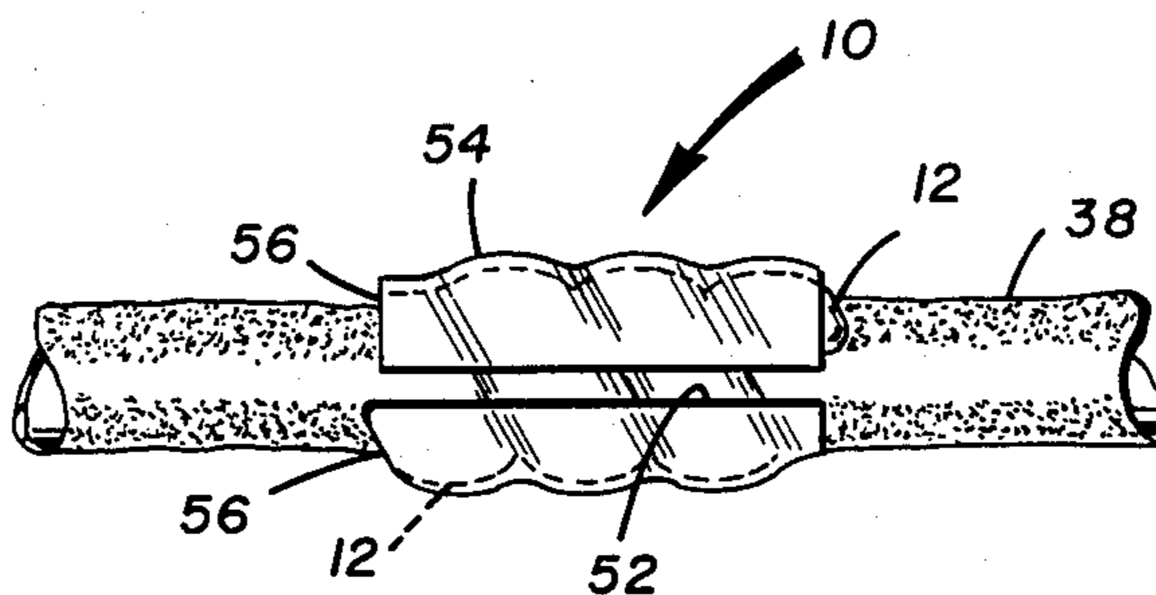
FIG. 8a
