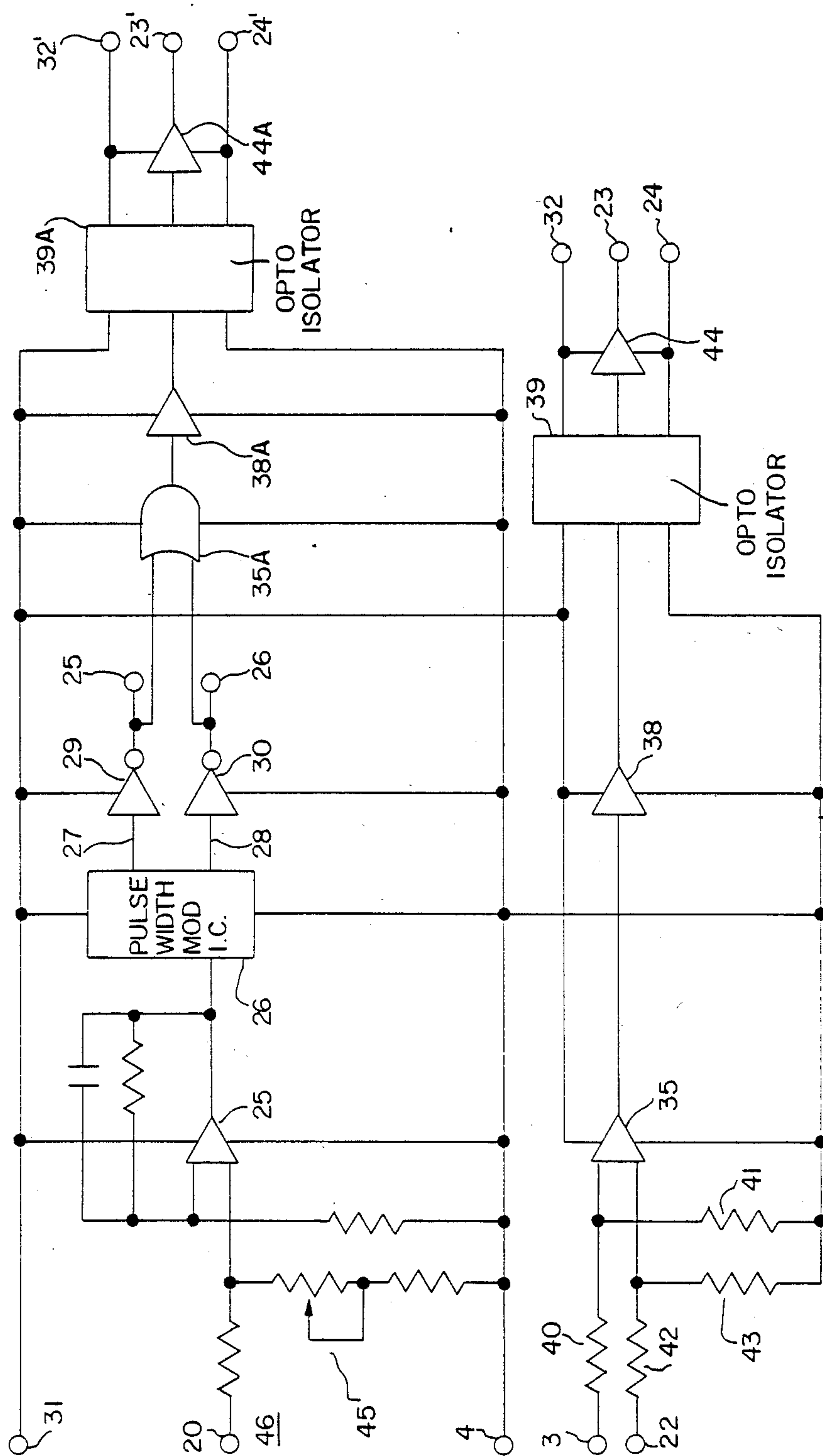
FIG. 2C
