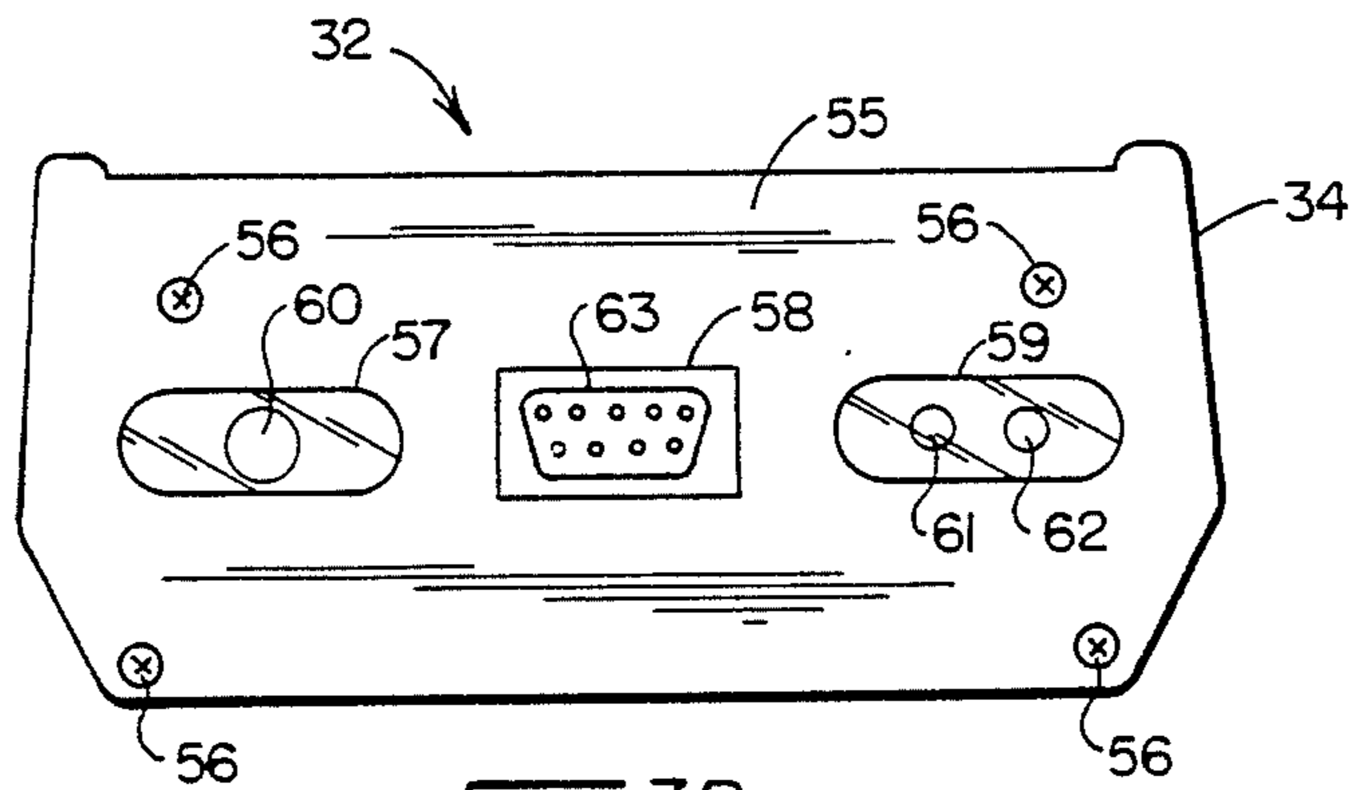
FIG. 3B
