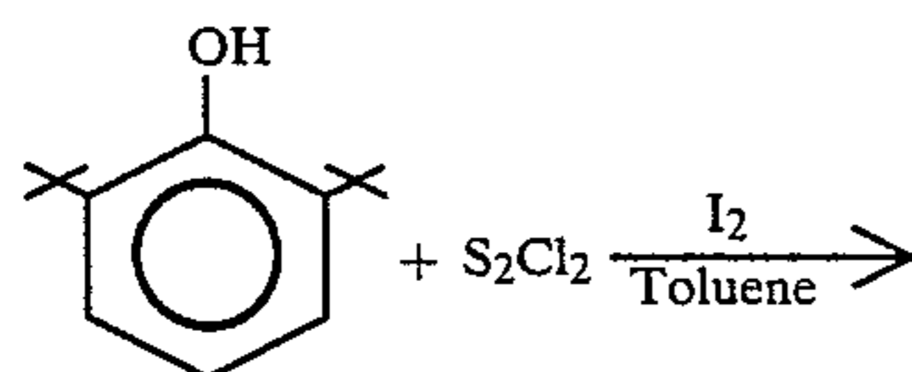
(I) DTBP
