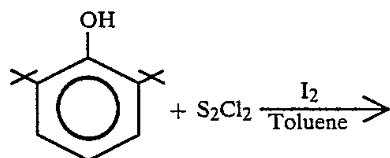
(I) DTBP
