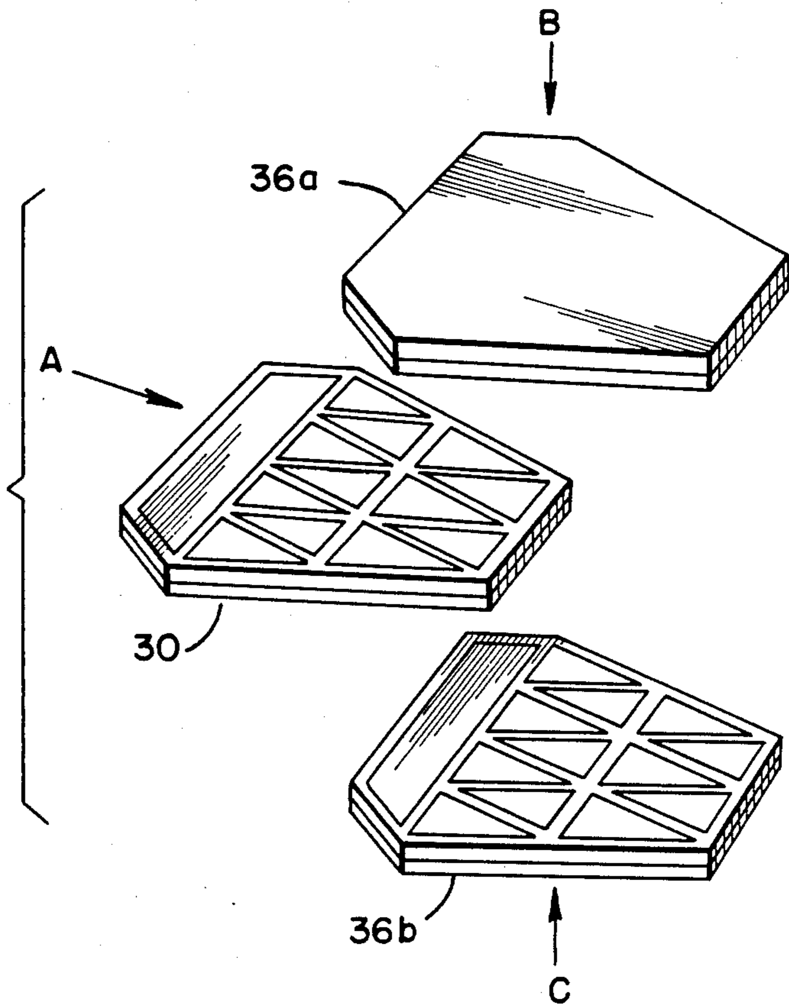
FIG. 3A.
