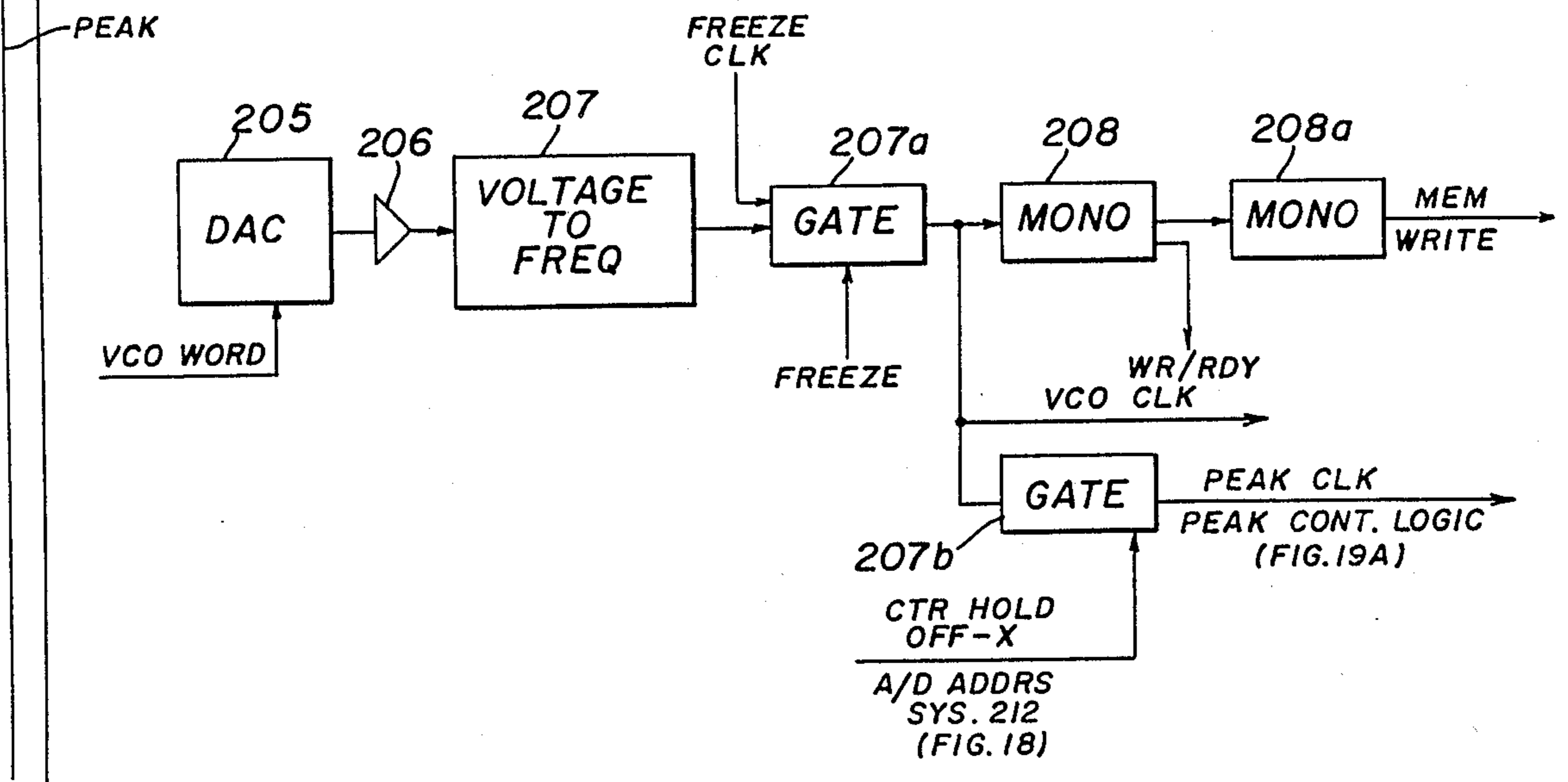
VCO CLOCK GEN. 204
