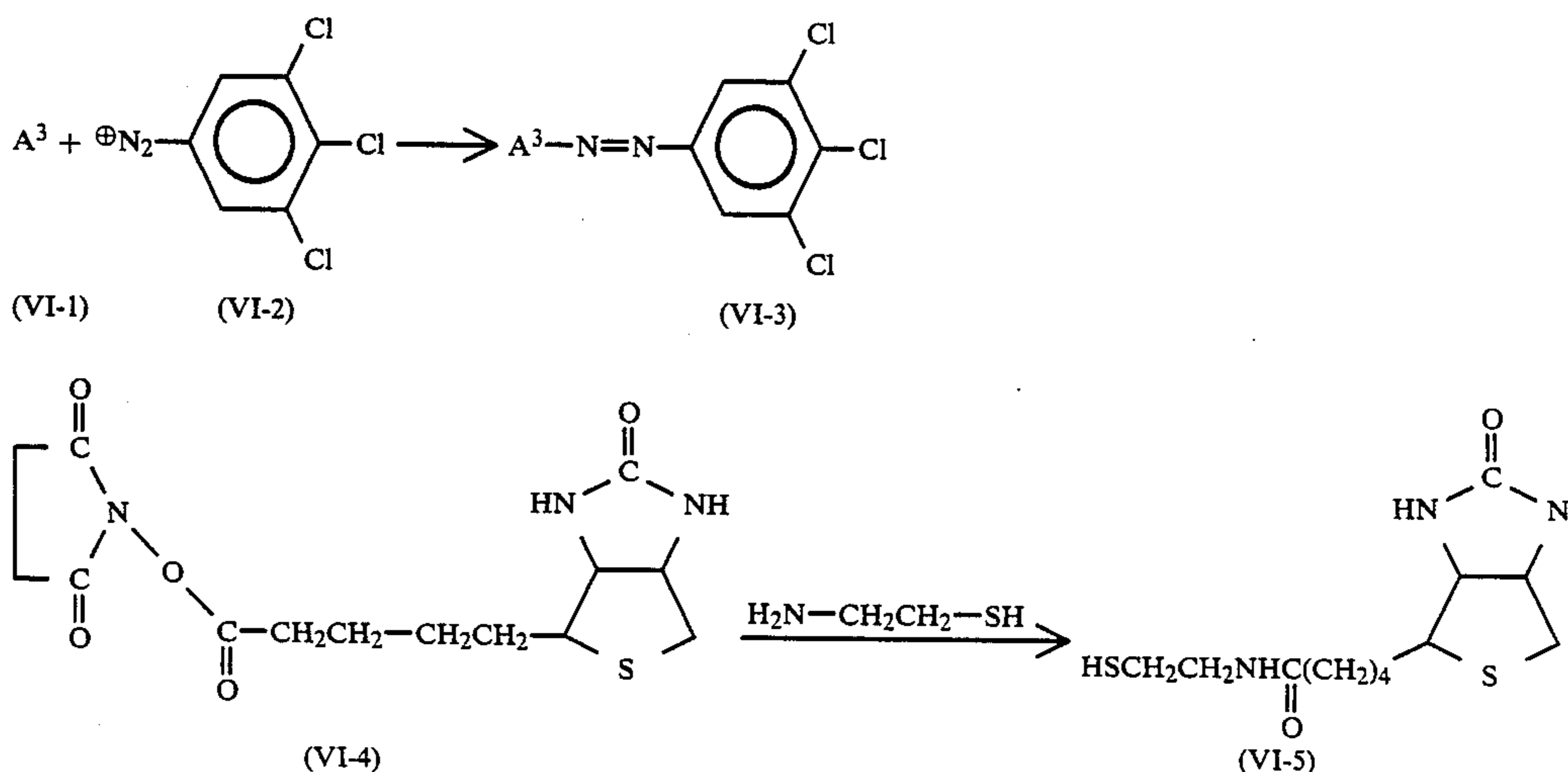
Scheme VI:
