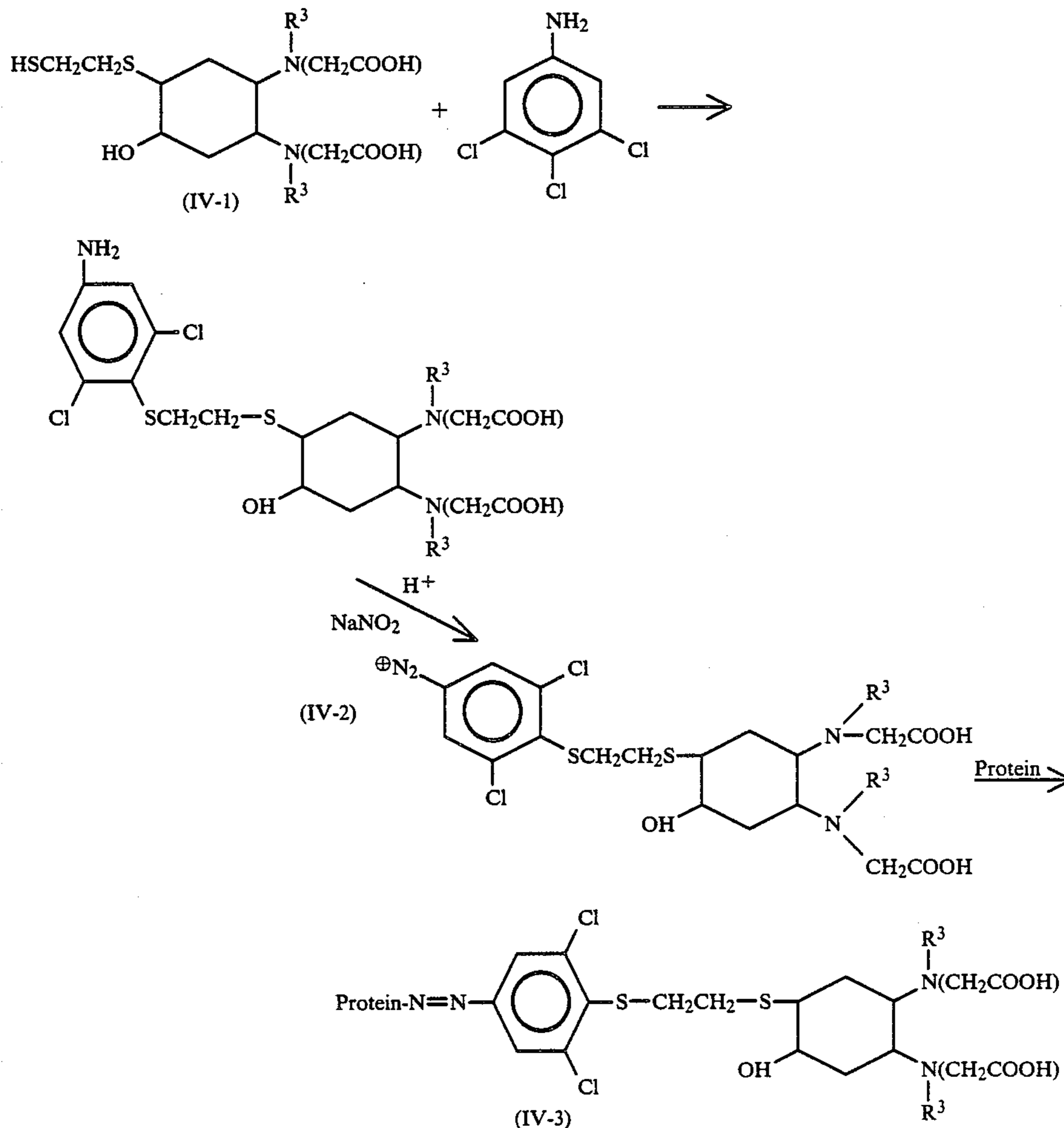
Scheme IV:
