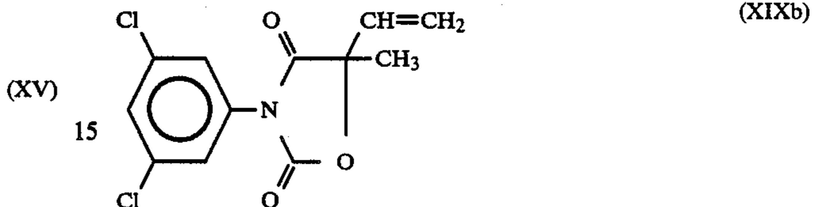
(XV) 15 (VINCHLOZOLIN)
