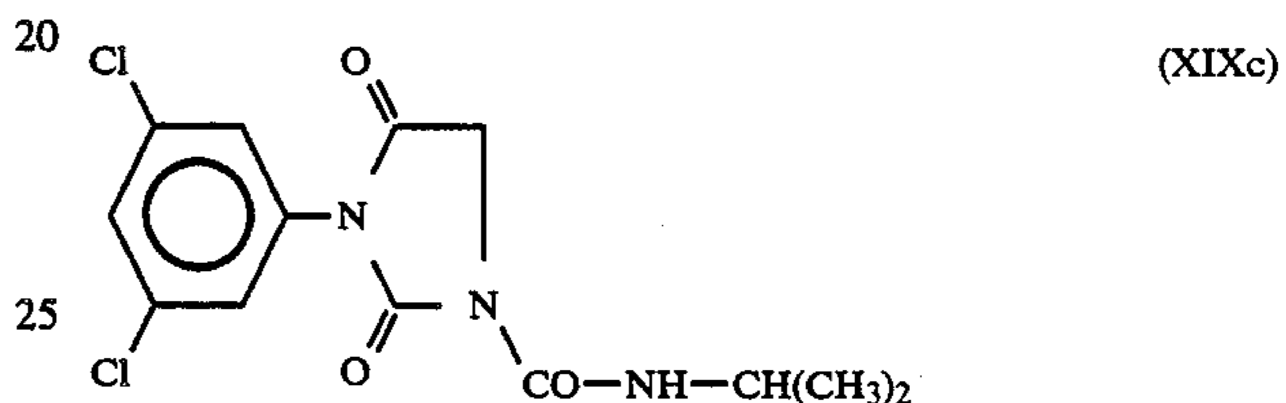
(XVI) 20 (IPRODIONE)
