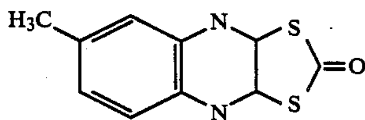
(CHINOMETHIONAT)
