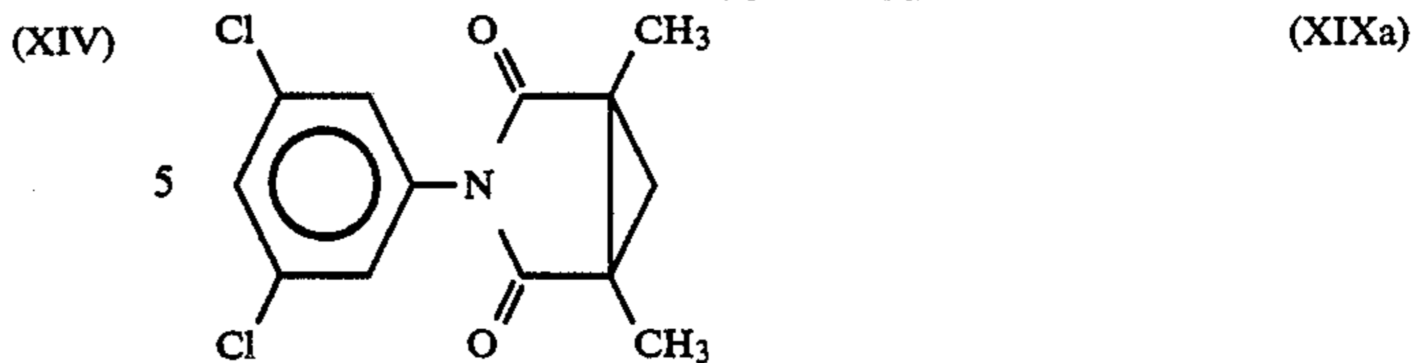
(XIV) 5 (PROCYMIDONE)
