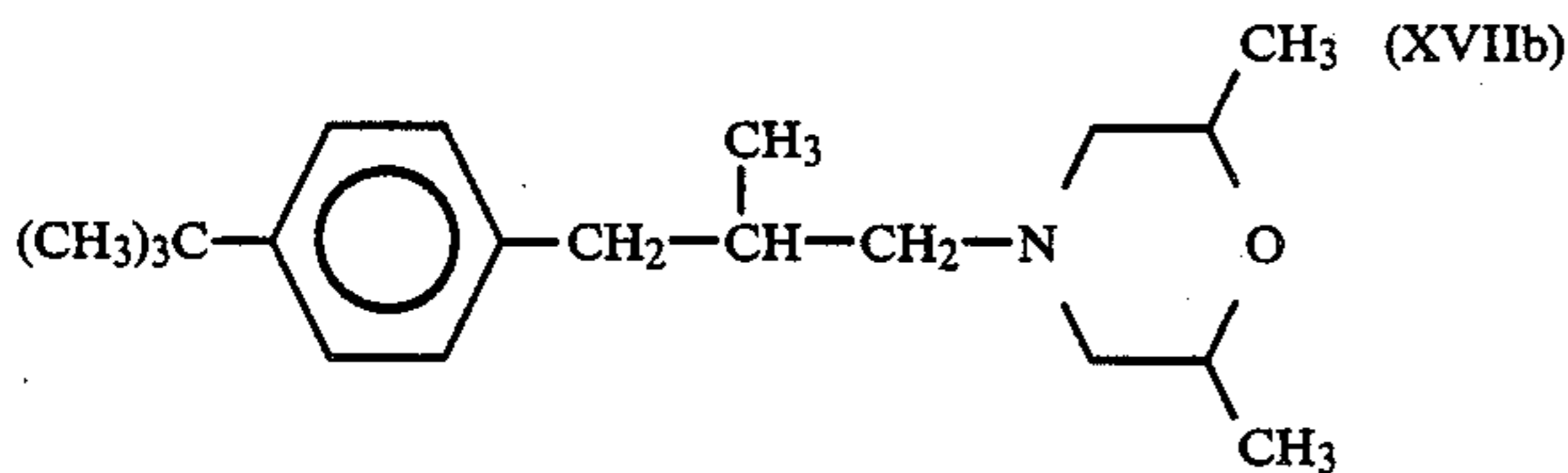
(FENPROPEMORPH)
