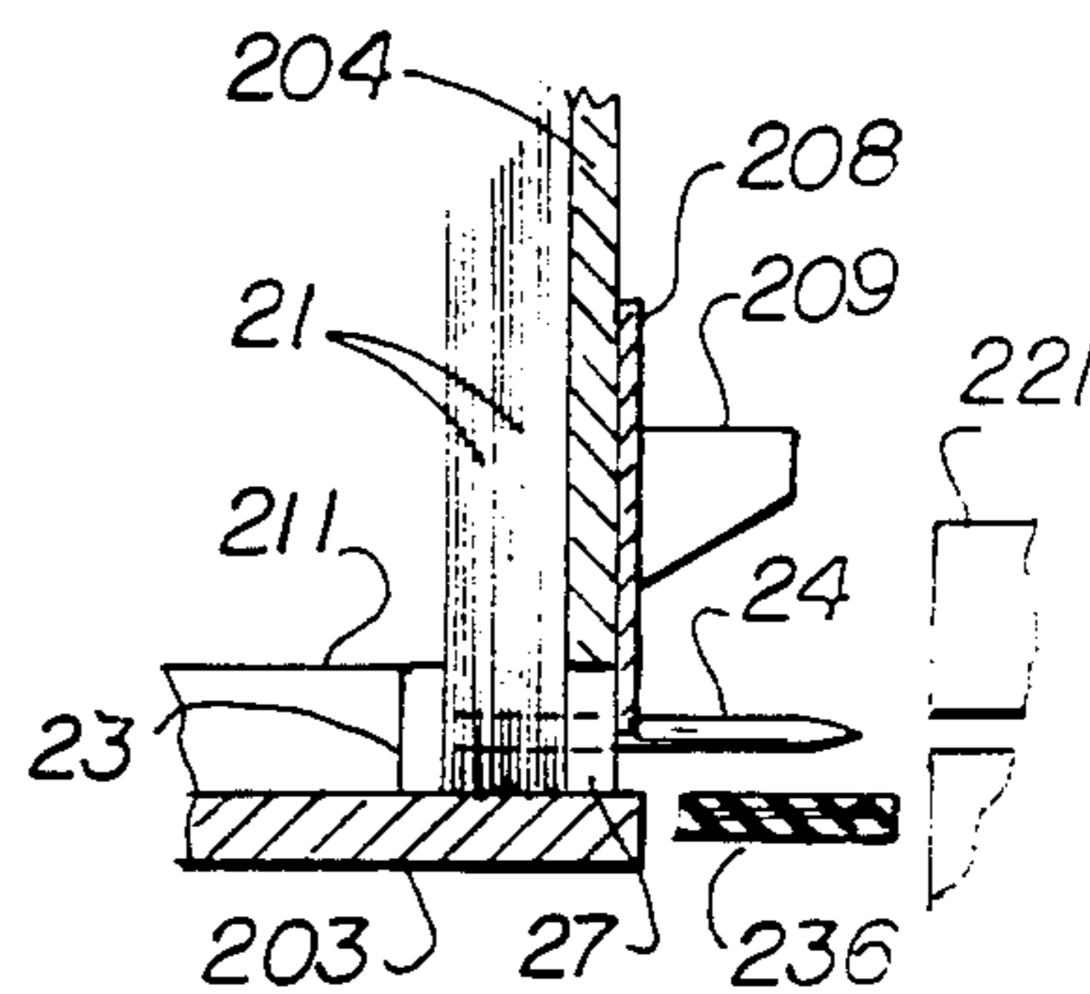
Fig. 24
