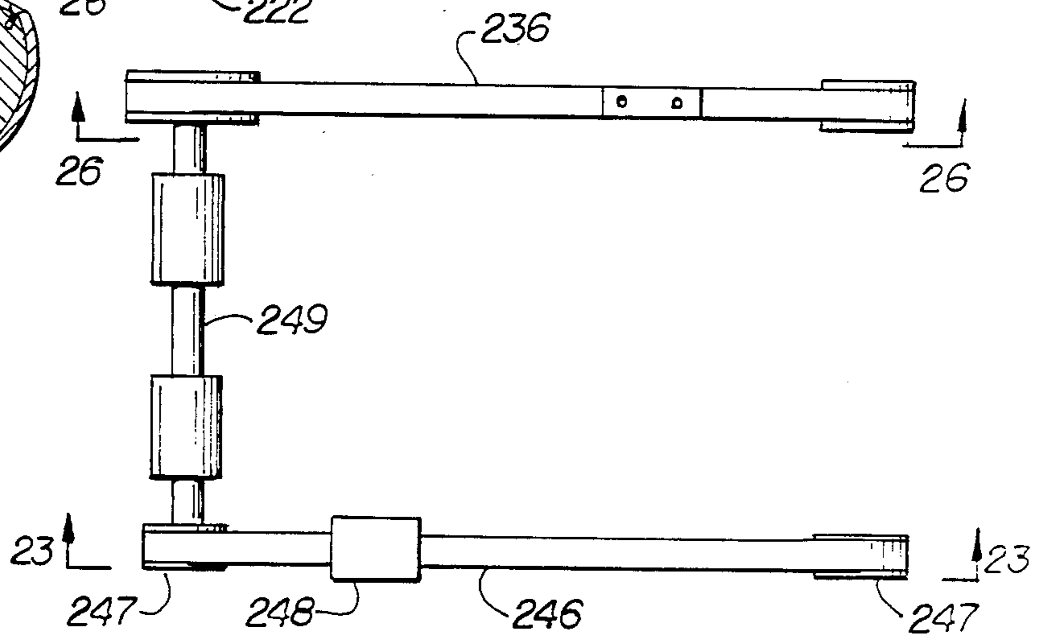
Fig. 22
