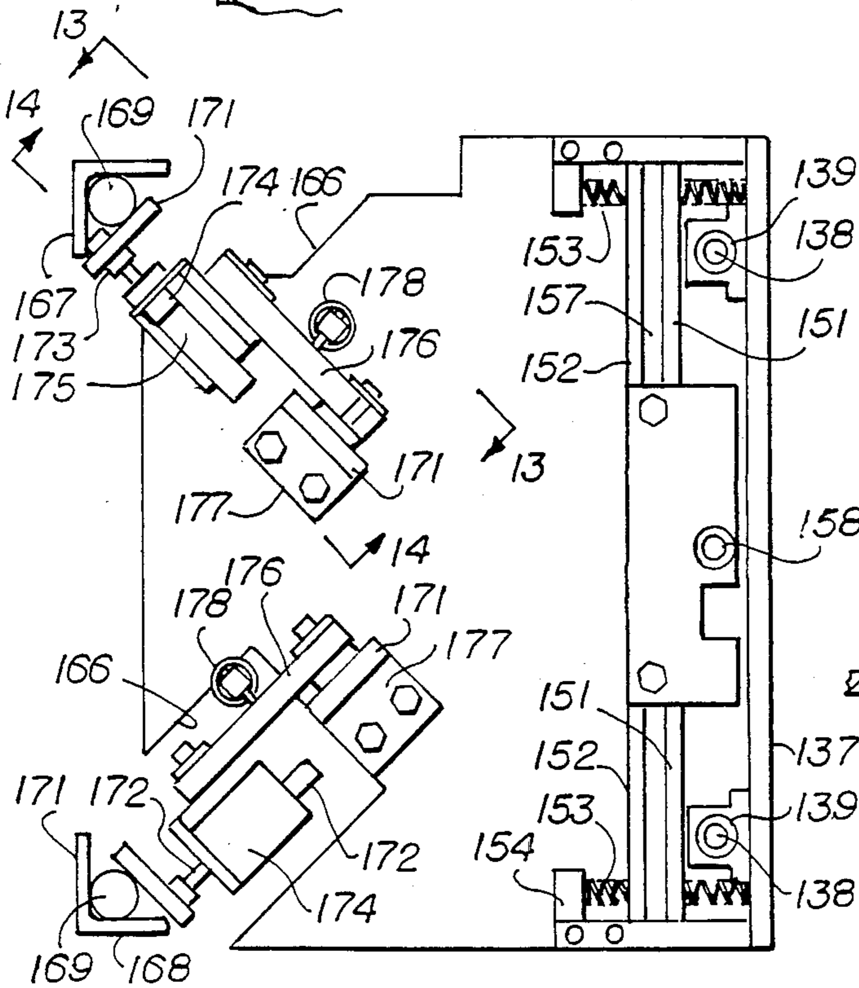
Fig. 12
