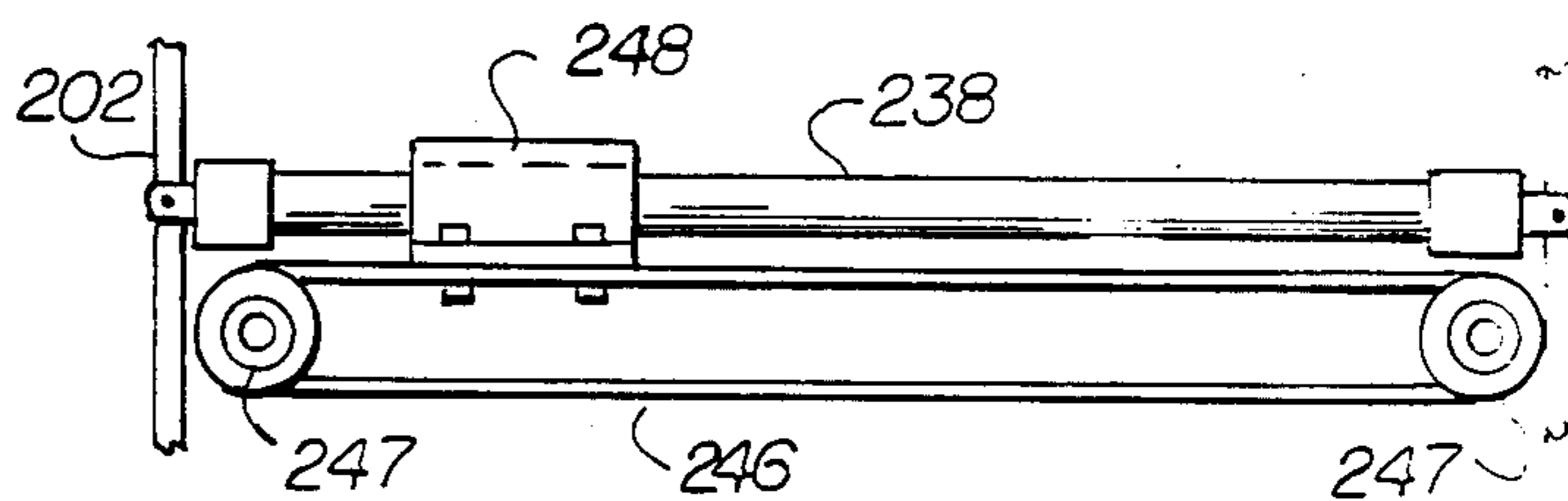
Fig. 23
