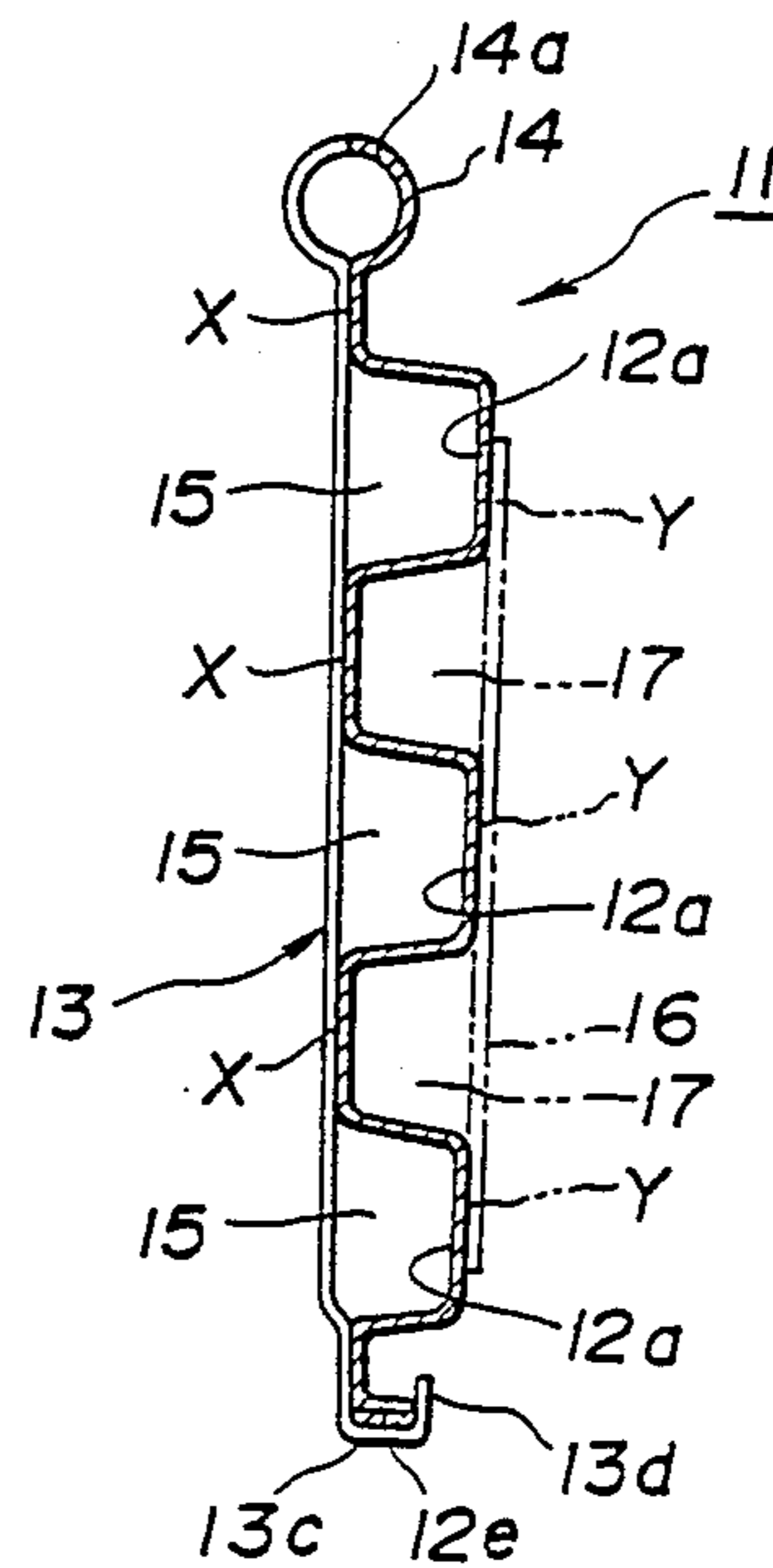
FIG. 13
