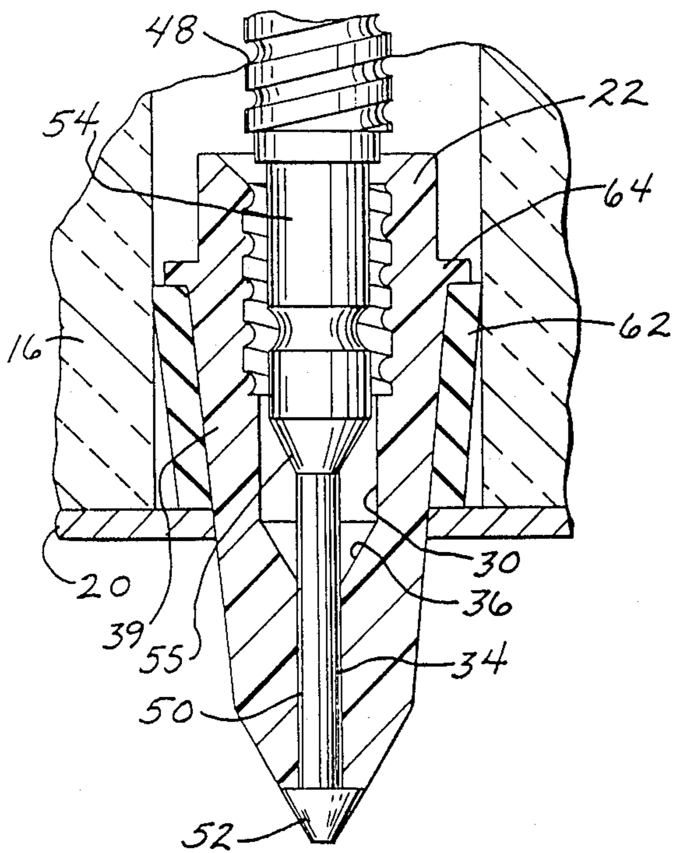
FIG. 9
