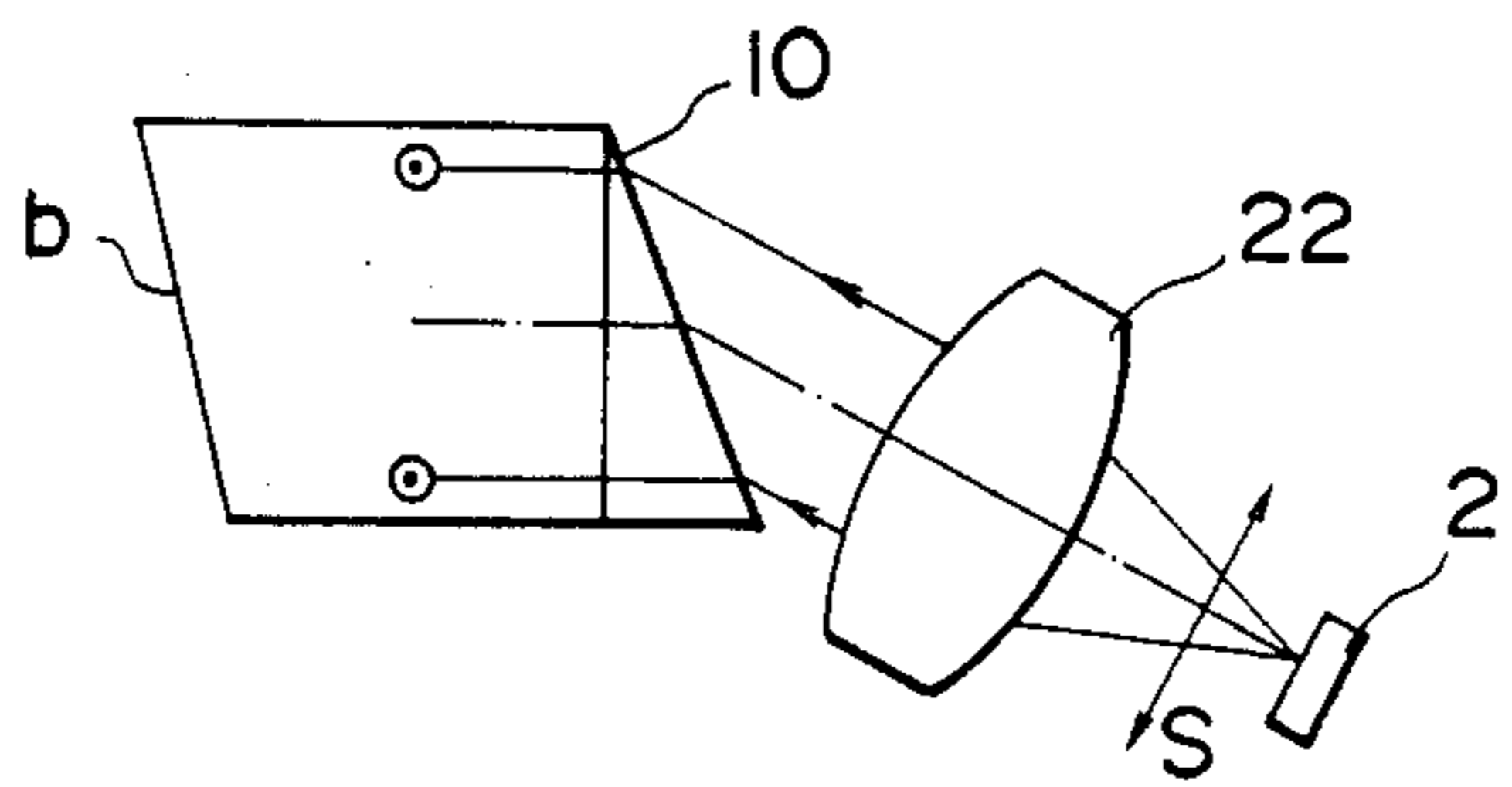
FIG. 10B
