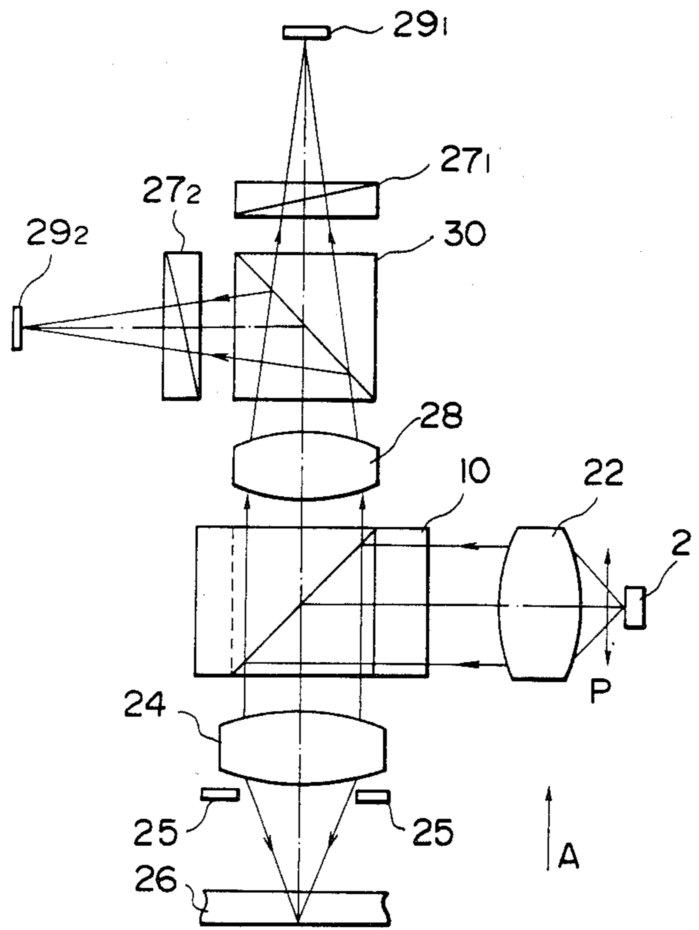
FIG. 10A
