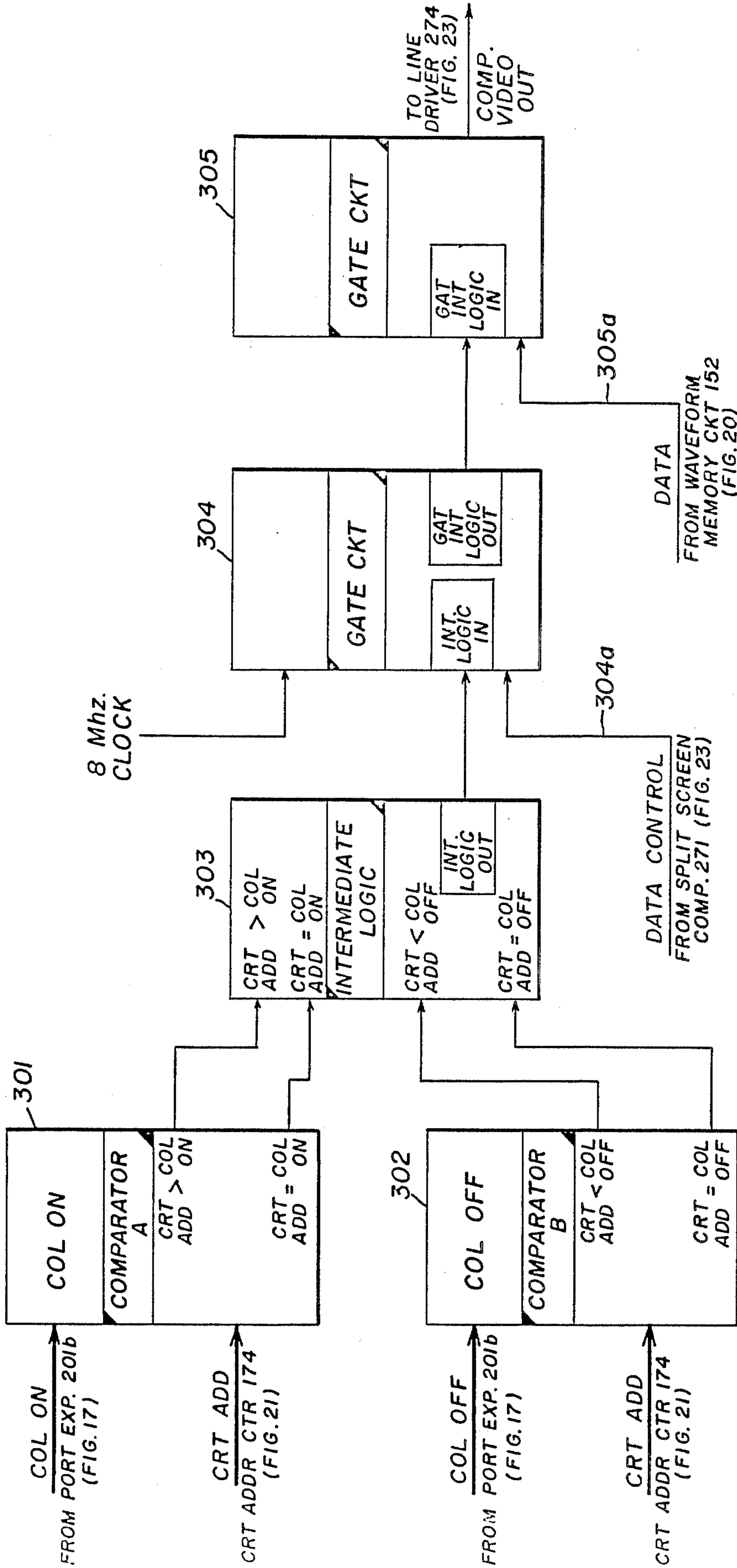
FIG. 25 CURTAIN CIRCUIT 273
