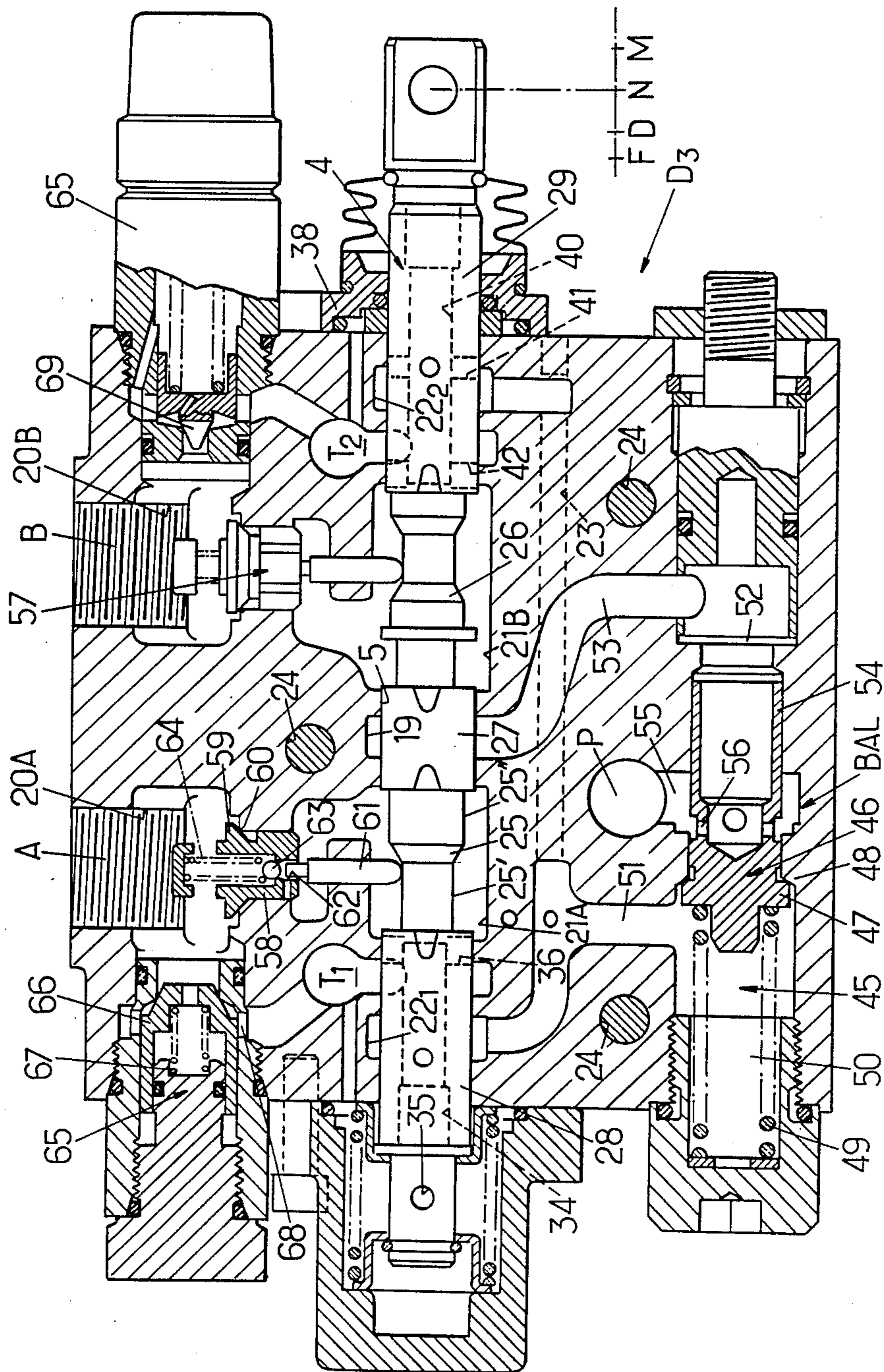
FIG. 7.
