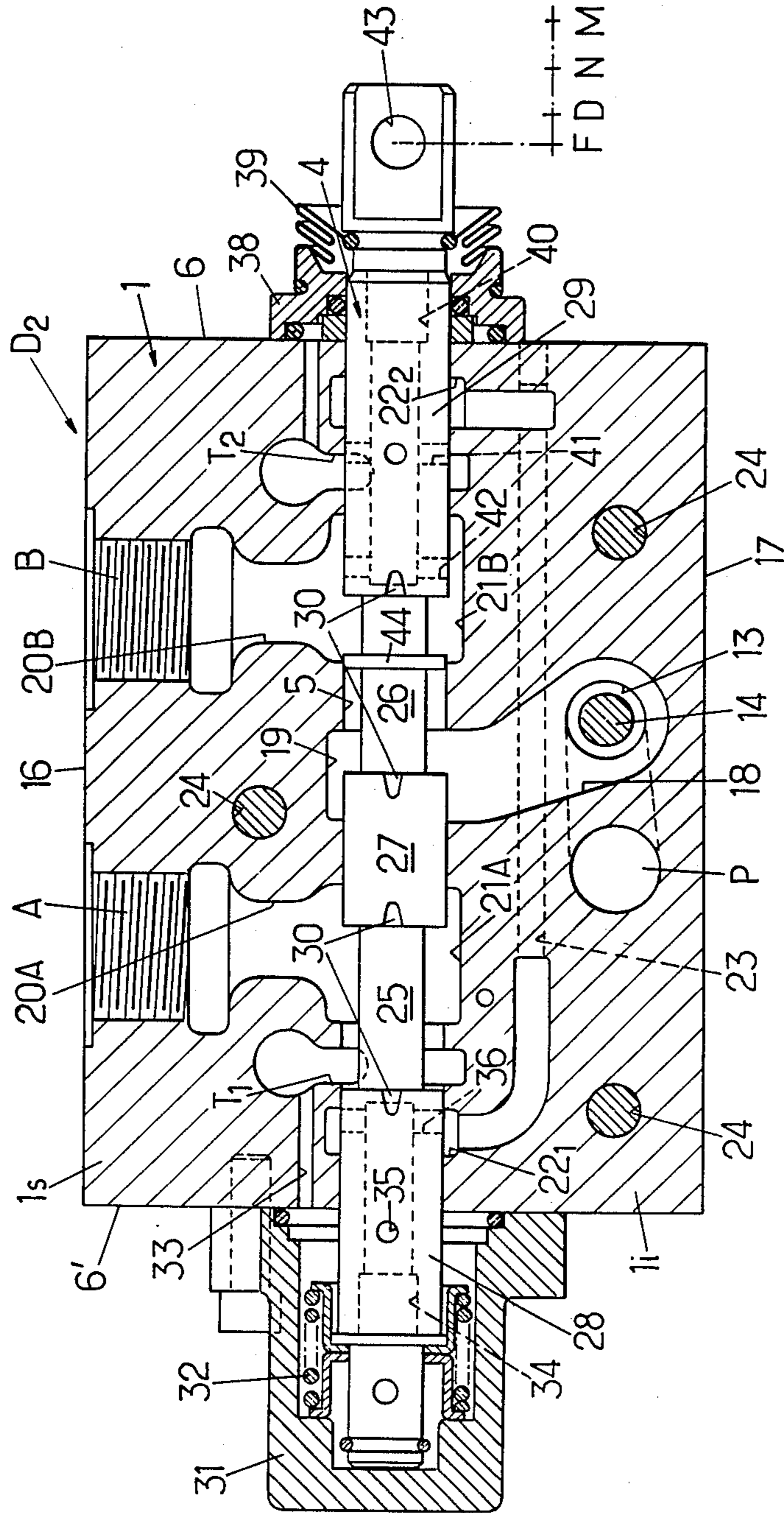
FIG. 6.
