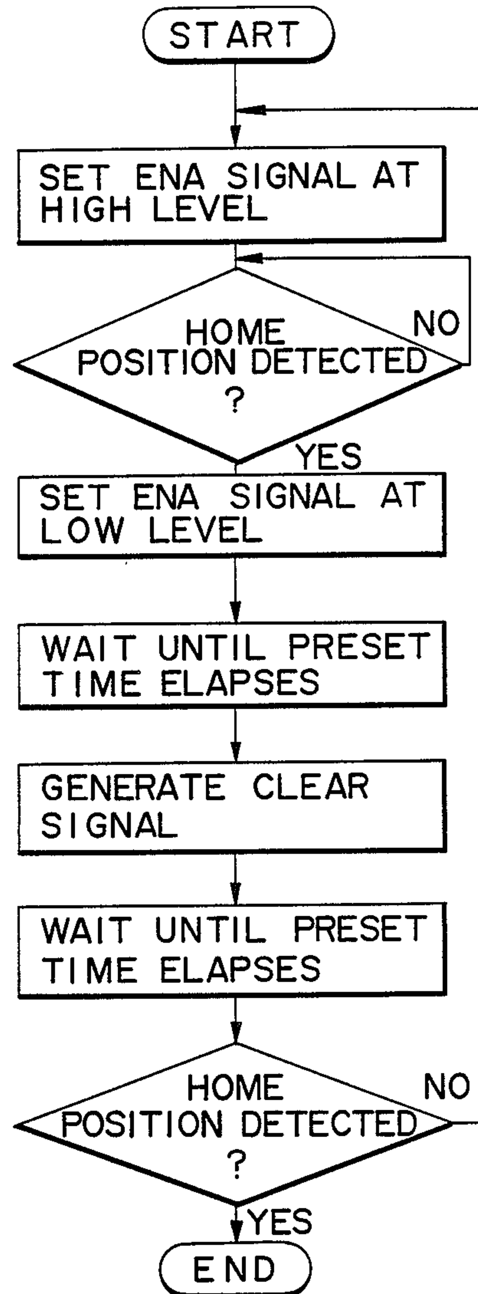
FIG. 9
