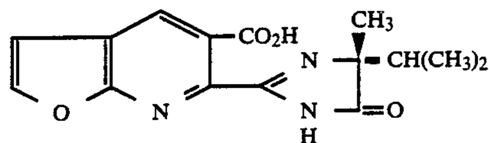
(+) - isomer
