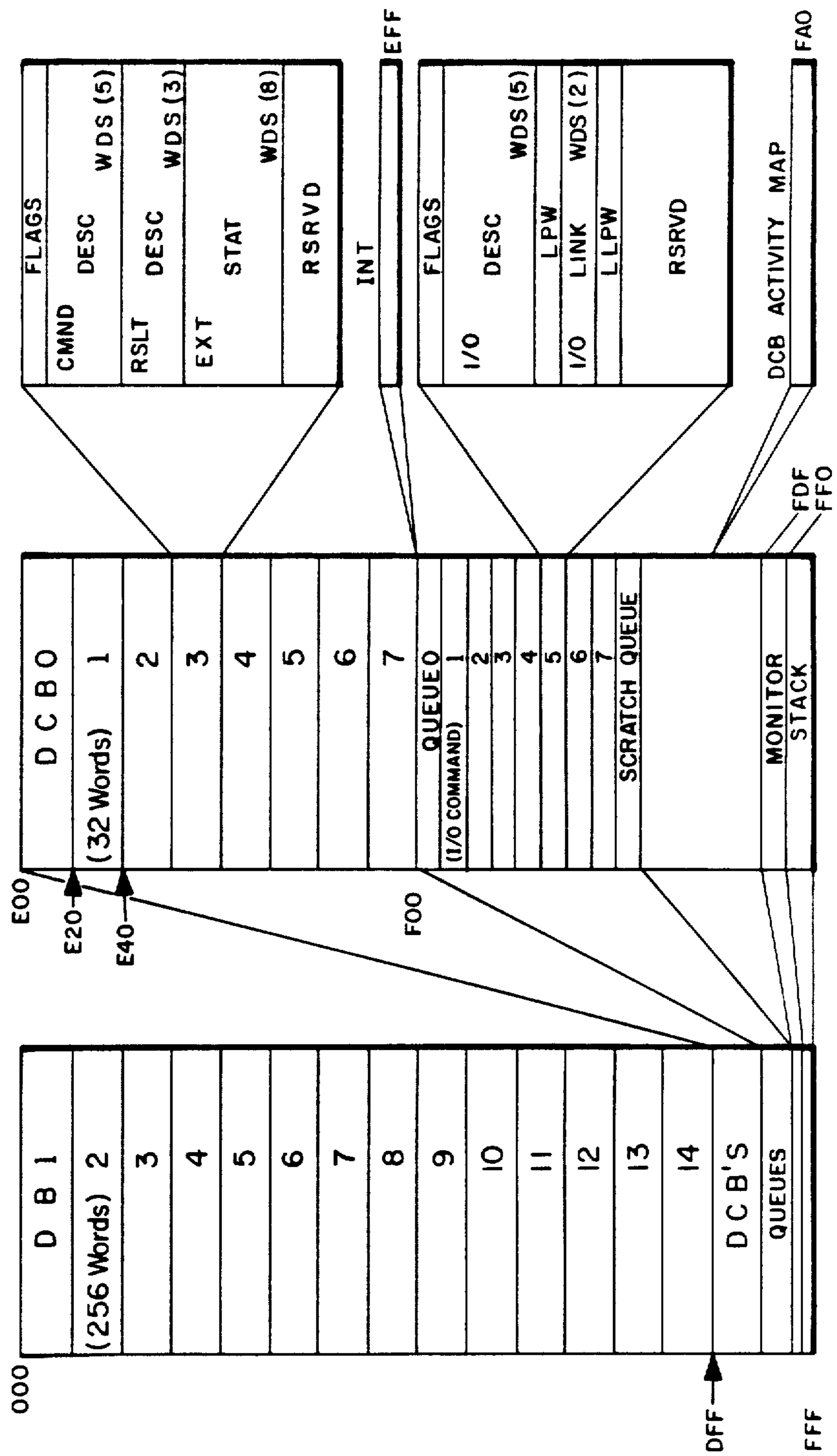
FIG. 6. SMD HA Memory Map (22, of Fig. 2.)
