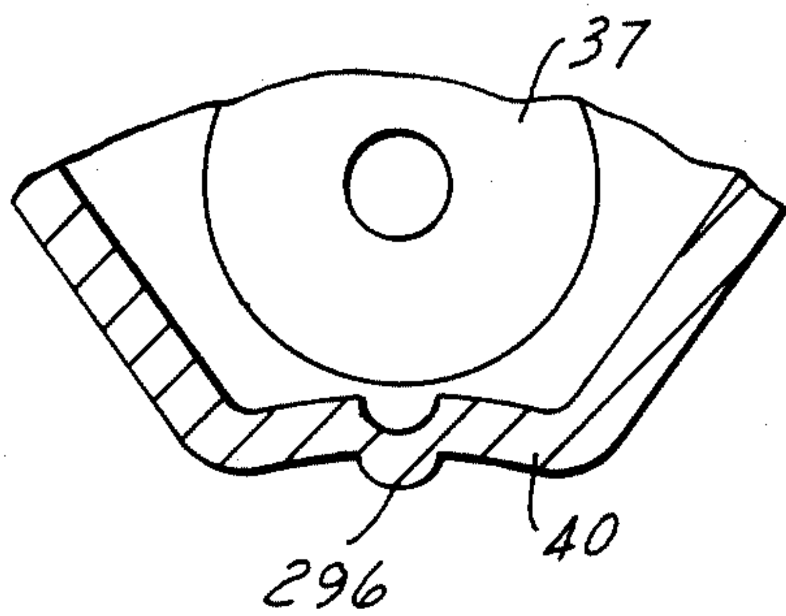
FIG. 19
