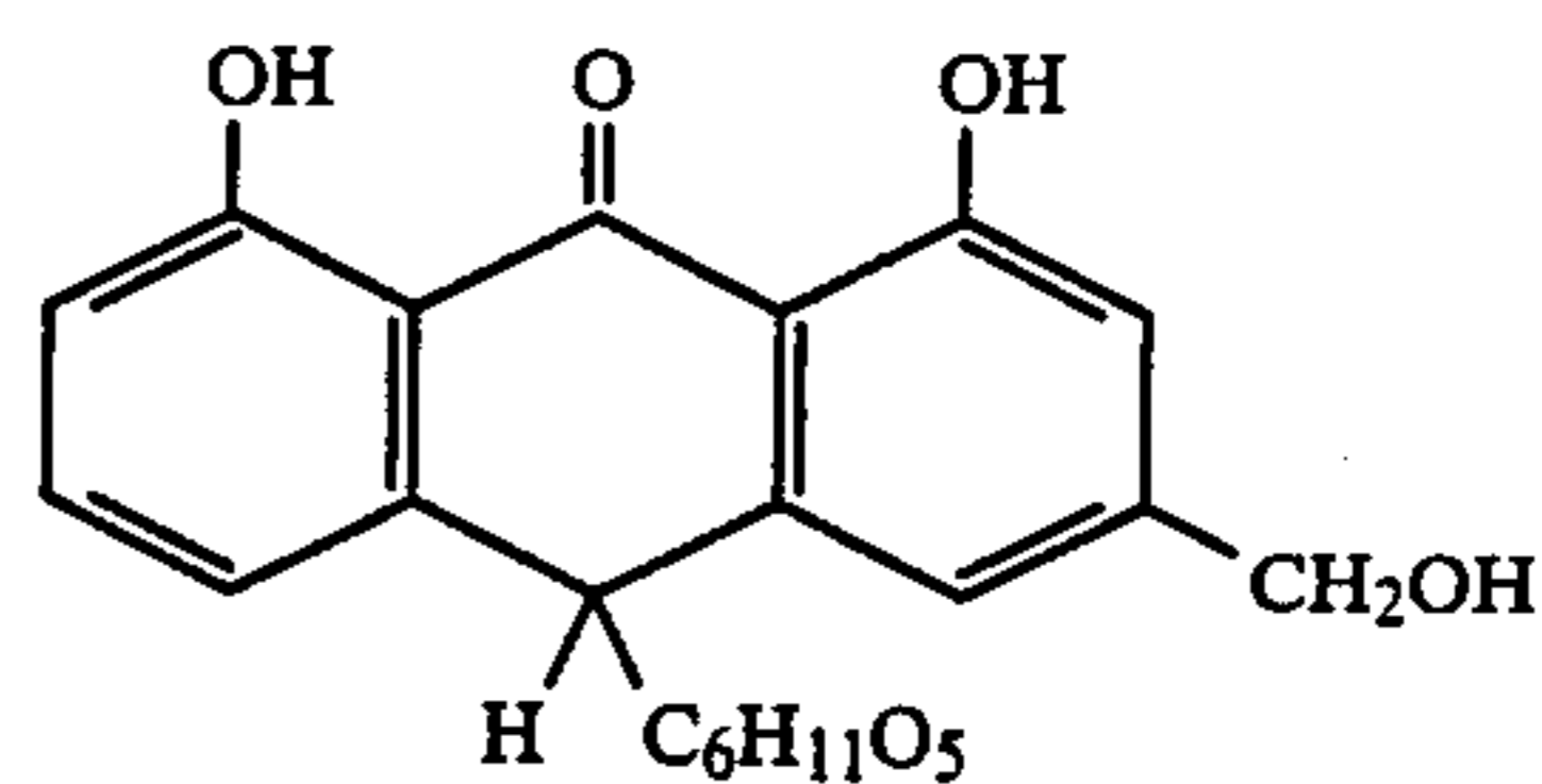
(±) Barbaloin
