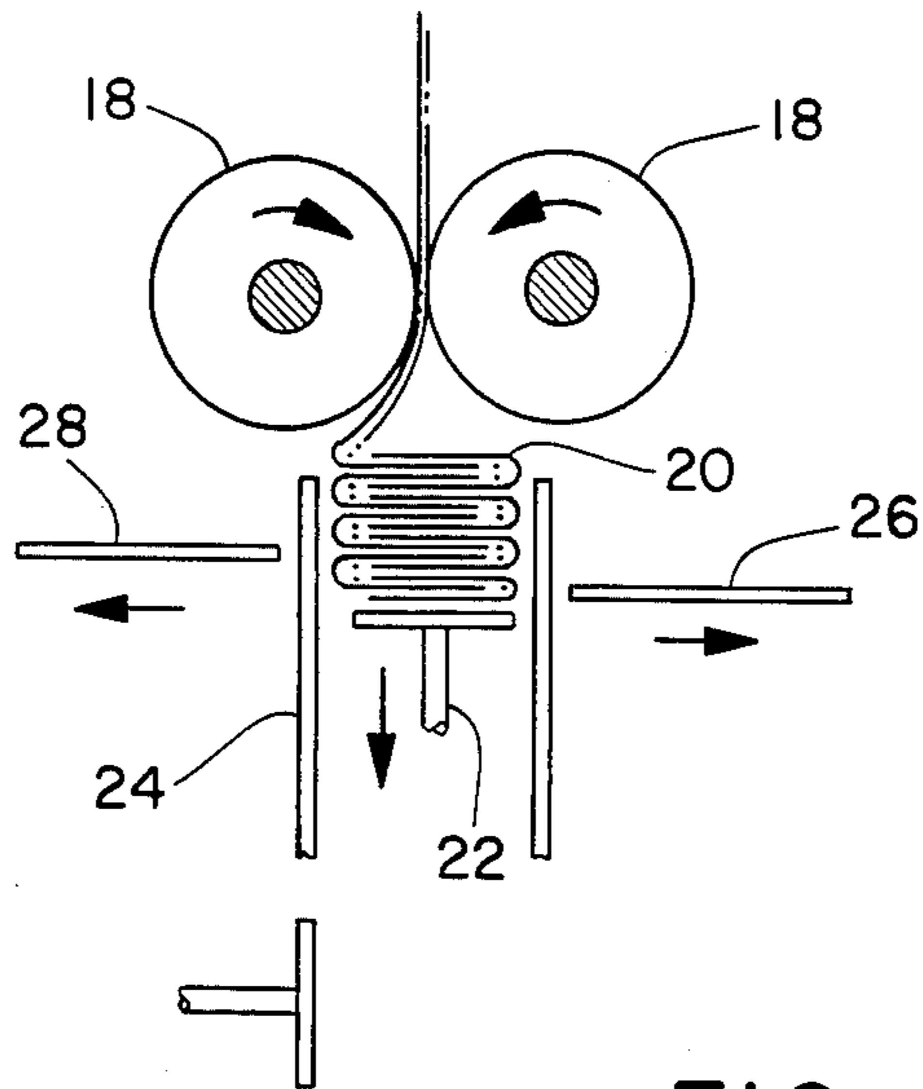
FIG. 10
