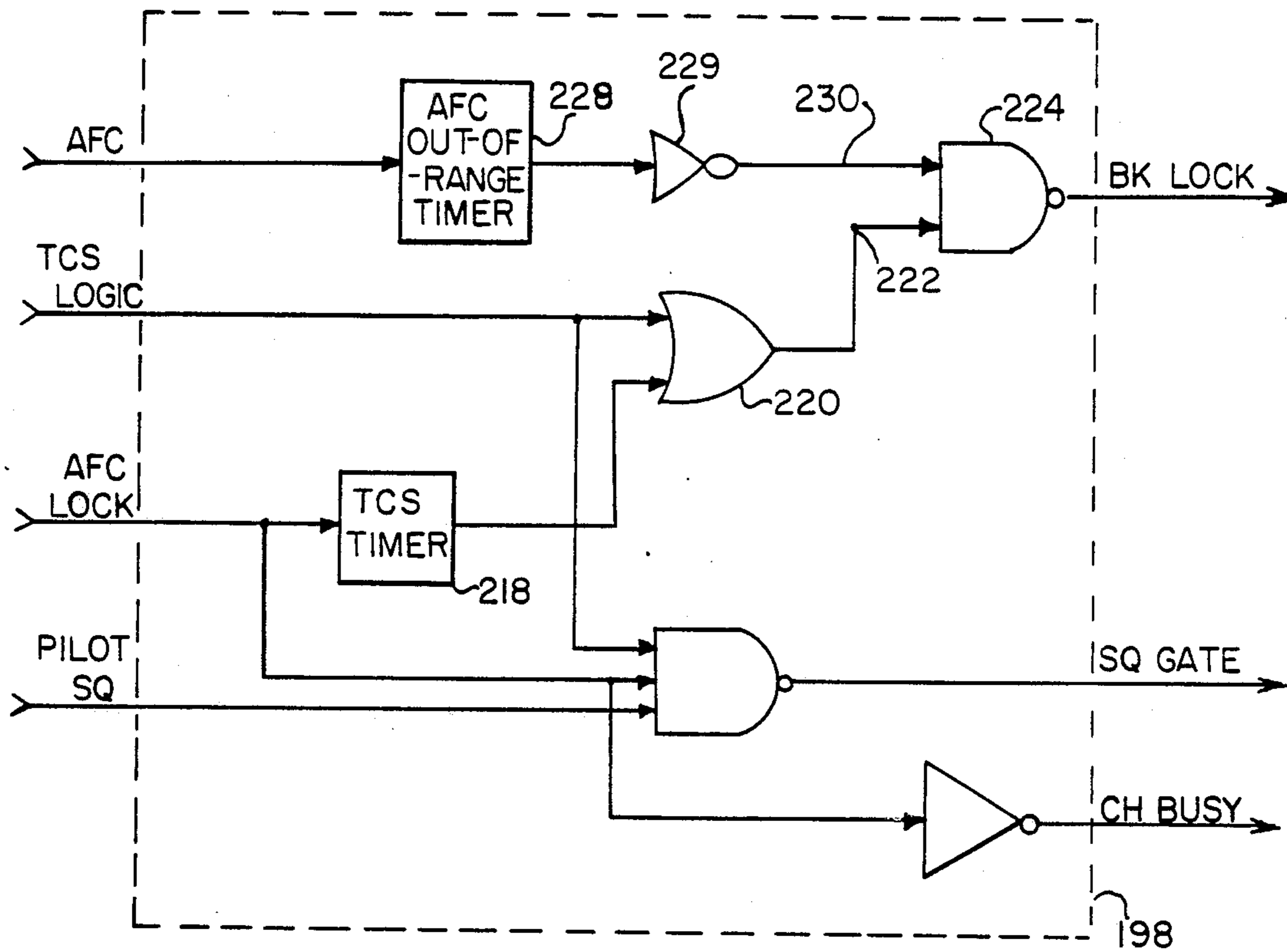
FIG. 5 LOGIC
