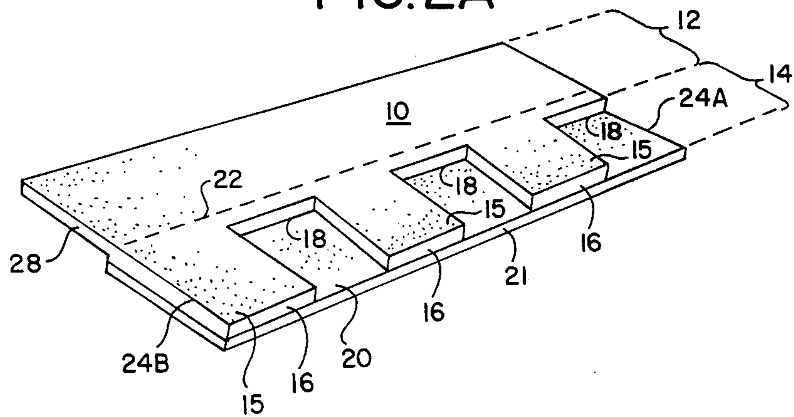
FIG. 2A
