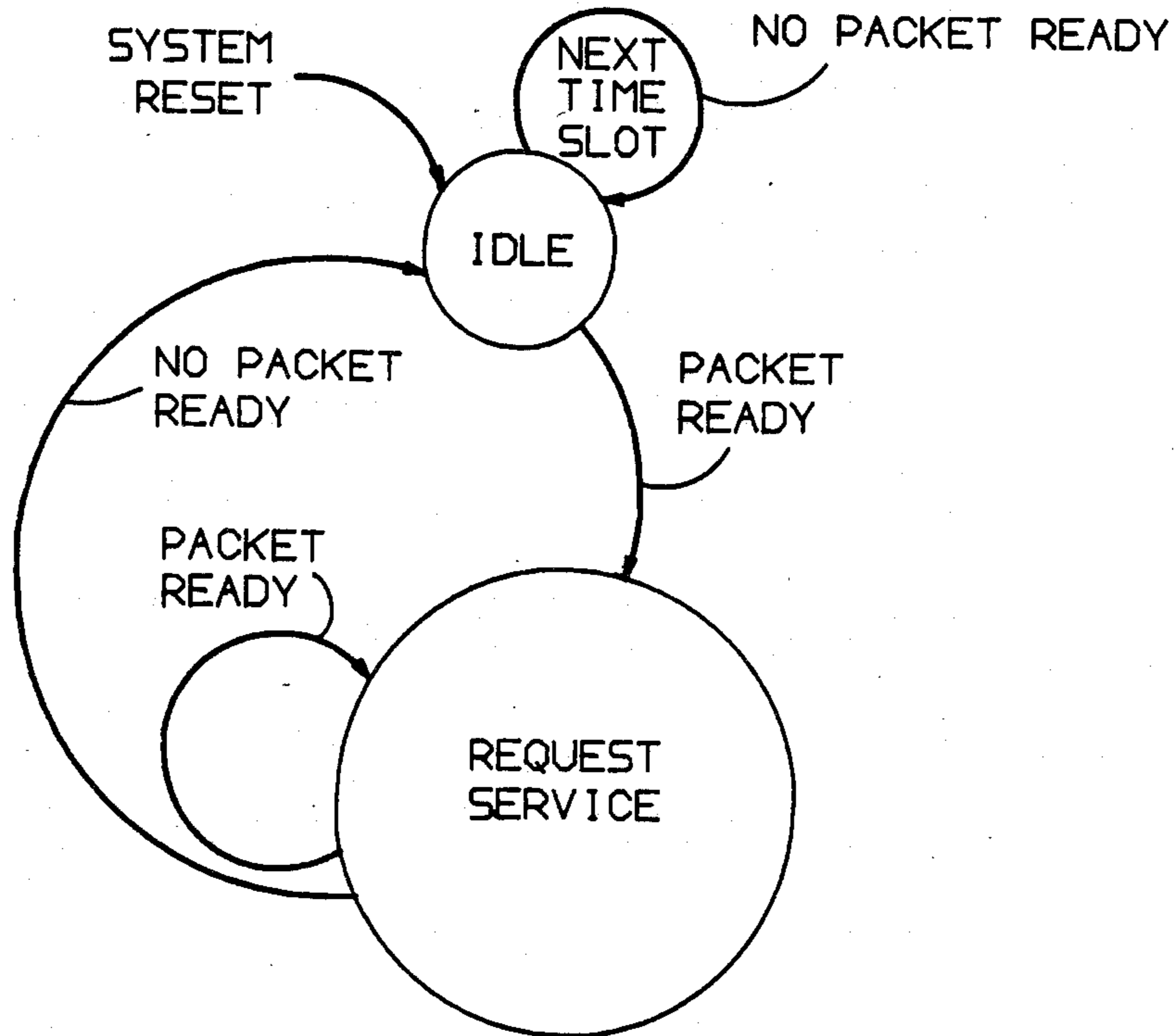
INPUT CONTROLLER 801
