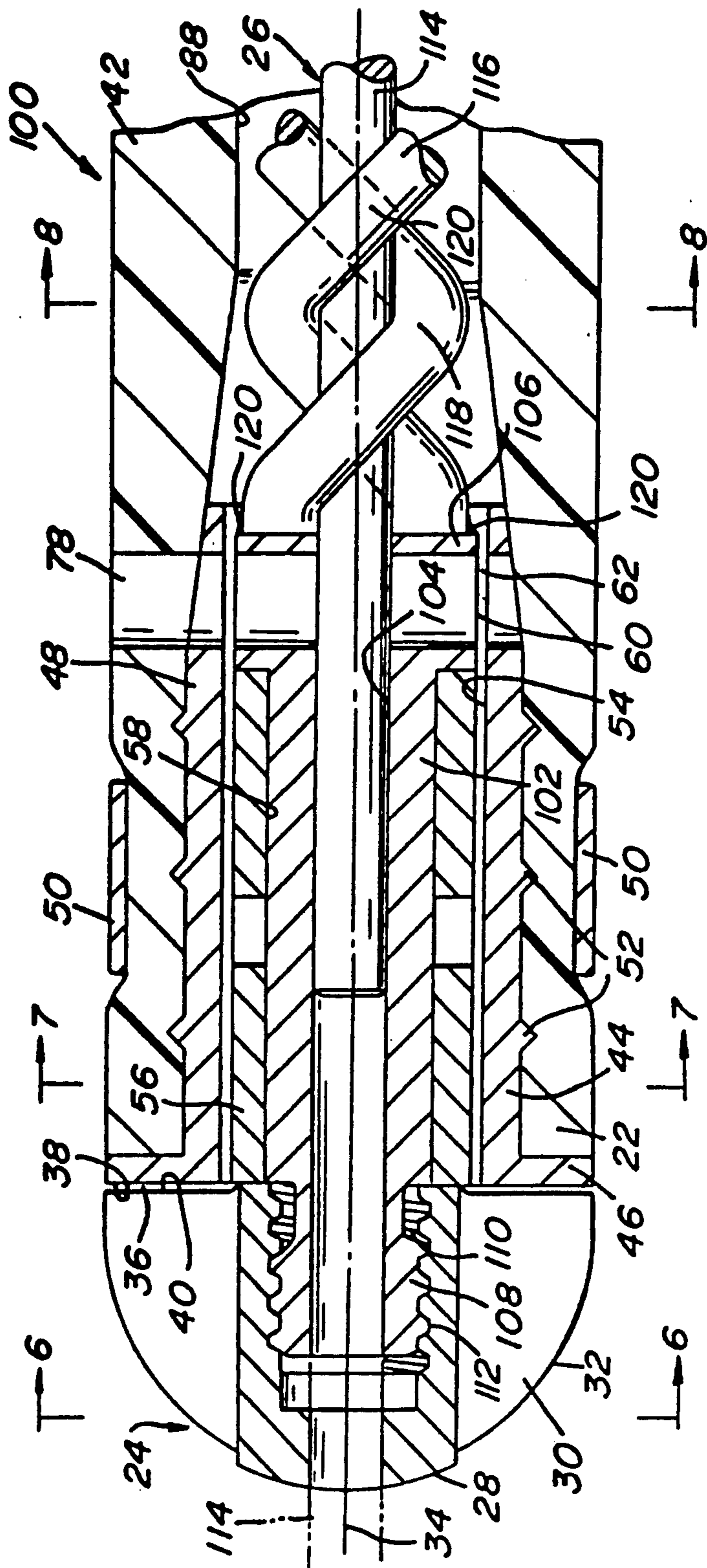
FIG. 5
