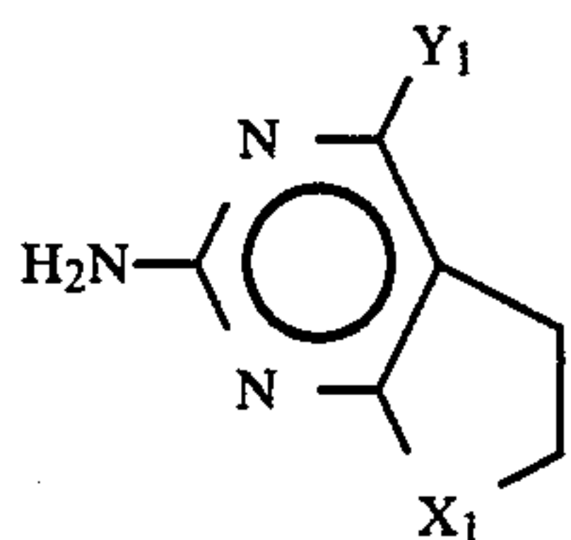
IIIb
