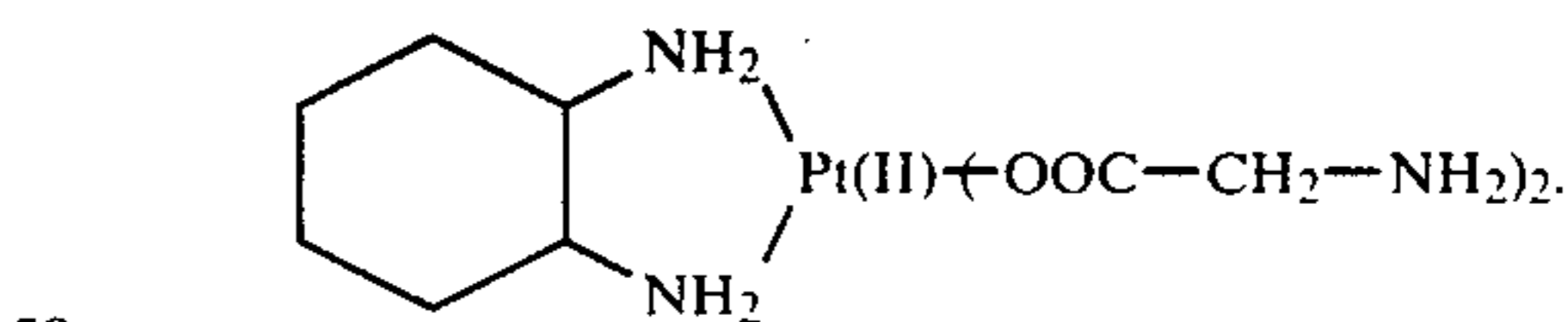
(bis-glycinato)
