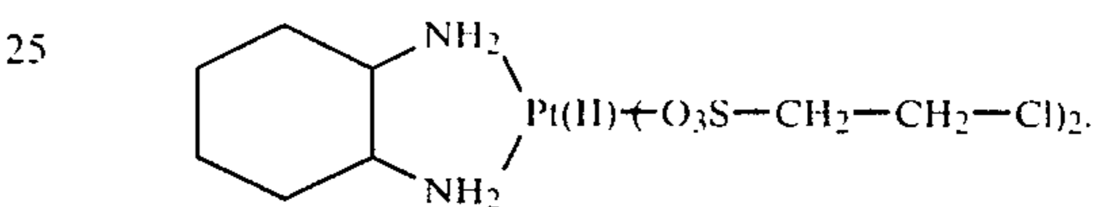
(bis-2-chloroethanesulfonato)
