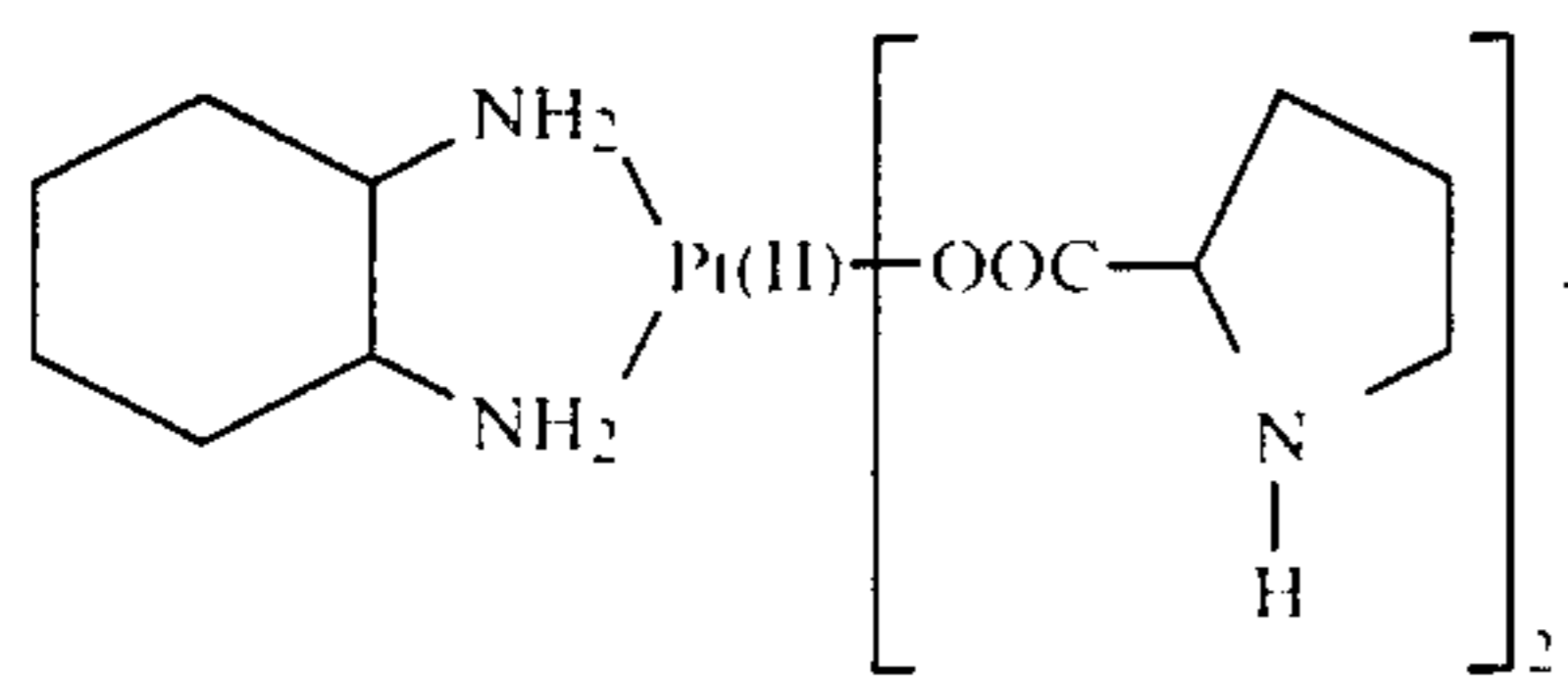
[bis-prolinato]
