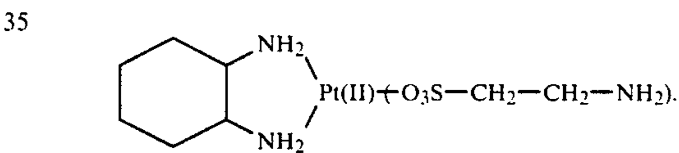
(bis-2-aminoethanesulfonato)
