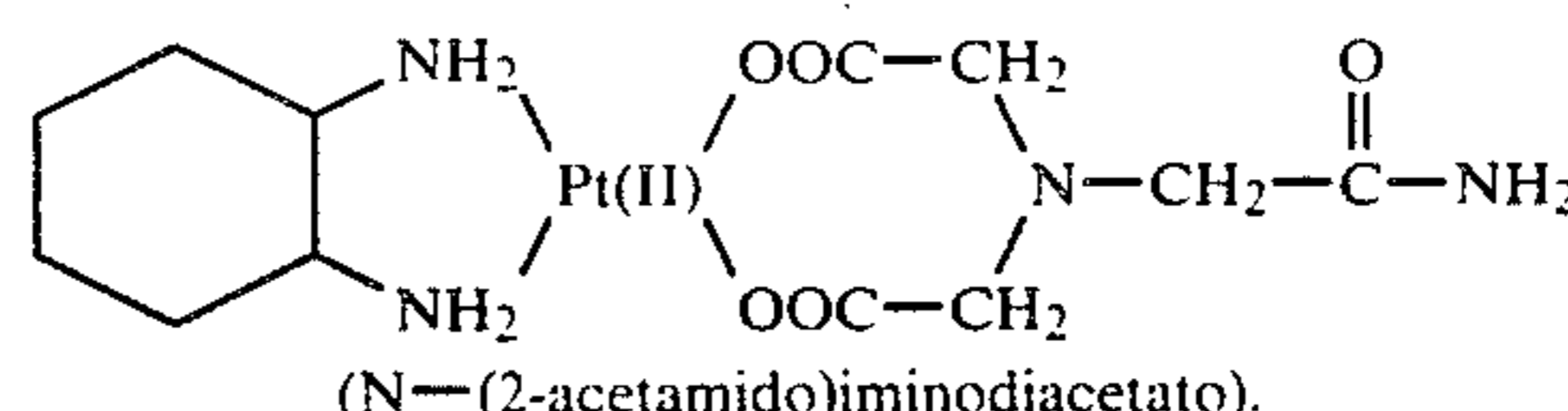
(N-(2-acetamido)iminodiacetato)
