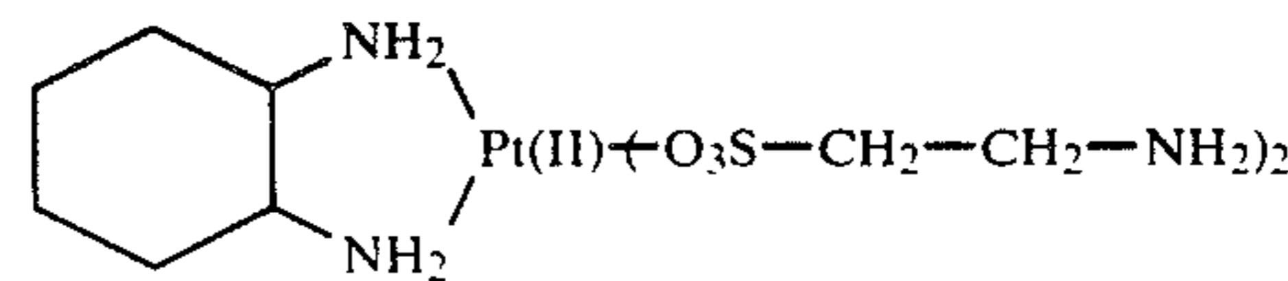
(bis-2-aminoethanesulfonato)
