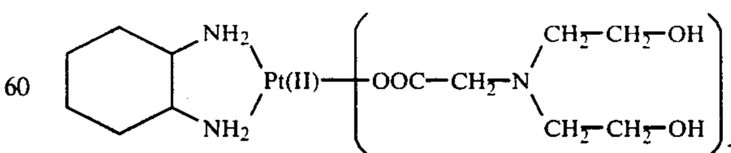
(bis-bicinato)
