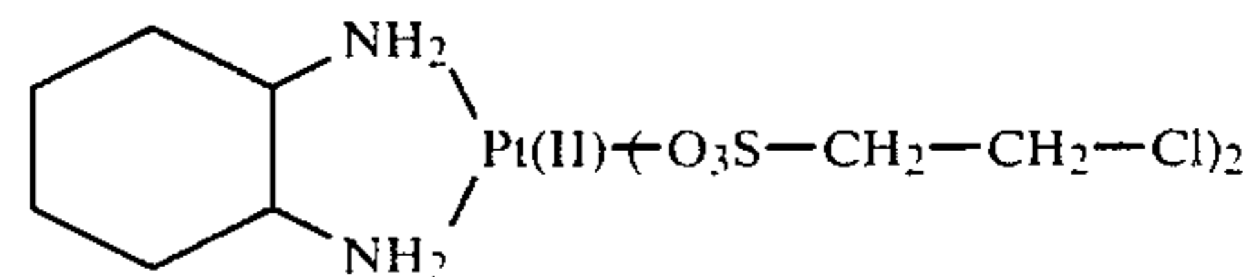
(bis-2-chloroethanesulfonato)
