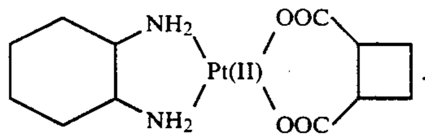
(trans-1,2-cyclobutanedicarboxylato)
