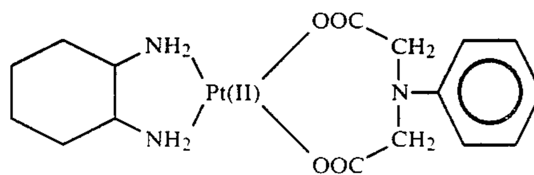
(N-phenyliminodiacetato)
